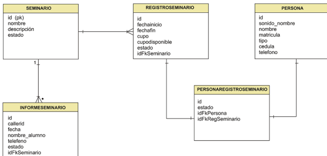
Figura 4.2: Modelo lógico de la base de datos seminario
