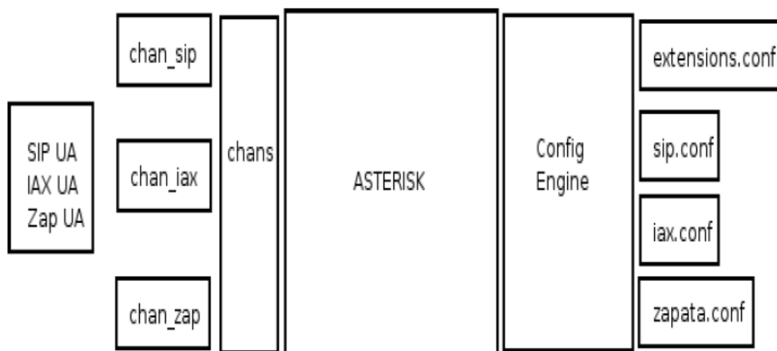
Figura 2.2. Arquitectura de archivos de configuración [8]
