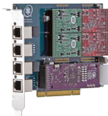
Figura 3.4: Tarjeta analógica modelo TDM410P [13]
