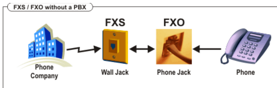
Figura 3.5: Conexión entre los puertos FXO y FXS [14]
