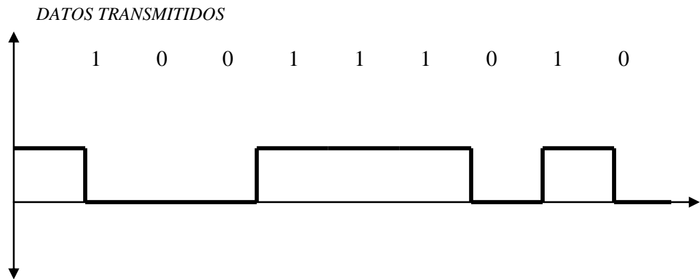
FIG. 2.30 MODULACIÓN ASK
