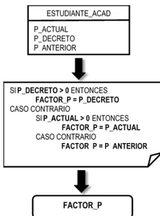
Figura 4.3. Pre-procesamiento de la variable Factor Socioeconómico
