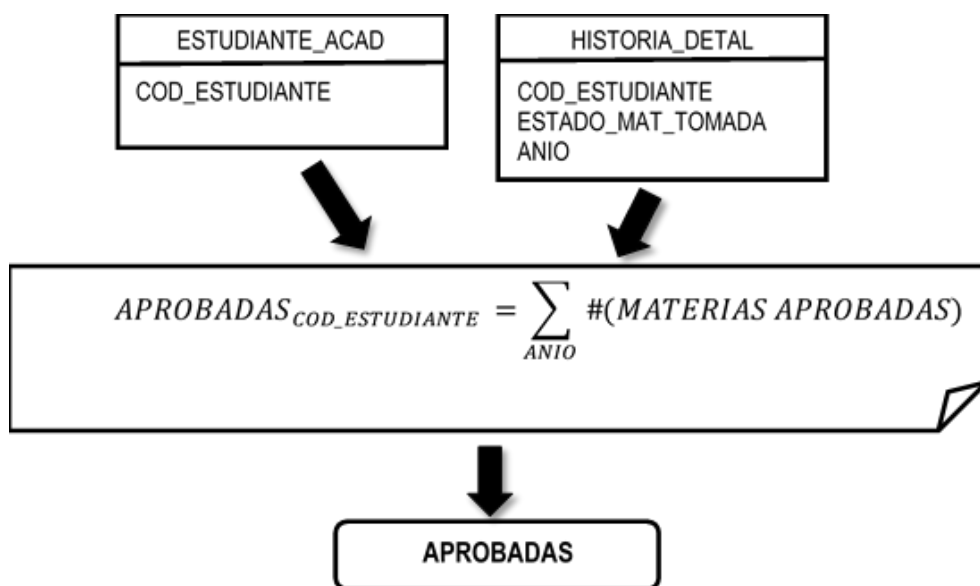
Figura 4.5. Pre-procesamiento de la variable Número de materias Aprobadas
