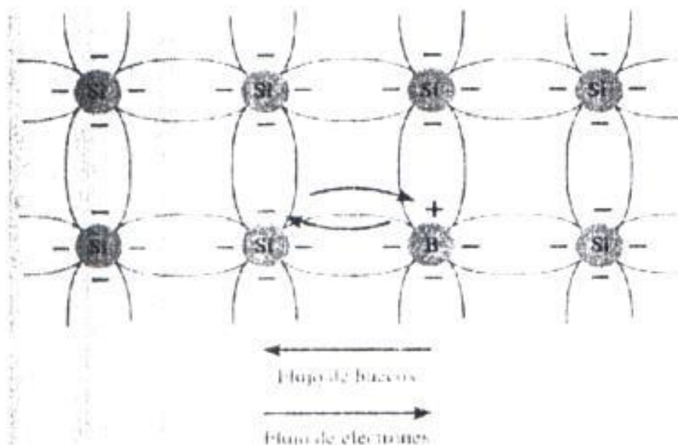
Figura 1.7: FLUJO DE ELECTRONES EN FUNCION DE FLUJO DE HUECOS (tomado del libro Circuitos Electrónicos de Boylestad)
