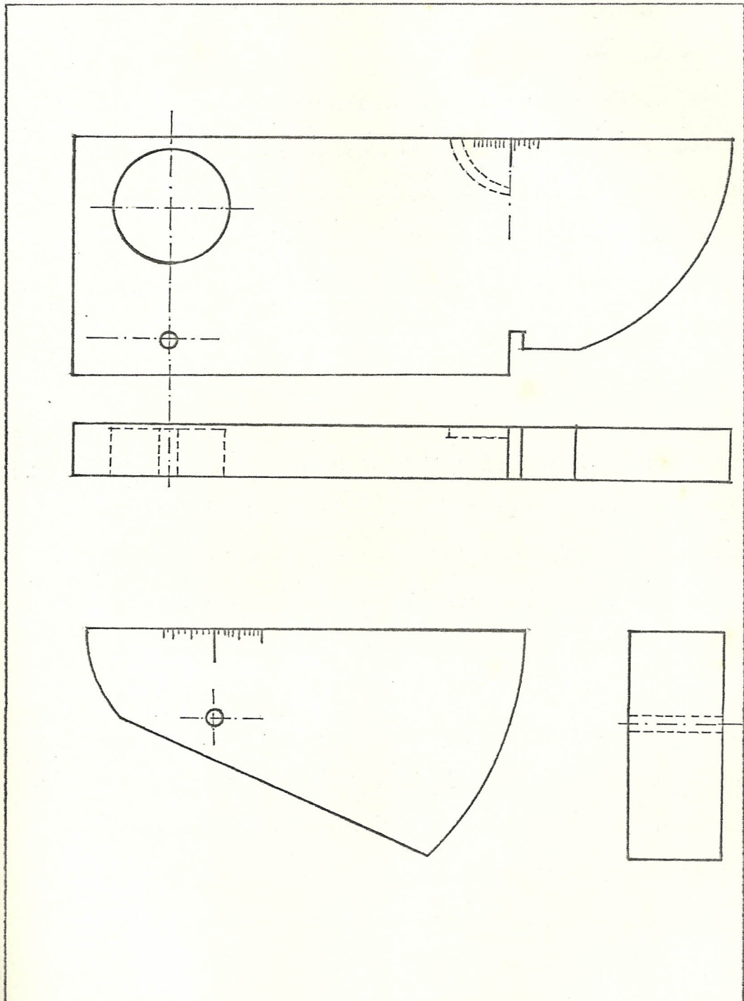
Fig. No. 30 BLOQUES DE CALIBRACION a) IIW o V1 b) V2
