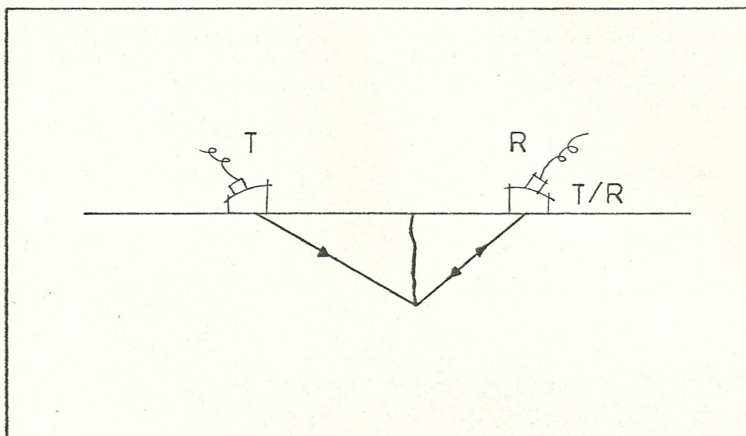
Fig.Nº24 Localización de una fisura usando los transductores como transmisor-receptor y uno de ellos como transmisor-receptor simultáneamente. (Ref.5)
