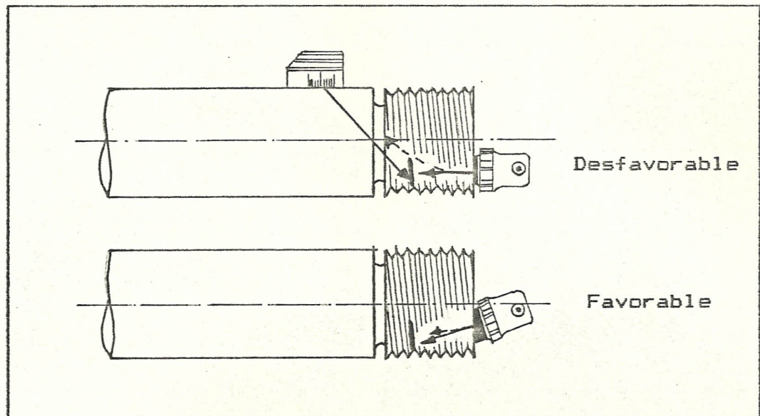
Fig.Nº11 Emisión inclinada del haz mediante transductor normal en ejes roscados para detectar fisuras en su inicio, partiendo del fondo de la rosca. (Ref.4)
