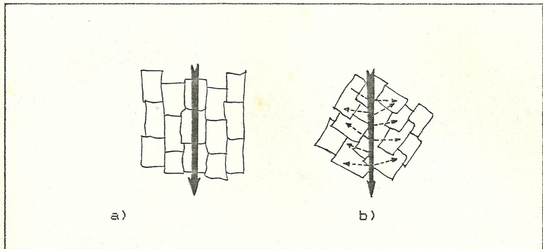
Fig.Nº20 a) En los materiales elásticamente anisotropo existe buen paso del haz ultrasónico por la orientación de los cristales. b) Fuerte dispersión de los ultrasónicos al hallarse los cristales dispuestos en forma irregular. (Ref.4)
