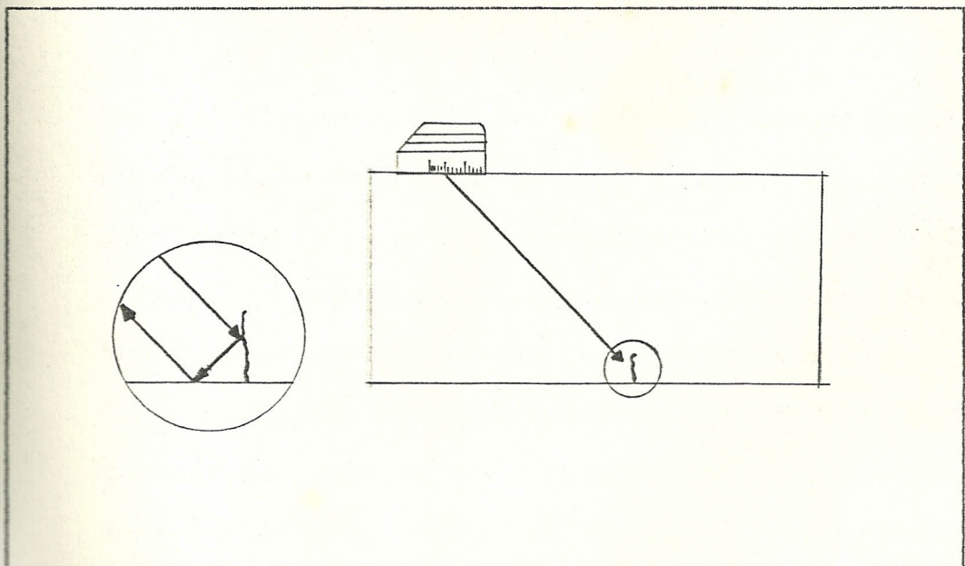
Fig.Nº10 Emisión inclinada del haz aprovechando el efecto de espejo angular de la fisura (Ref.4)
