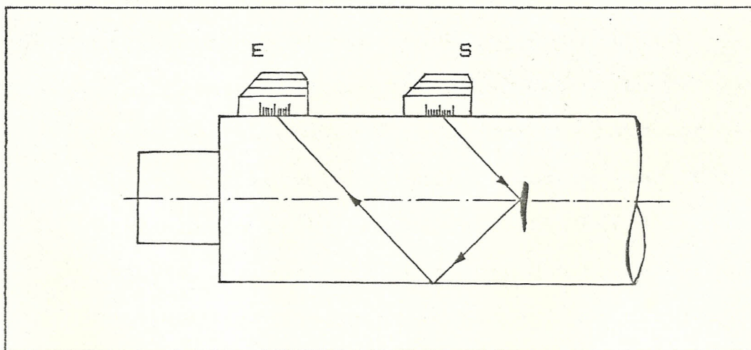
Fig.Nº14 Detección segura de una fisura utilizando el sistema Tandem (método de 2 palpadores). (Ref.4).
