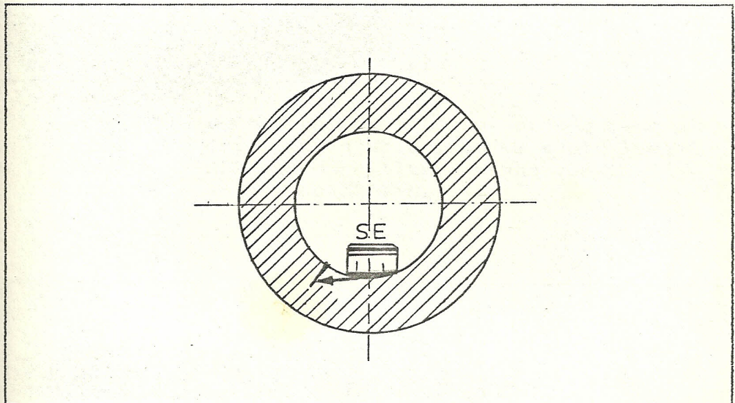
Fig.Nº17 Detección de fisuras radiales situadas en el orificio interior por medio de transductores angulares SE. (Ref.4)
