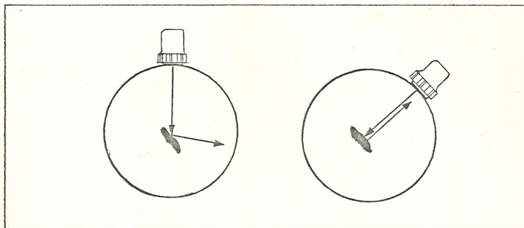
Fig. N07 Detección de discontinuidades planas mediante emisión perpendicular del haz ultrasónico. (Ref.4).
