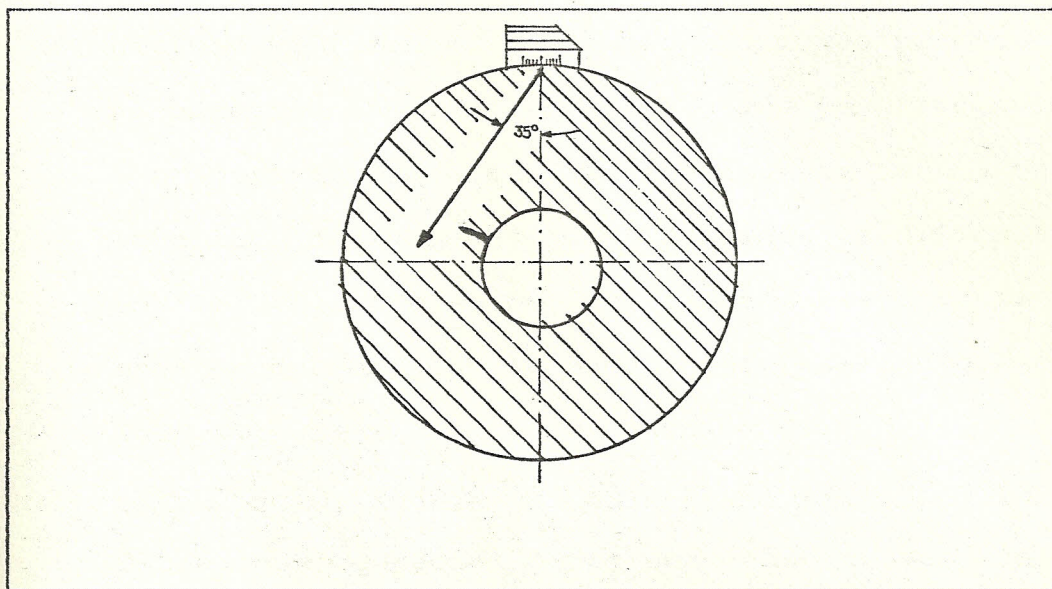
Fig.Nº18 Detección de fisuras sin acceso al orificio interior, no se suele llegar a la zona crítica incluso con un ángulo de 35°. (Ref.4)
