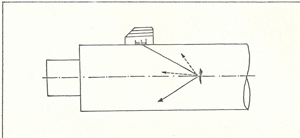
Fig.Nº13 Detección, con emisión inclinada mediante un solo transductor angular de la superficie irregular de la fisura. (Ref.4)
