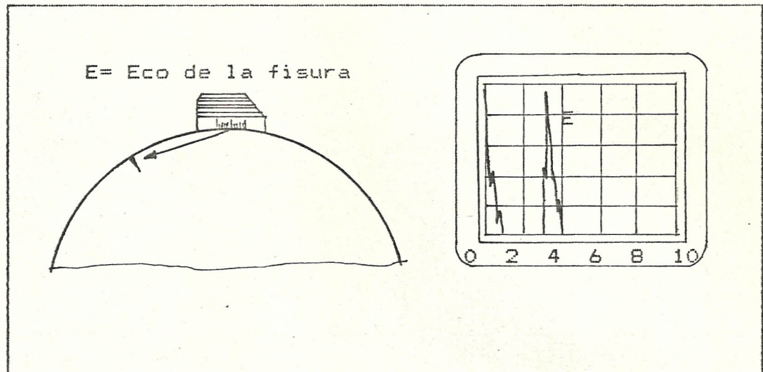
Fig.Nº15 Buena detectabilidad de fisuras longitudinales superficiales por la curvatura superficial. (Ref.4)
