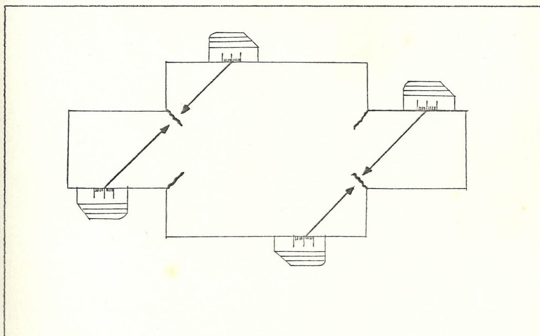
Fig.N08 Verificación de las zonas expuestas a fisuras, teniendo en cuenta su dirección preferente. (Ref.4)
