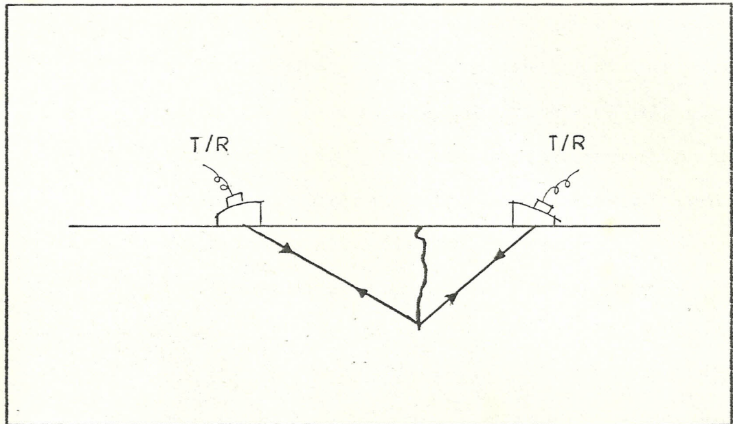
Fig.Nº22 Localización de una fisura usando los transductores como transmisor-receptor simultáneamente. (Ref.5)
