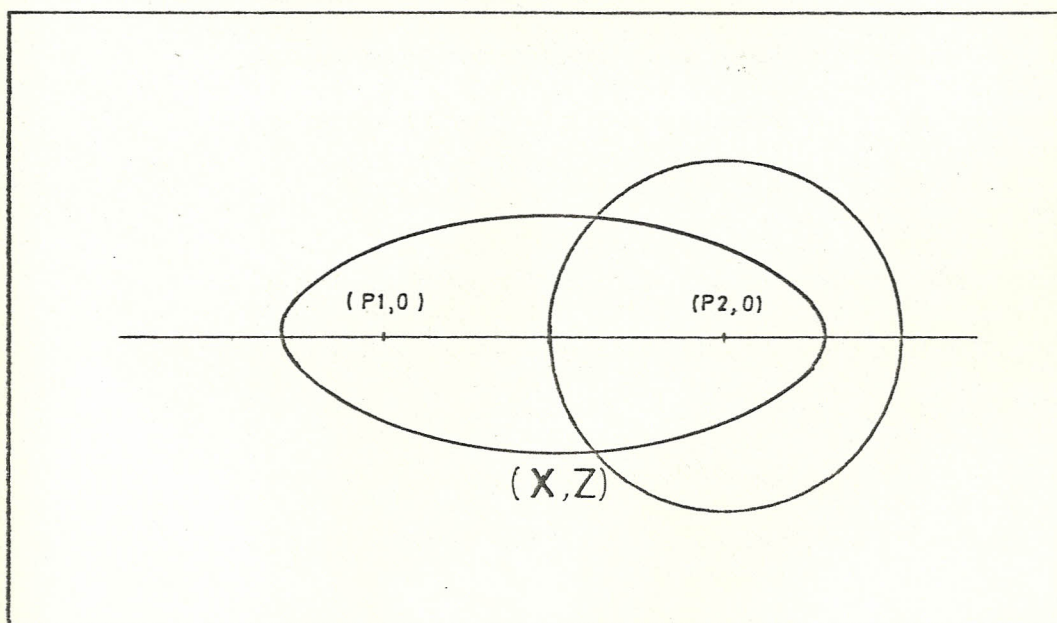
Fig.Nº25 La localización de la fisura (x,z) es dada por el punto de intersección de la elipse y el círculo dentro del material. (Ref.5)
