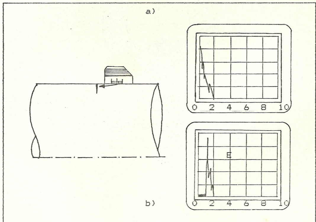
Fig.Nº16 a) Poder resolutivo insuficiente en el campo cercano de la fisura. b) Excelente poder resolutivo en el campo cercano del transductor angular SE. (Ref.4).
