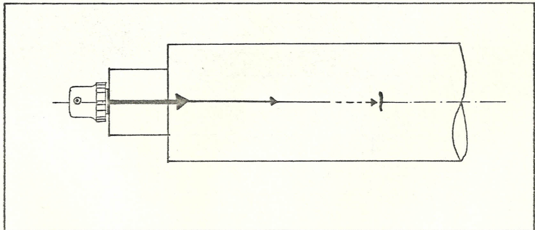
Fig.Nº12 Detección de fisuras utilizando transductor normal a lo largo del eje de una pieza alargada. (Ref.4)
