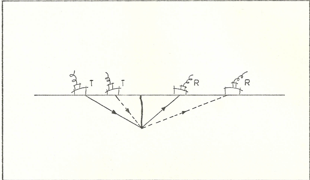
Fig.Nº26 Localización de una fisura colocando los transductores en dos posiciones y usando ellos como transmisor-receptor (Ref.5)
