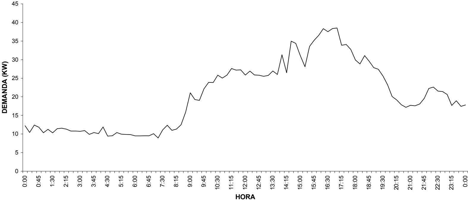
CURVA DE CARGA TIPO COMERCIAL
