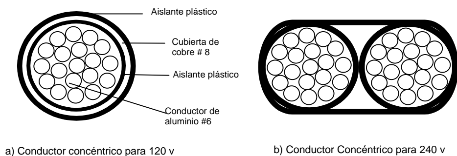
FIGURA 4.4. CONDUCTOR ANTIHURTO
