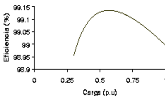
FIGURA 4.7. EFICIENCIA TÍPICA DE LOS TRANSFORMADORES DE DISTRIBUCIÓN
