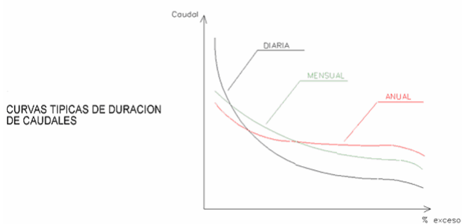
GRAFICO III CURVA DE CUADALES MEDIOS
