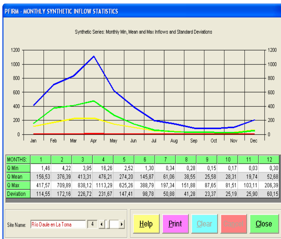
GRAFICO XXXVIII CAUDALES SINTETICOS PROYECTO BABA
