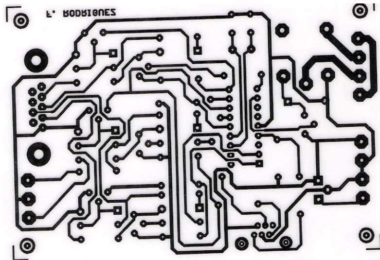
Figura 2.4. Circuito impreso del circuito de interfase entre el lector ACR30 y la tarjeta SBC45EC
