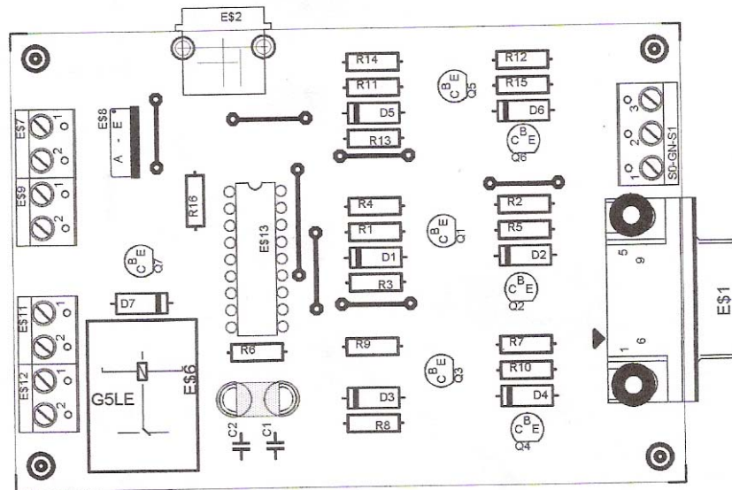
Figura 2.5. Componentes en la placa del circuito de interfase entre el lector ACR30 y la tarjeta SBC45EC
