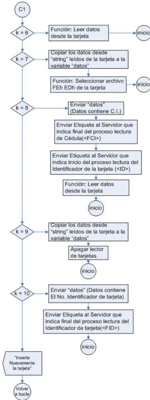
Figura 2.7. Diagrama de flujo de la función implementada en el Microcontrolador 2
