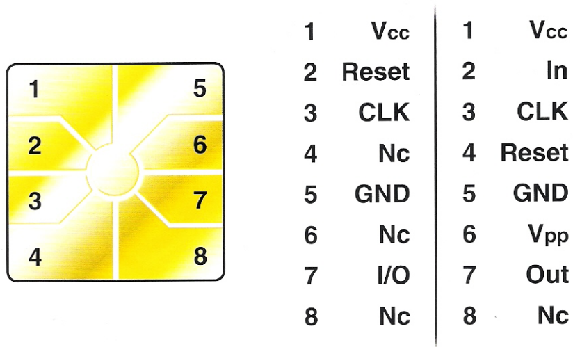
Figura 3.3. Definición de contactos de acuerdo al estándar ISO 7816 – 2.
