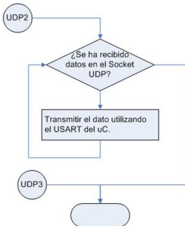
Figura 2.8. Diagrama de Flujo de la función implementada en el Microcontrolador 1 .
