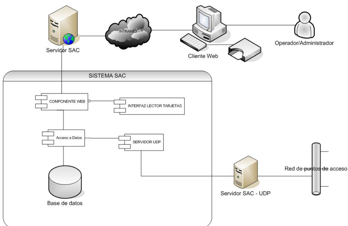
Figura 7.2 – Arquitectura del sistema SAC
