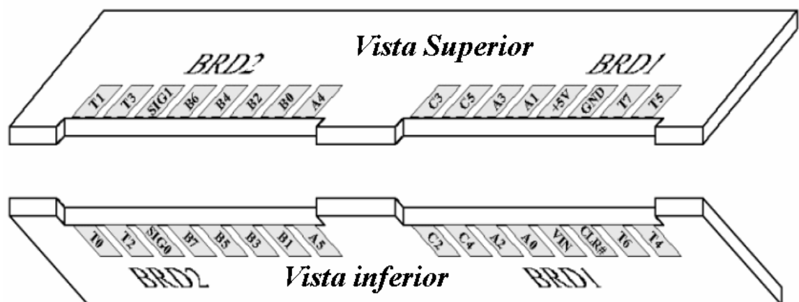
Figura 6.4. Conector frontal de la tarjeta SBC45EC
