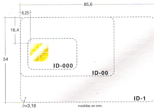
Figura 3.2. Tipos de tarjetas según el formato
