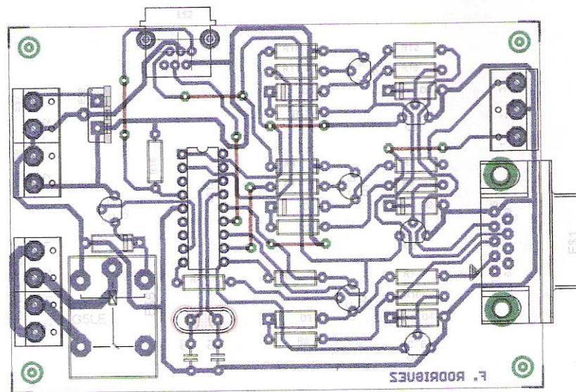
Figura 2.6. Gráfico de la ubicación de los componentes en el circuito de interfase entre el lector ACR30 y la tarjeta SBC45EC y su conexión.
