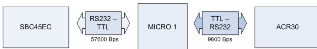
Figura 2.2 Diagrama de bloques del circuito de interfase entre el lector ACR30 y la tarjeta SBC45EC.
