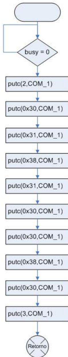
poweroff()
