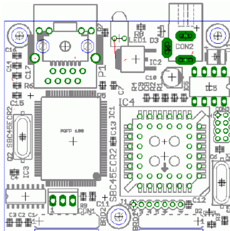
Figura 6.7. Layout de la tarjeta madre SBC45EC usada en el desarrollo del proyecto.
