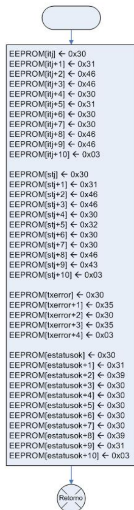
ComandosRespuestaEEprom()
