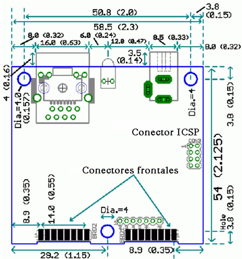
Figura 6.6. Dimensiones de la tarjeta SBC45EC.
