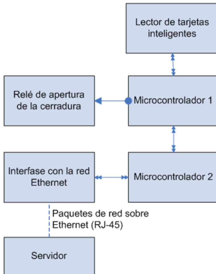
Figura 2.1. Diagrama de Bloques General del Proyecto.
