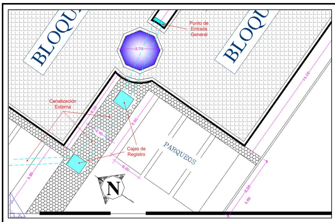
Figura 4-117.- Recorrido Canalización Externa
