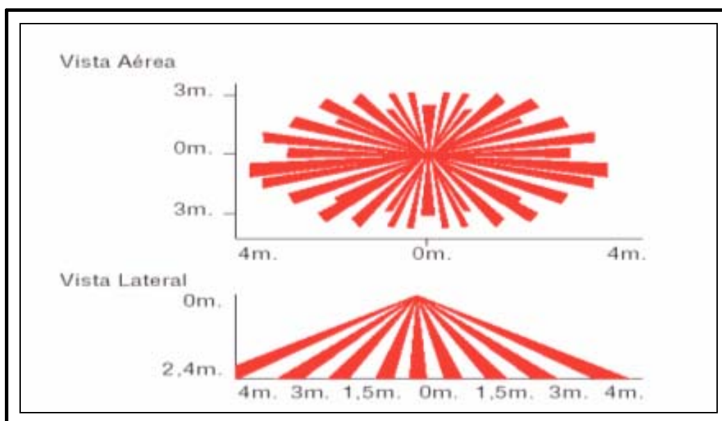
Figura 4-80.- Rango de cobertura detector infrarrojo de movimiento
