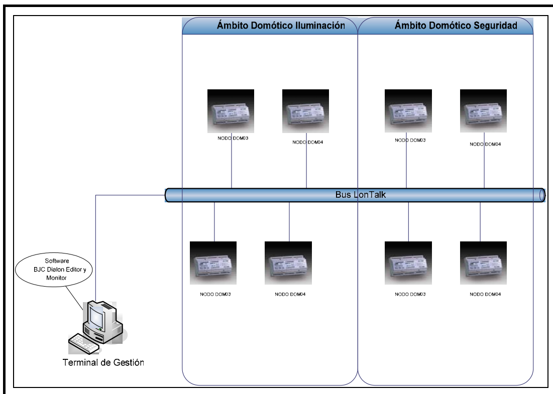
Figura 4-12.- Sistema de Gestión sobre el Bus LonTalk
