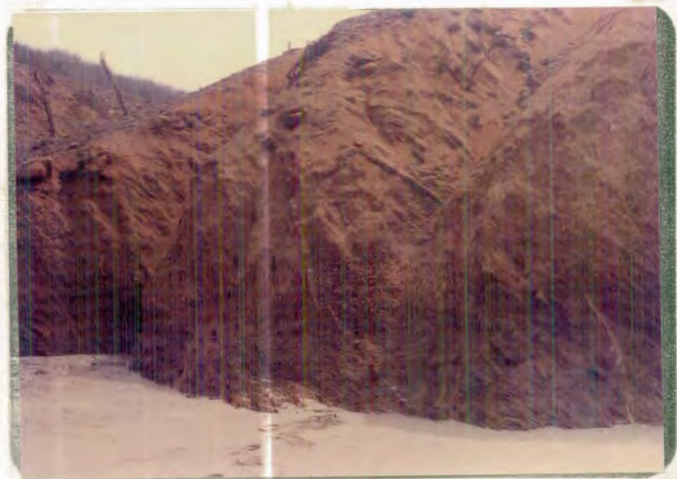
Fig. 61. Pliegue anticlinal, vuelto a plegar en el vértice (en dirección del martillo). Pto. 15a, vista al NO.
