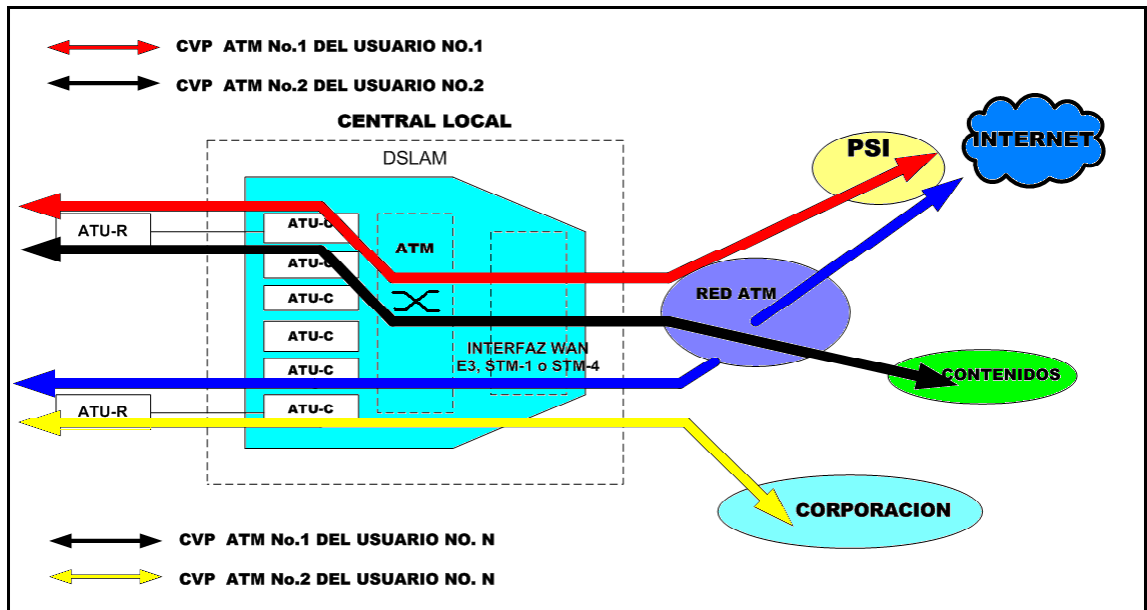
Figura 1.16 DSLAM ATM
