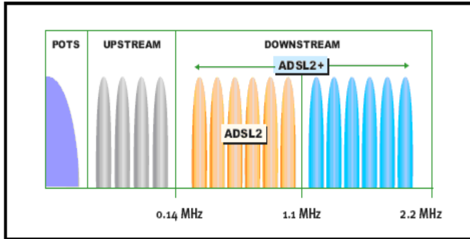
Figura 1.30 ADSL2+ dobla el ancho de banda de ADSL2
