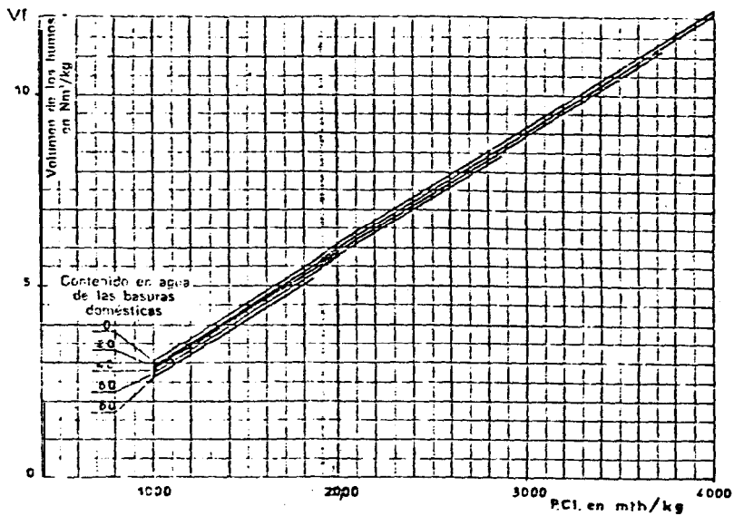
FIG. 11 Volúmenes de los humos en \text{Nm}^3 producidos por la combustión de 1 kg de basuras domésticas a la temperatura de 950\text{ }^\circ\text{C} , en función del PCI y del contenido en agua.
