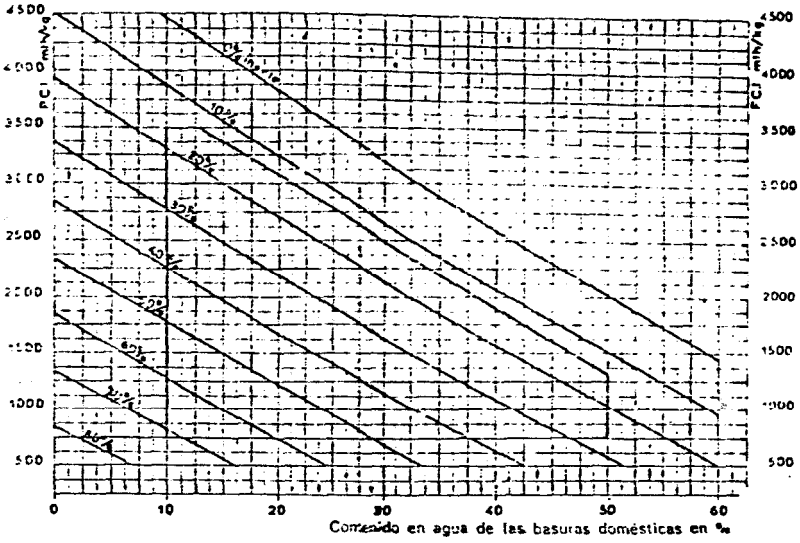
FIG. 8 Valor del PCI de las basuras domésticas en función del contenido en vertes y del contenido en agua, suponiendo que las materias combustibles son de domi- nante celulósico.
