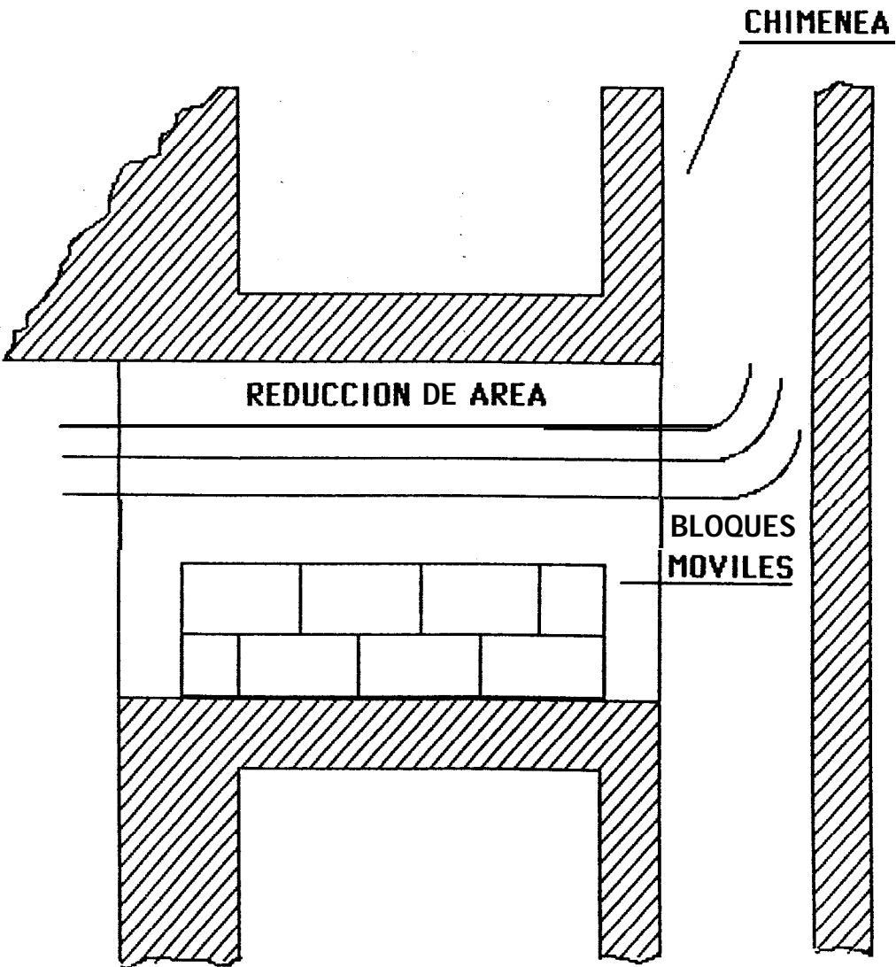
FIGURA Nº 18 REGULACION DEL TIRO
