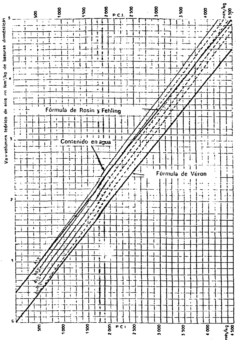
FIG. 10 Volumen teórico de aire para una combustión neutra (en Nm^3 por kilogramo de basuras) en función del PCI y del contenido en agua de las basuras domésticas.
