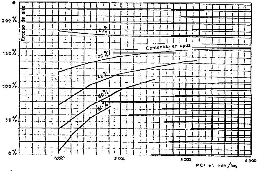
FIG. 9 Exceso de aire, en porcentaje del aire teórico, para una temperatura de 950°C en la cámara de combustión, en función del PCI y del contenido en agua de las basuras domésticas.
