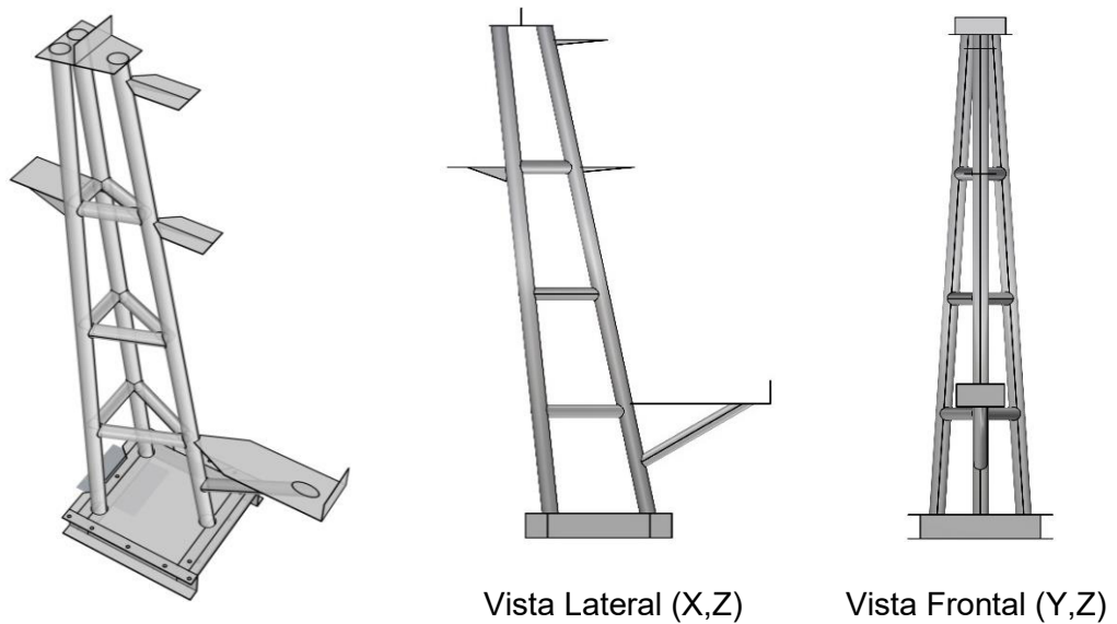
Figura 5. Modelo geométrico
