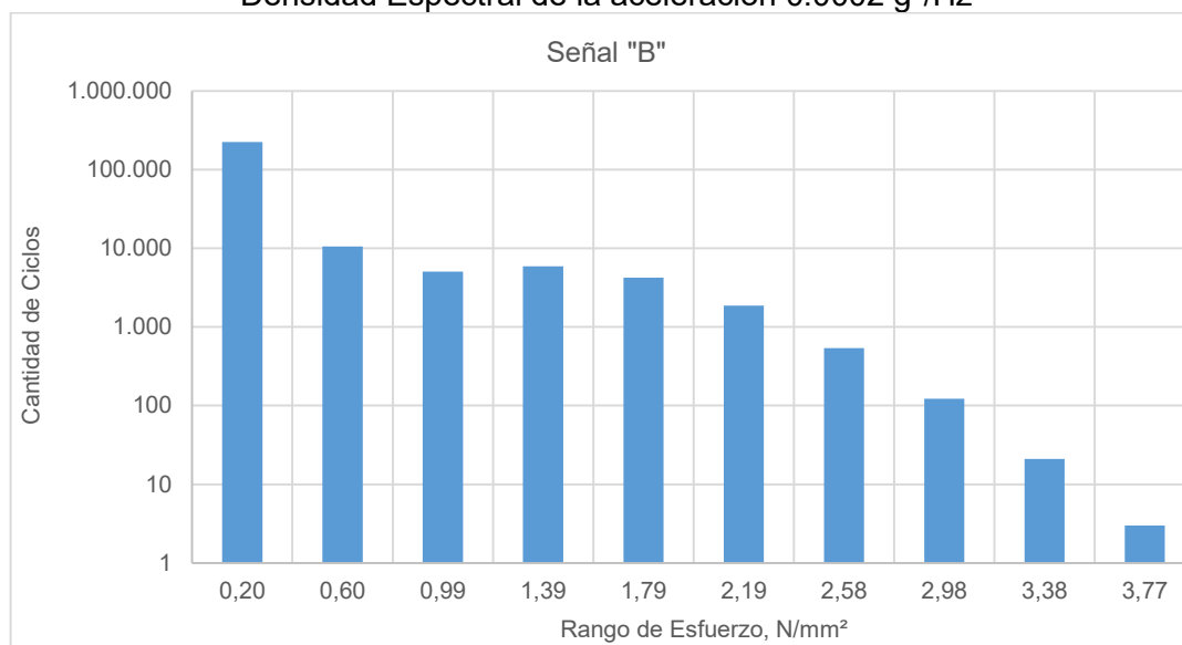
Figura 3.17: Cálculo de cantidad de ciclos para la señal "B", dirección "Y"
