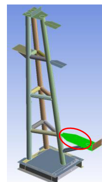
Figura 8. Asignación de espesor y propiedad del elemento “Parte 1”
