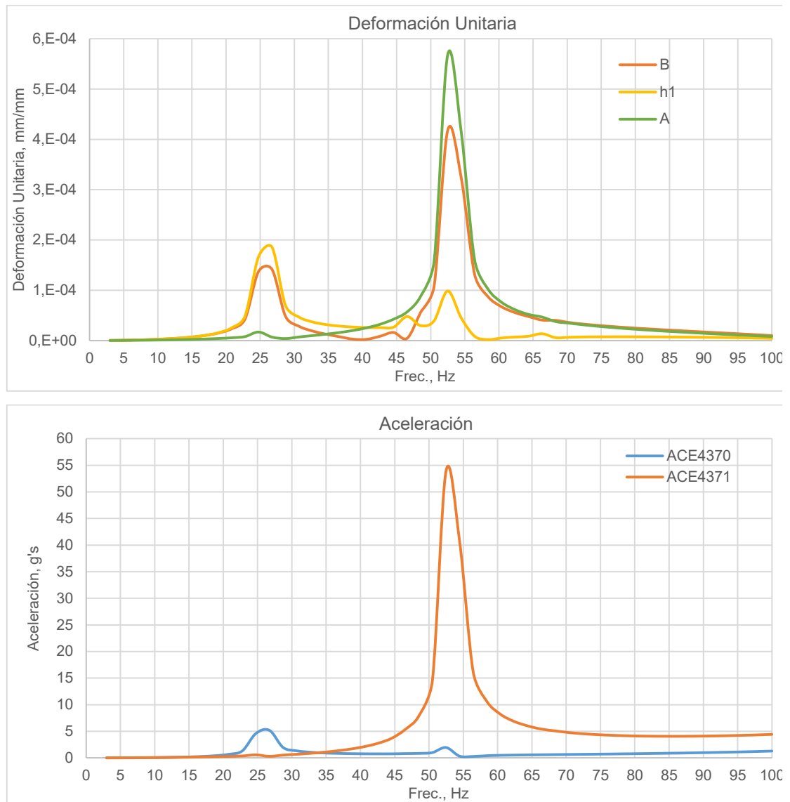
Figura 16: Respuesta armónica del mástil en dirección Y
