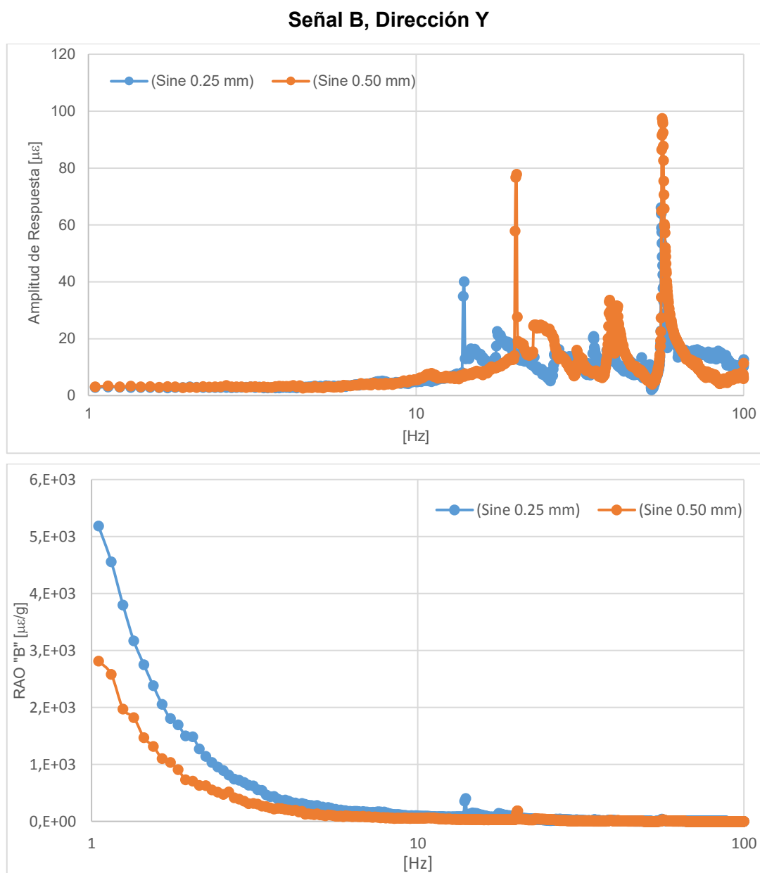
Figura 2.16: Respuesta de micro deformación unitaria en "B", dirección Y
