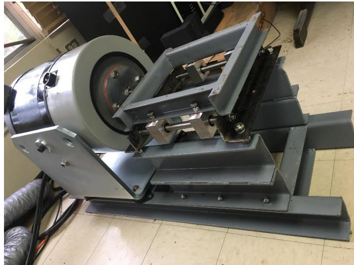
Figura 1.12: Mesa vibratoria construida
