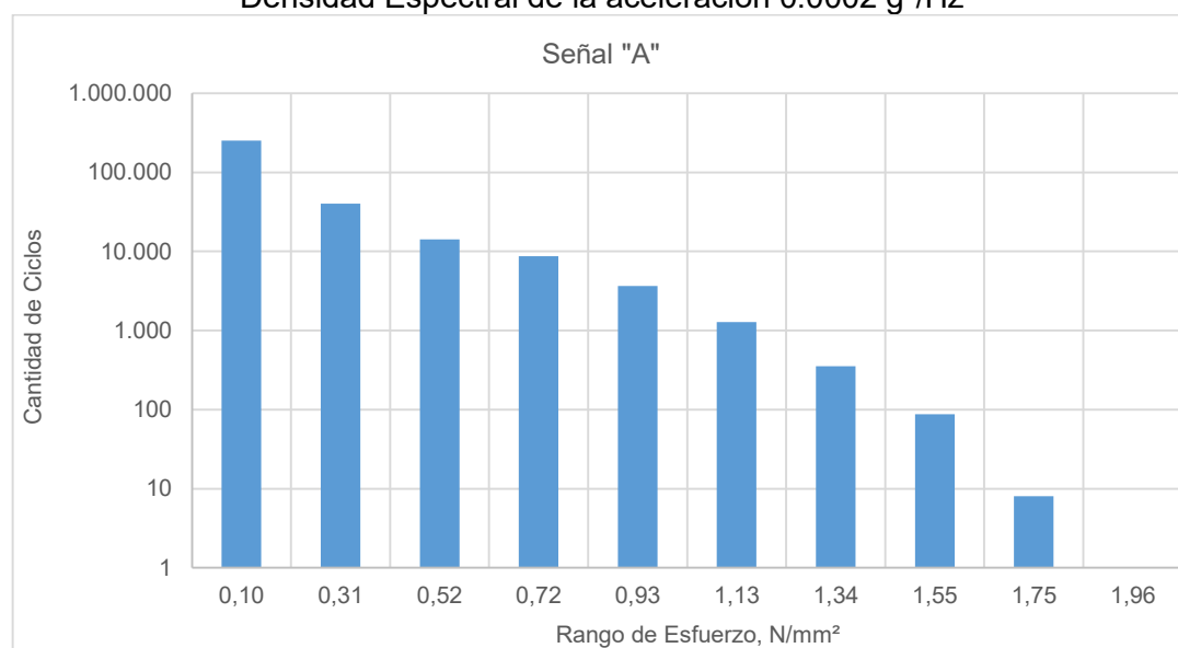
Figura 3.19: Cálculo de cantidad de ciclos para la señal "A", dirección "Y"
