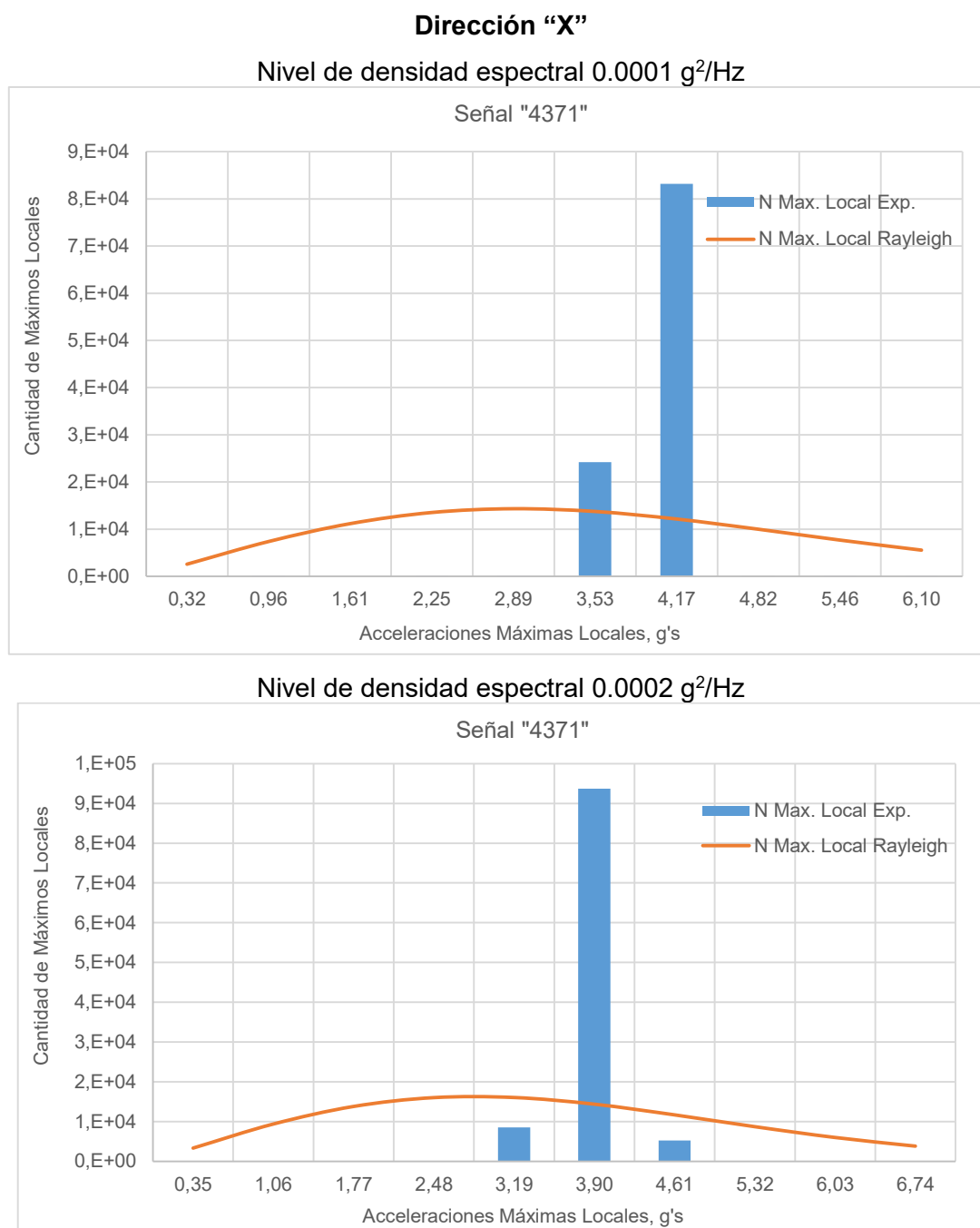
Figura 3.12: Cálculo de máximos locales para la señal "4371", dirección "X"
