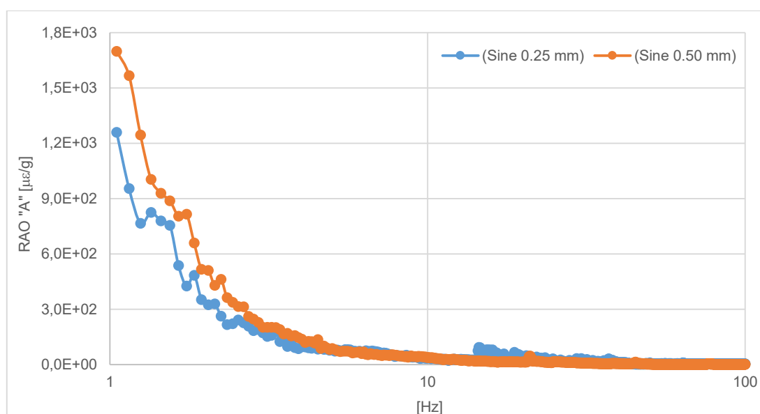
Figura 2.17: Respuesta de micro deformación unitaria en "A", dirección Y
