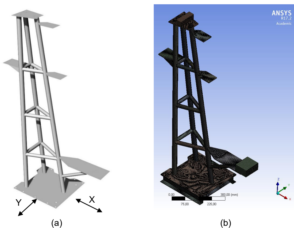
Figura 2.10: Modelo geométrico (a) y Modelo estructural (b)
