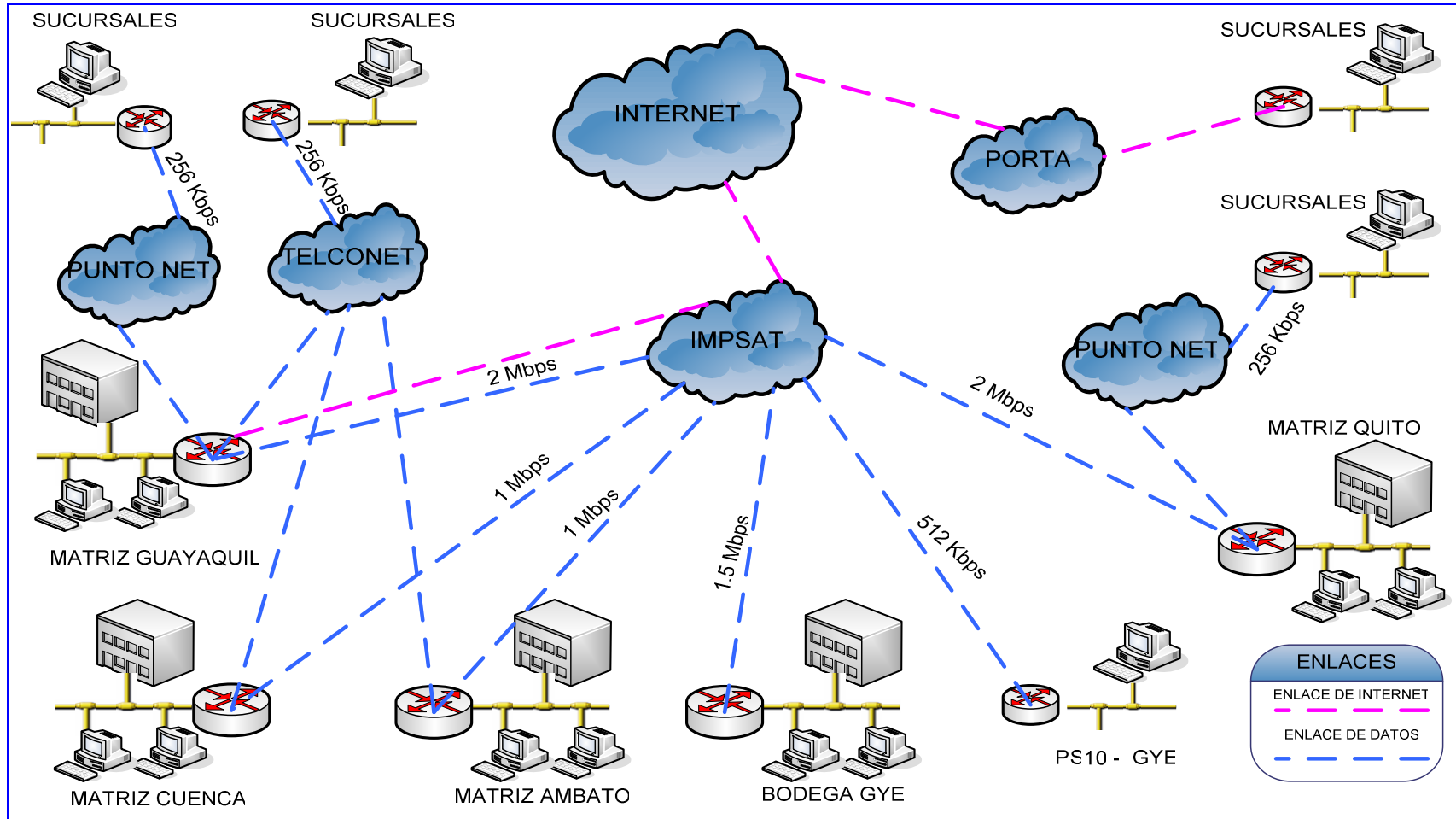
Figura 3.2 Asignación de Anchos de Banda de la Red de Datos de Servientrega
