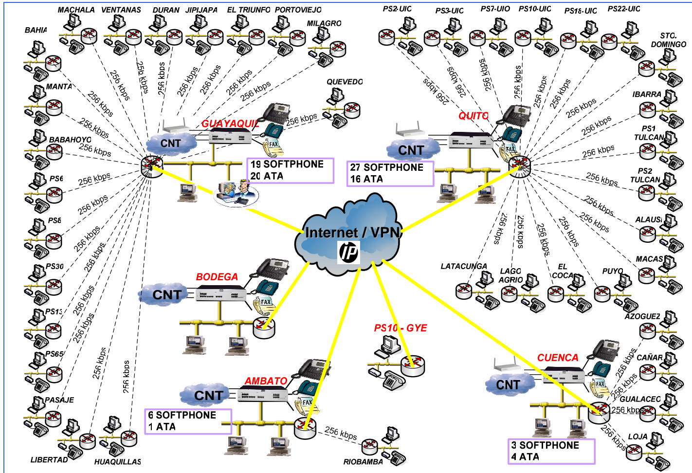
Figura 3.46 Estructura definitiva
