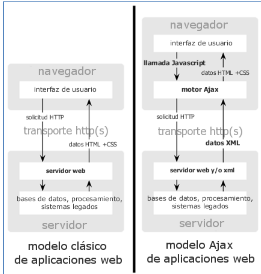
Figura 2.2 Representación del modelo clásico y modelo ajax.
