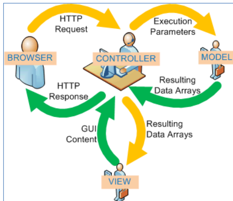
Figura 2.5 Funcionamiento Modelo Vista Controlador
