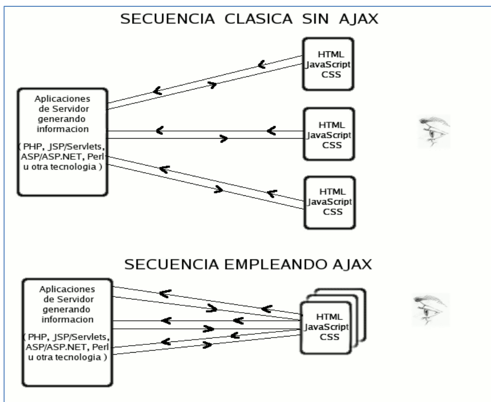
Figura 2.3 Secuencia clásica sin Ajax – Secuencia clásica con Ajax.
