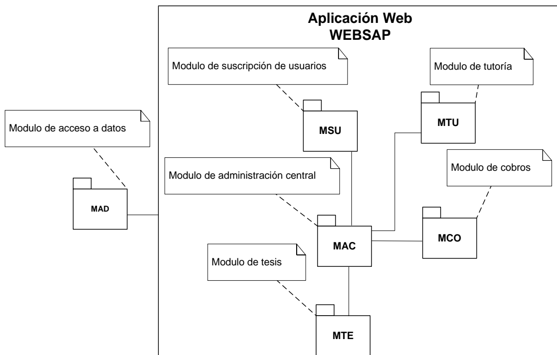
Figura 5.2 Módulos del Sistema.
