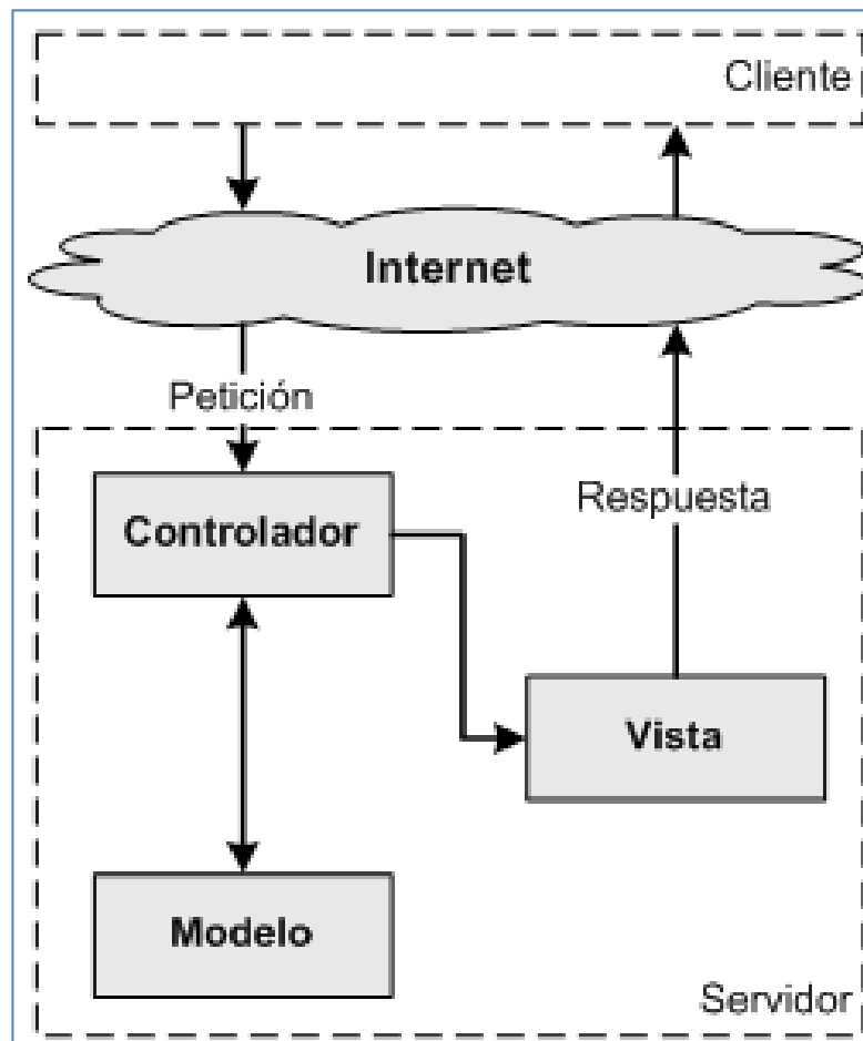
Figura 2.4 Esquema Modelo Vista Controlador
