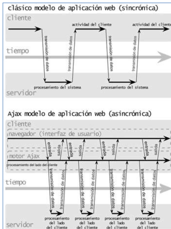
Figura 2.1 El patrón de interacción sincrónica y patrón asincrónico de una aplicación AJAX.
