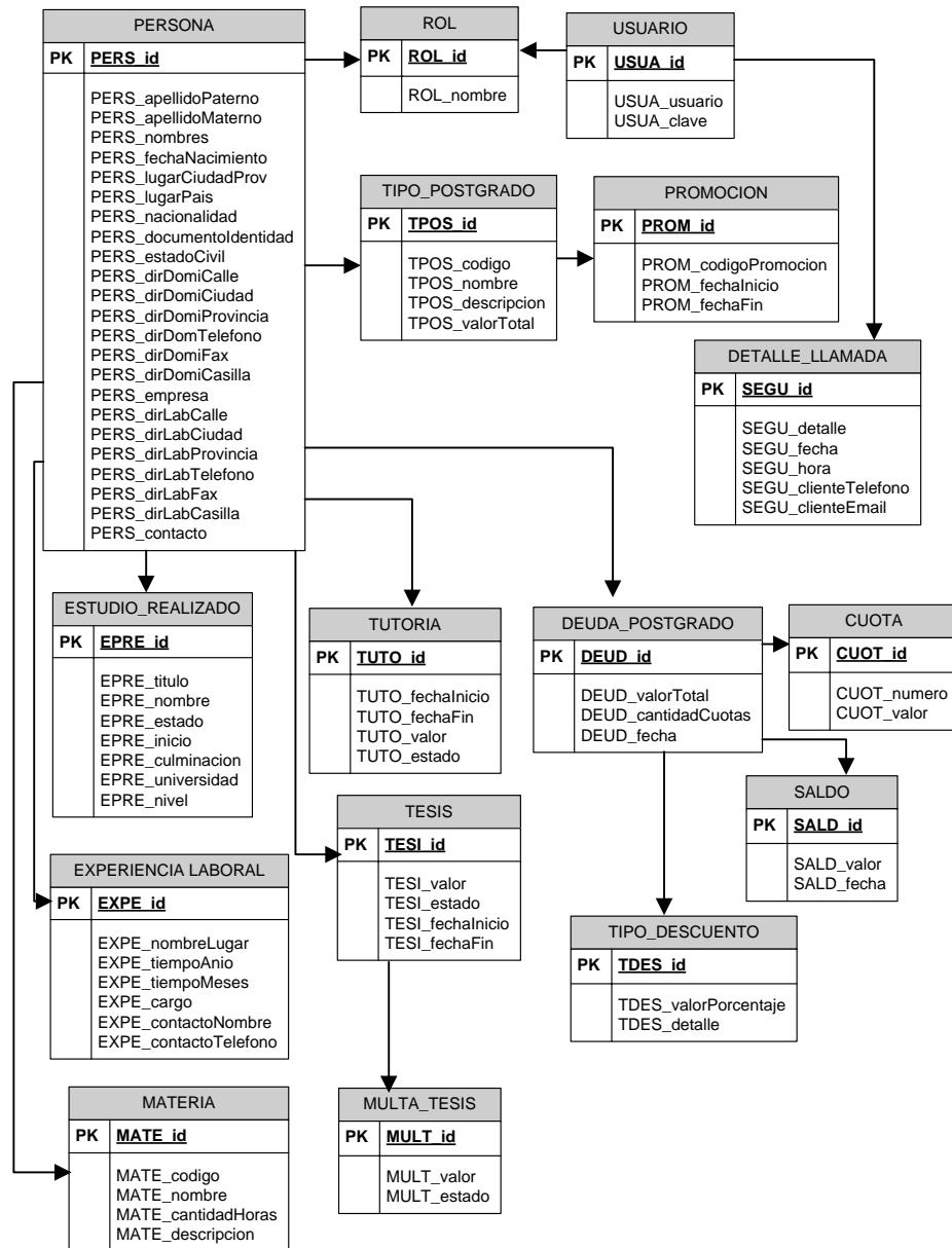
Figura 5.1: Modelo lógico de la base de datos.
