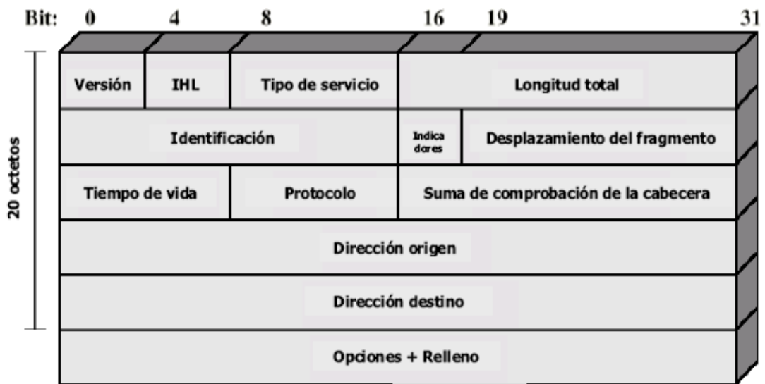
Figura A.2 Datagrama del protocolo IP [1]
