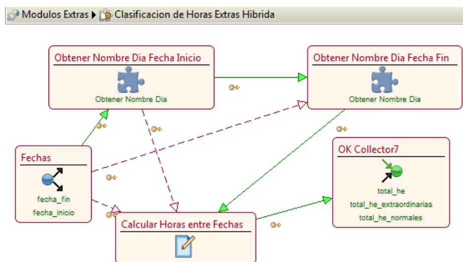
Figura 3.45 WebML del Módulo Clasificación de Horas Extras Hibrida
