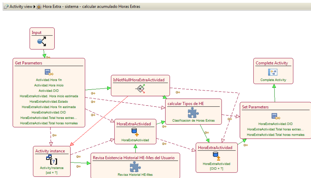
Figura 3.48 WebML del Módulo Calcular Acumulado Horas Extras
