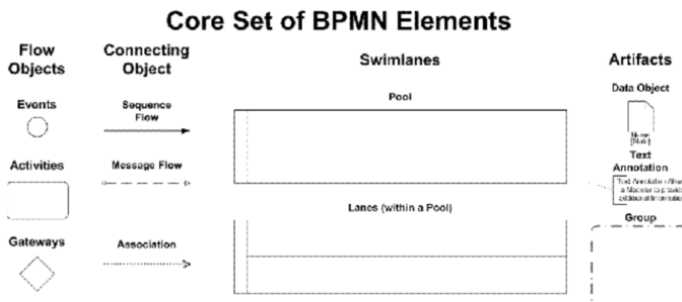
Figura 2.2 Notación BPMN
