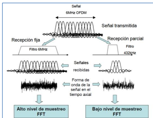
Figura 4.4.1 Procesamiento de señal en recepción banda ancha y recepción parcial. [23]
