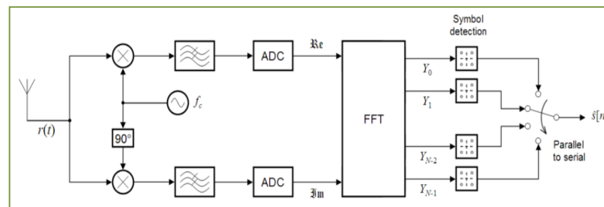
Figura 2.3.4.3 Receptor modelo de sistema OFDM [14]
