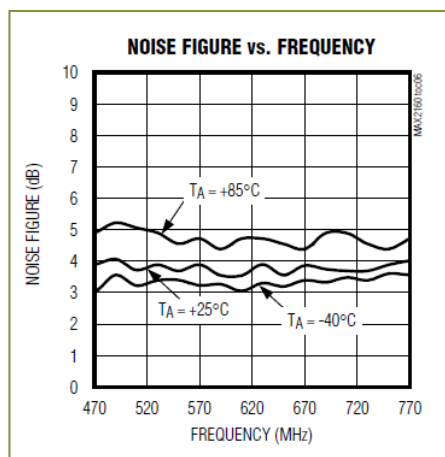
Figura 3.4.1.1 Frecuencia vs Ruido [25]
