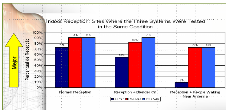
Figura 2.4.5 Comparación de la propagación de la señales [16]
