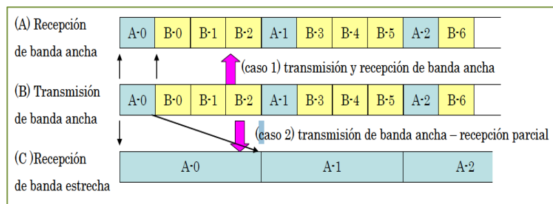
Figura 4.4.1 Flujo de transporte en transmisiones [23]
