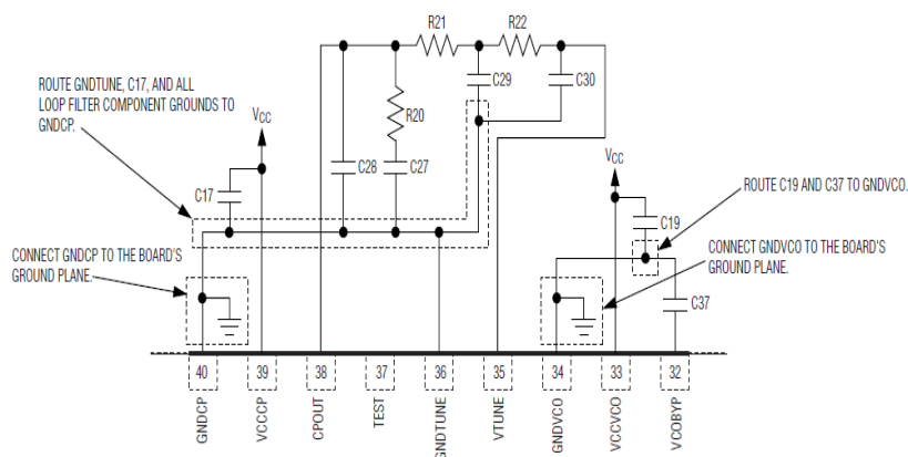
Figura 3.4.1.1.1 Diagrama del retorno a tierra de los componentes [25]
