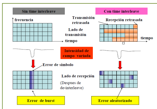
Figura 2.3.5.1.1 Efecto del time Interleave [15]
