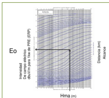
Figura 4.1.2 Altura de la antena de transmisión en metros [21]
