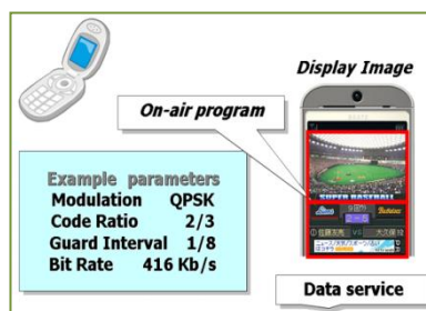
Figura 3.1 Esquema de funcionamiento One-Seg [16]
