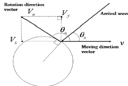
Figura 4.3.2 Modelo de recepción en un vehículo [22]
