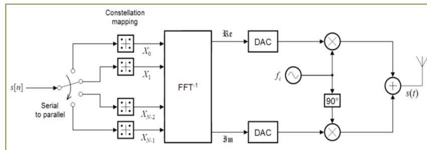
Figura 2.3.4.2 Transmisor modelo de sistema OFDM [14]
