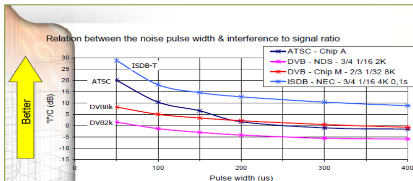
Figura 2.4.3 Relación señal ruido [16]
