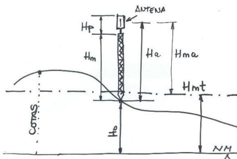
Figura 4.1.1 Punto de emisión [21]
