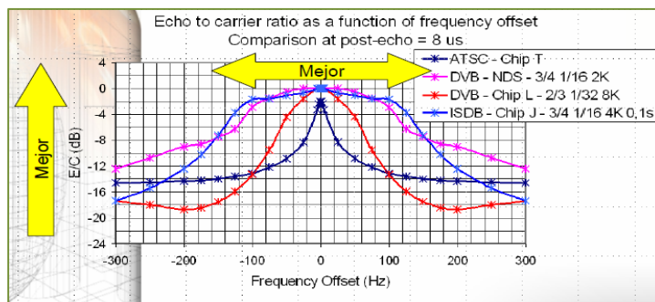
Figura 4.3.3.1 Respuesta de ISDB-T ante el efecto Doppler [16]
