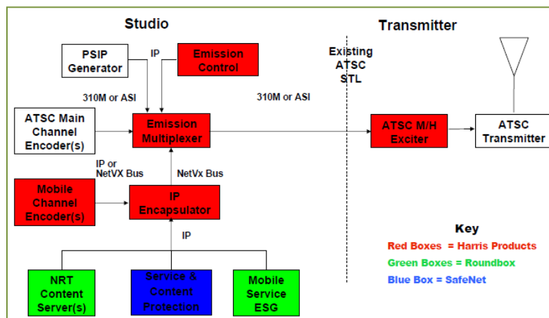
Figura 2.1.3 Arquitectura del Sistema ATSC [5]
