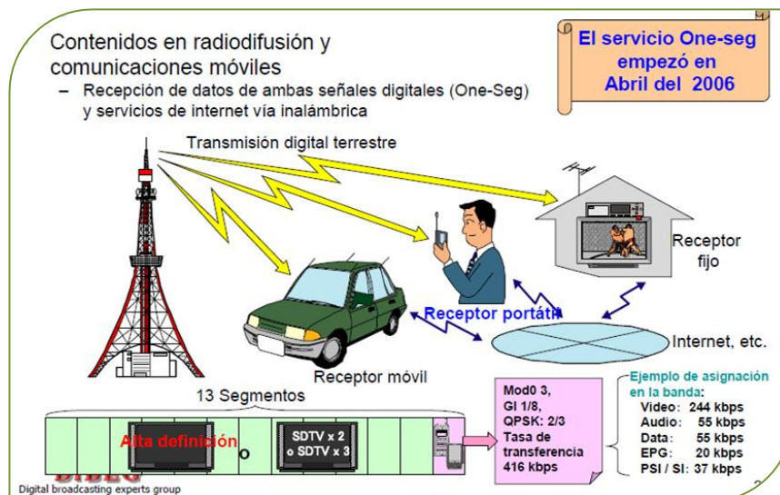
Figura 3.3.1 Formas de Recepción One-Seg [17]
