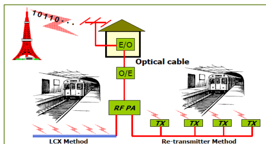
Figura 4.3.3.2 Método de retransmisión para trenes [16]
