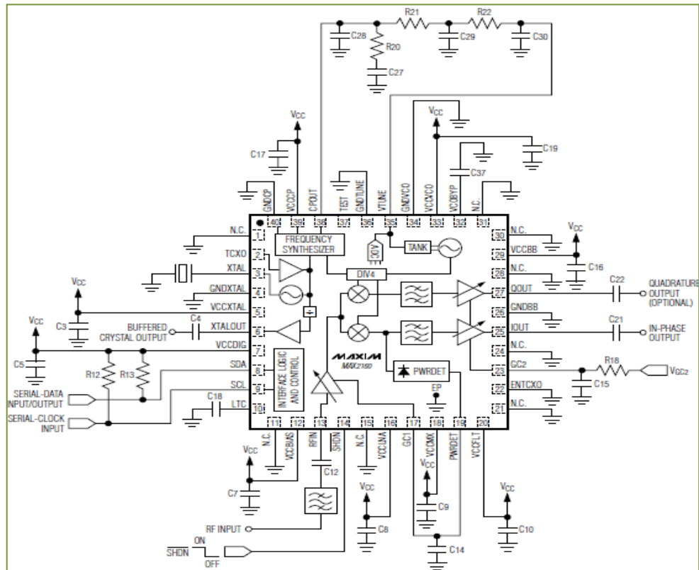
Figura 3.4.1.1.2 Diagrama interno del MAX2160/EBG de Maxim [25]
