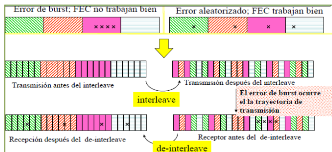
Figura 2.3.5 Ejemplo de corrección Interleave [15]
