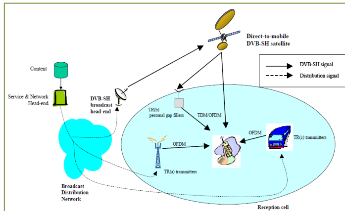
Figura 2.2.5 Arquitectura de transmisión del Sistema DVB-SH [11]
