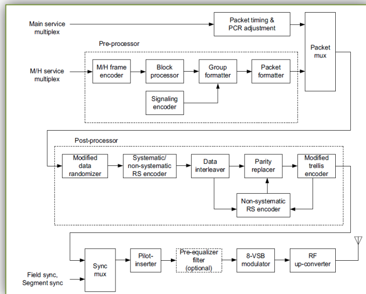
Figura 2.1.3.1 Proceso de Transmisión [6]
