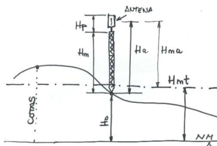
Figura 4.1.1.3 Ubicación de la antena [21]
