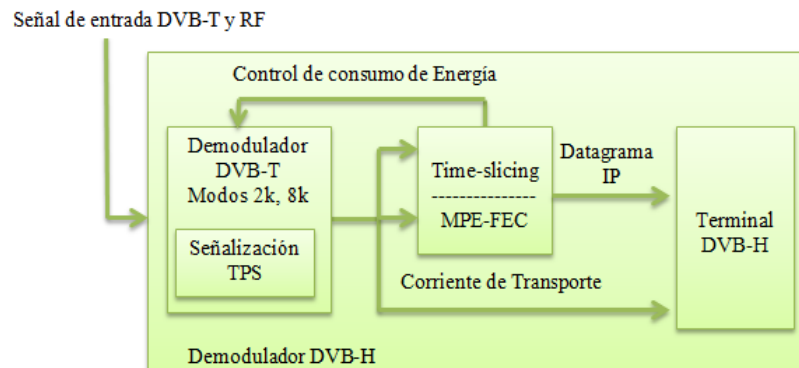
Figura 2.2.4.2 Estructura del Receptor DVB-H [30]
