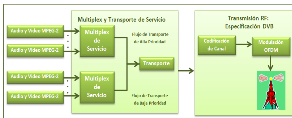
Figura 2.2.3 Diagrama general del Sistema DVB-T [30]
