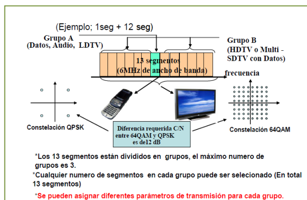
Figura 2.3.2 Estructura segmentada y recepción parcial [12]
