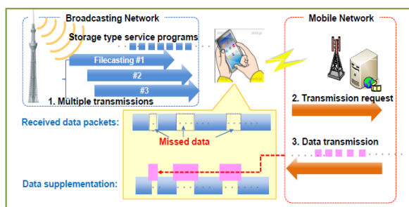
Figura 2.3.6.2 Estructura del sistema de transmisión de datos [15]
