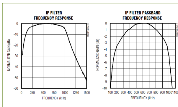
Figura 3.4.1.2 Respuestas de Frecuencia intermedia [25]
