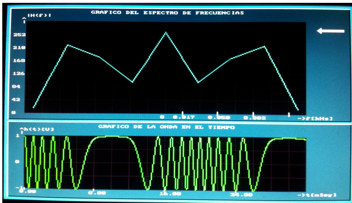
Figura 11 Gráfica de la señal FM en el dominio de la frecuencia ZOOM IN
