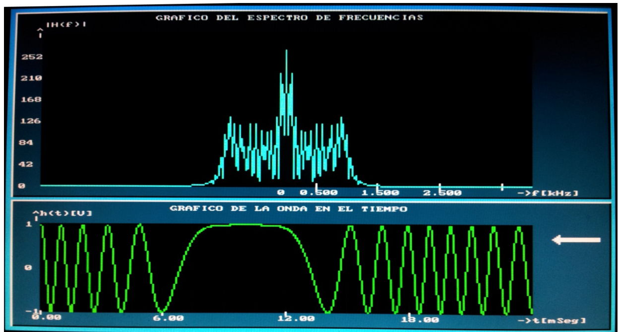
Figura 5 Gráfica de la señal FM en el dominio del tiempo ZOOM IN x2
