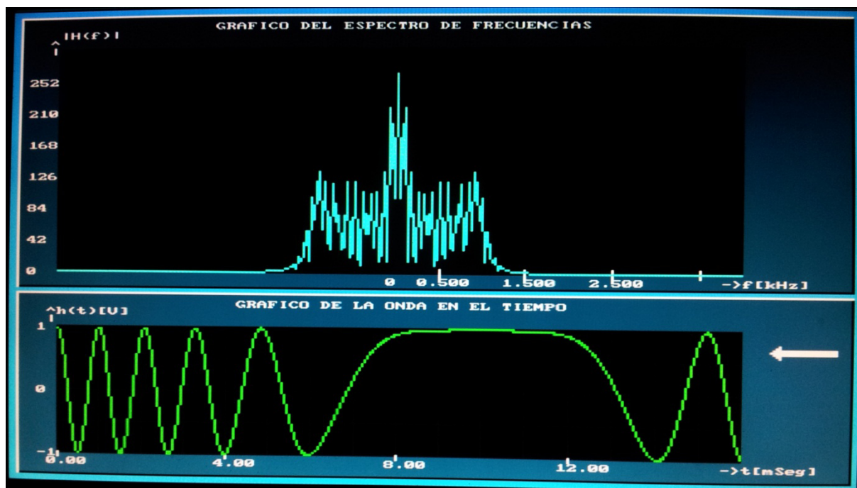
Figura 6 Gráfica de la señal FM en el dominio del tiempo ZOOM IN x3
