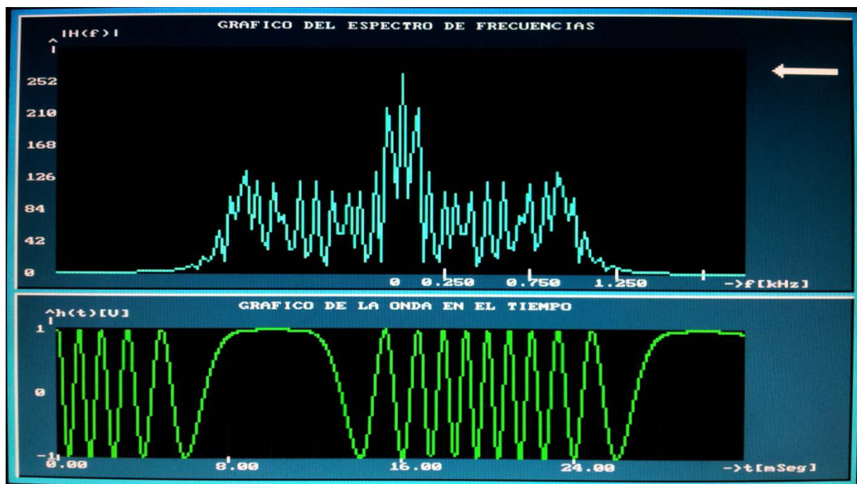
Figura 9 Gráfica de la señal FM en el dominio de la frecuencia ZOOM IN
