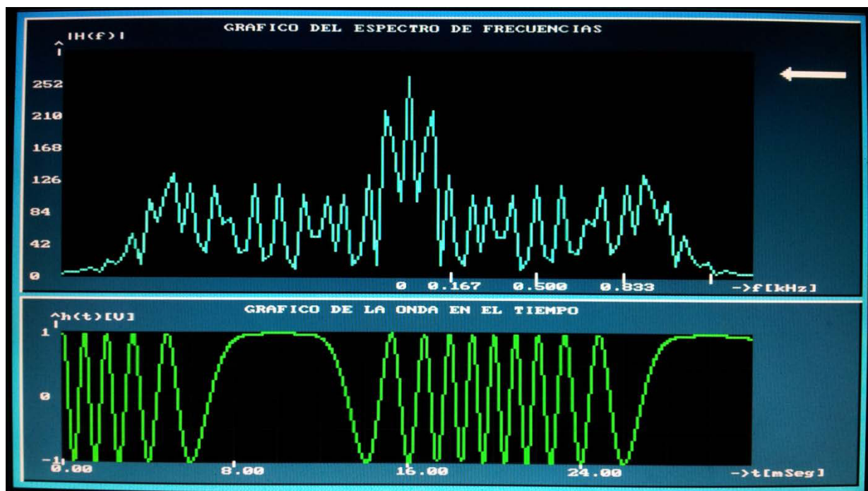
Figura 10 Gráfica de la señal FM en el dominio de la frecuencia ZOOM IN
