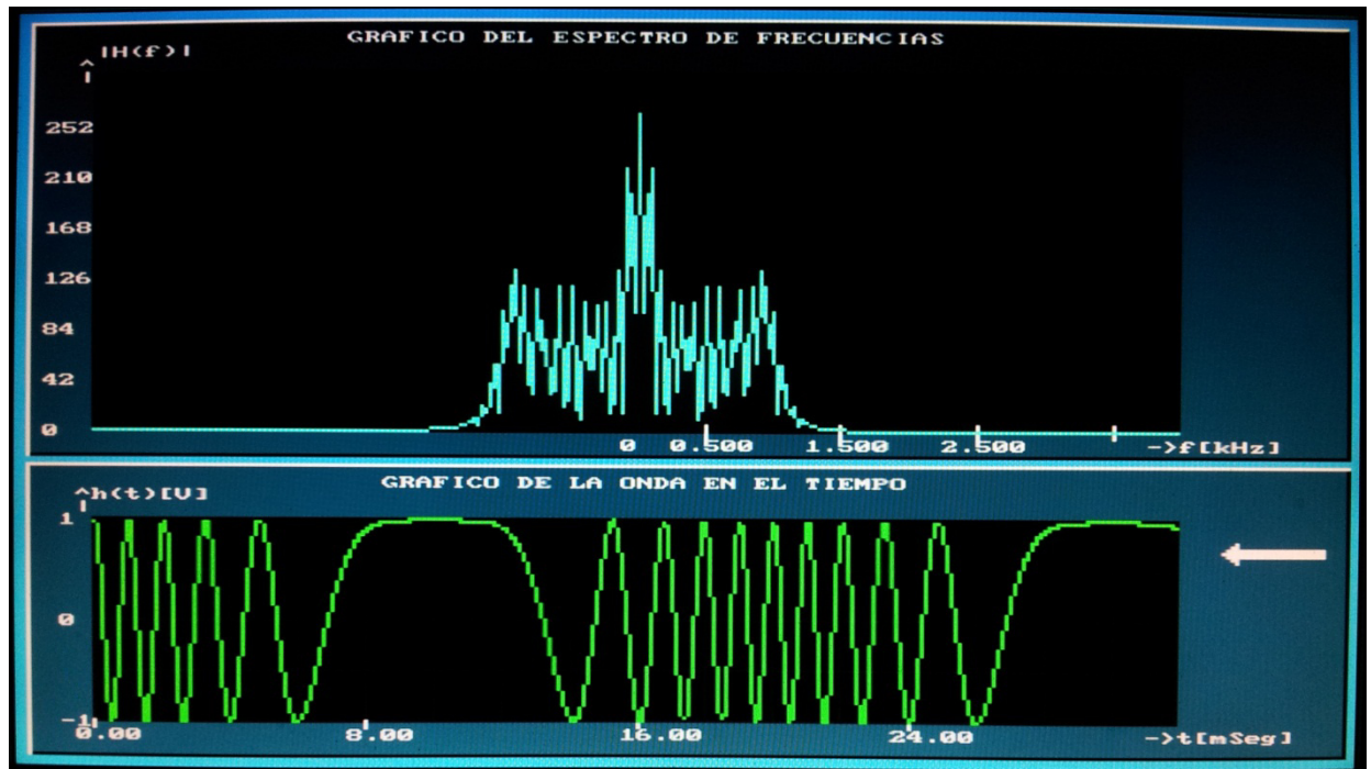
Figura 4 Gráfica de la señal FM en el dominio del tiempo ZOOM IN x1
