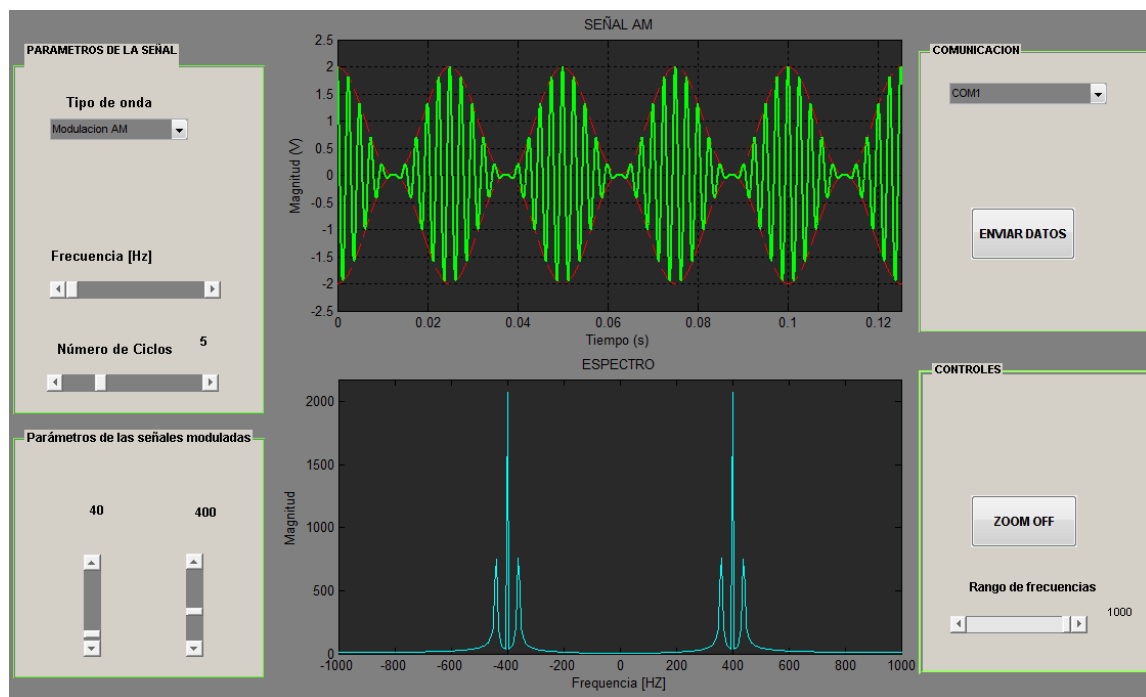
Figura 3-12 Ventana del Generador configurada para señal AM
