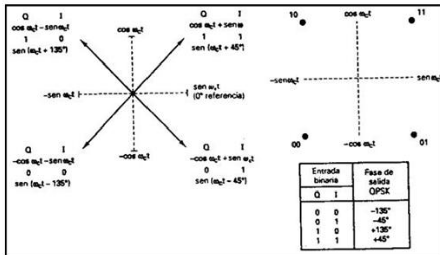
Figura 4.35 Diagrama de Constelaciones Modulador QPSK
