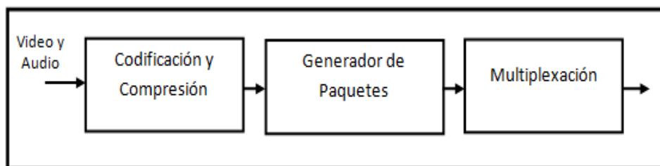
Figura 4.10 Diagrama de Bloques – Codificación Transporte de Paquetes y Multiplexación de Señales de Audio y Video
