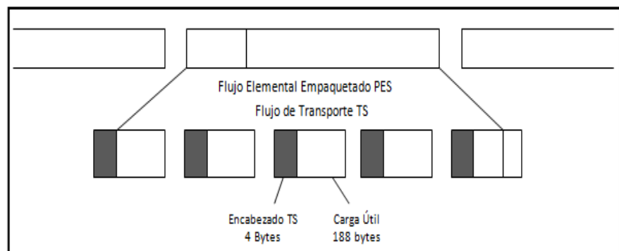
Figura 4.22 Paquete de Flujo de Transporte
