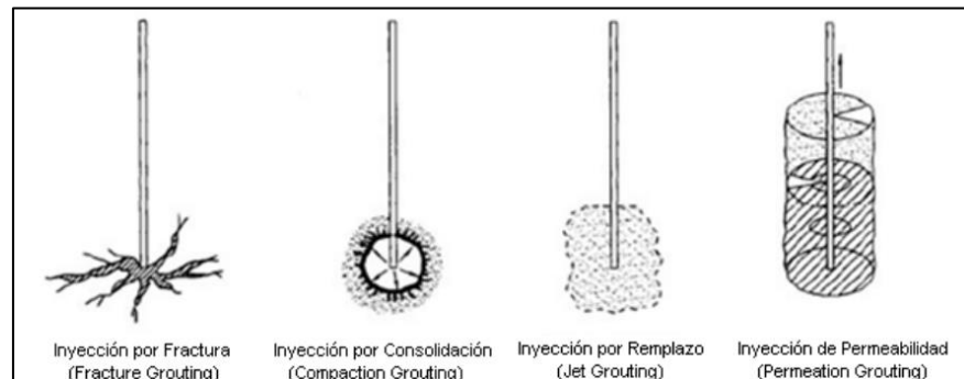
Figura 6.6. Inyección de Cemento.
