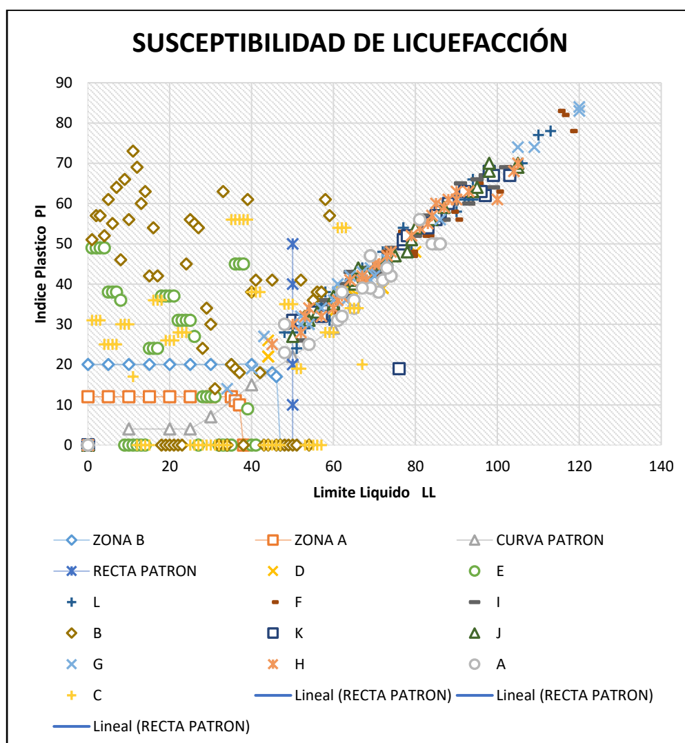
Figura 3.5. Curva con las zonas potencialmente licuables propuestas por Seed, 2003, junto con las diferentes muestras de cada perforación.
