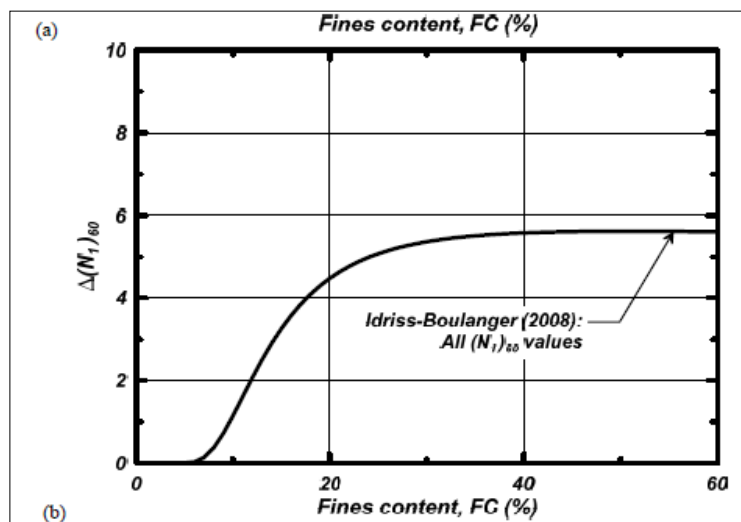
Figura 4.5. Contenido de Finos. Fuente: Idriss & Boulanger, 2008.
