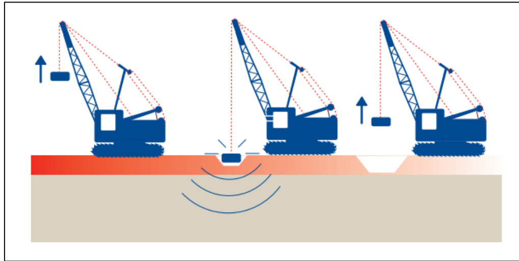
Figura 6.4. Compactación Dinámica. Fuente: Menard México, 2013
