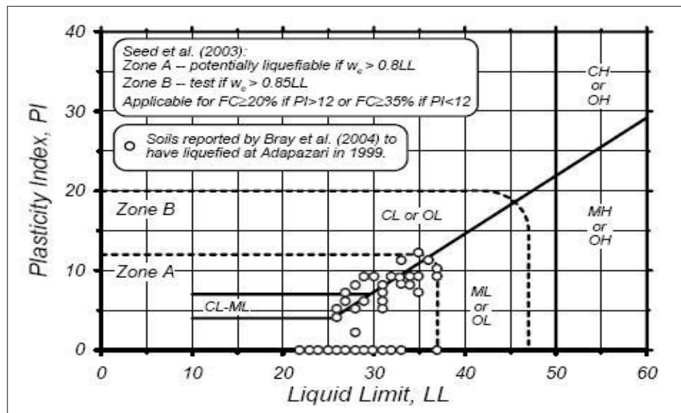
Figura 3.4. Zonas Susceptibles a licuefacción. Fuente: Seed, 2003
