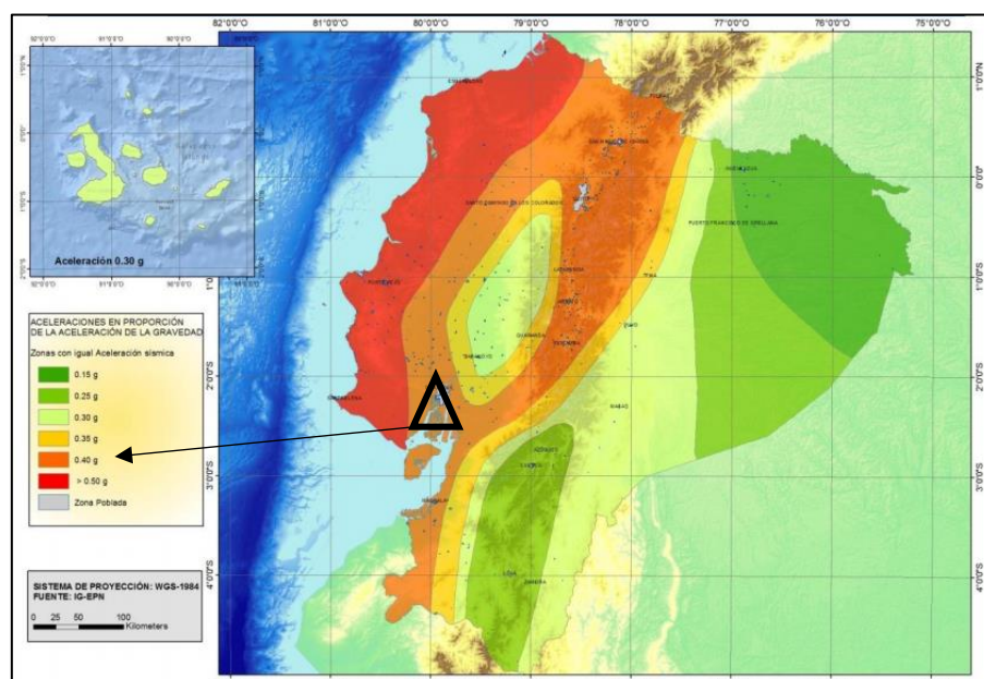
Figura 4.1. Mapa de Peligrosidad Sísmica del Ecuador. Fuente: NEC, 2015
