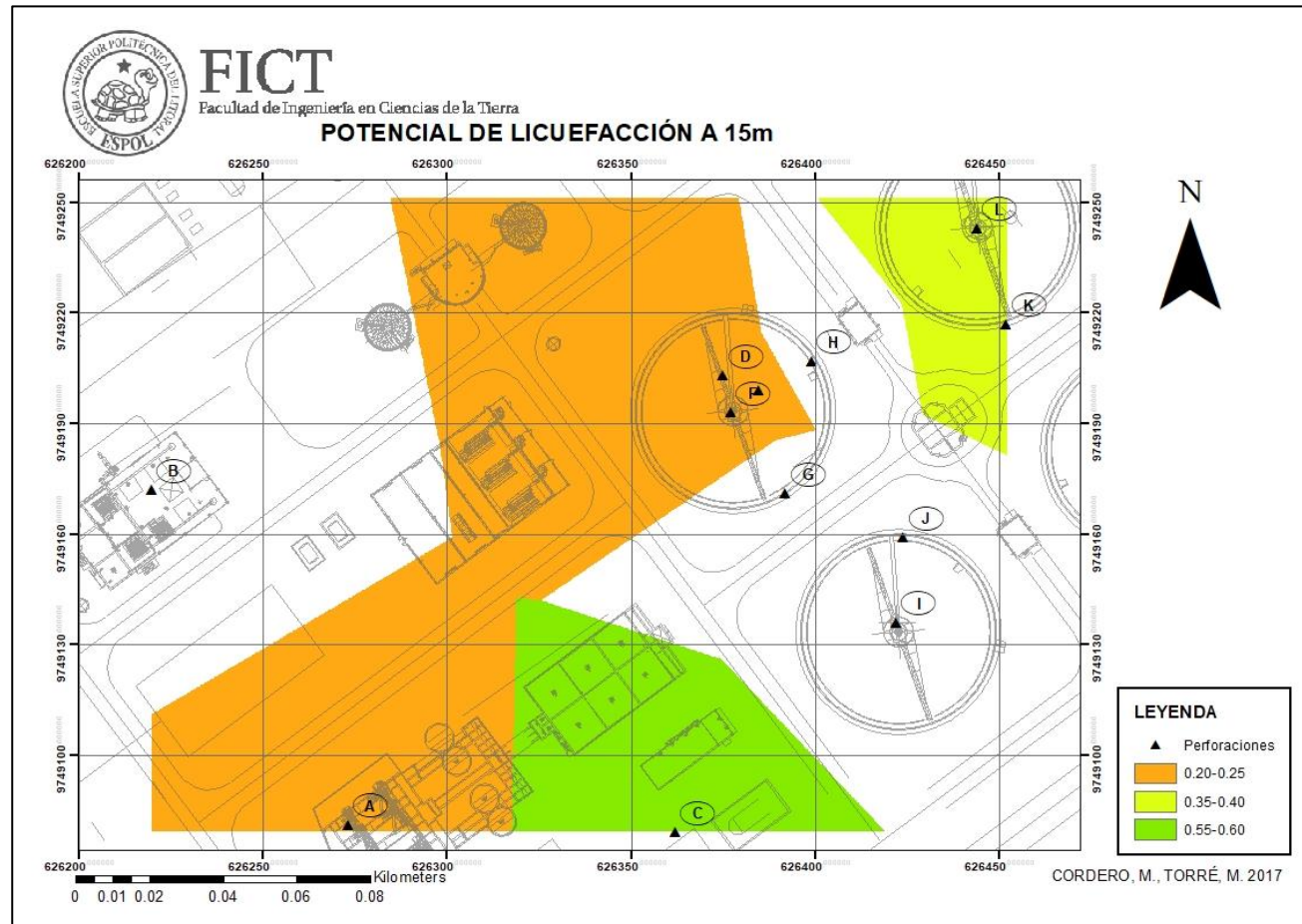
Figura 5.5. Mapa representativo del Potencial de Licuefacción a 15m de profundidad. Fuente: Cordero, M., Torre, M. 2017
