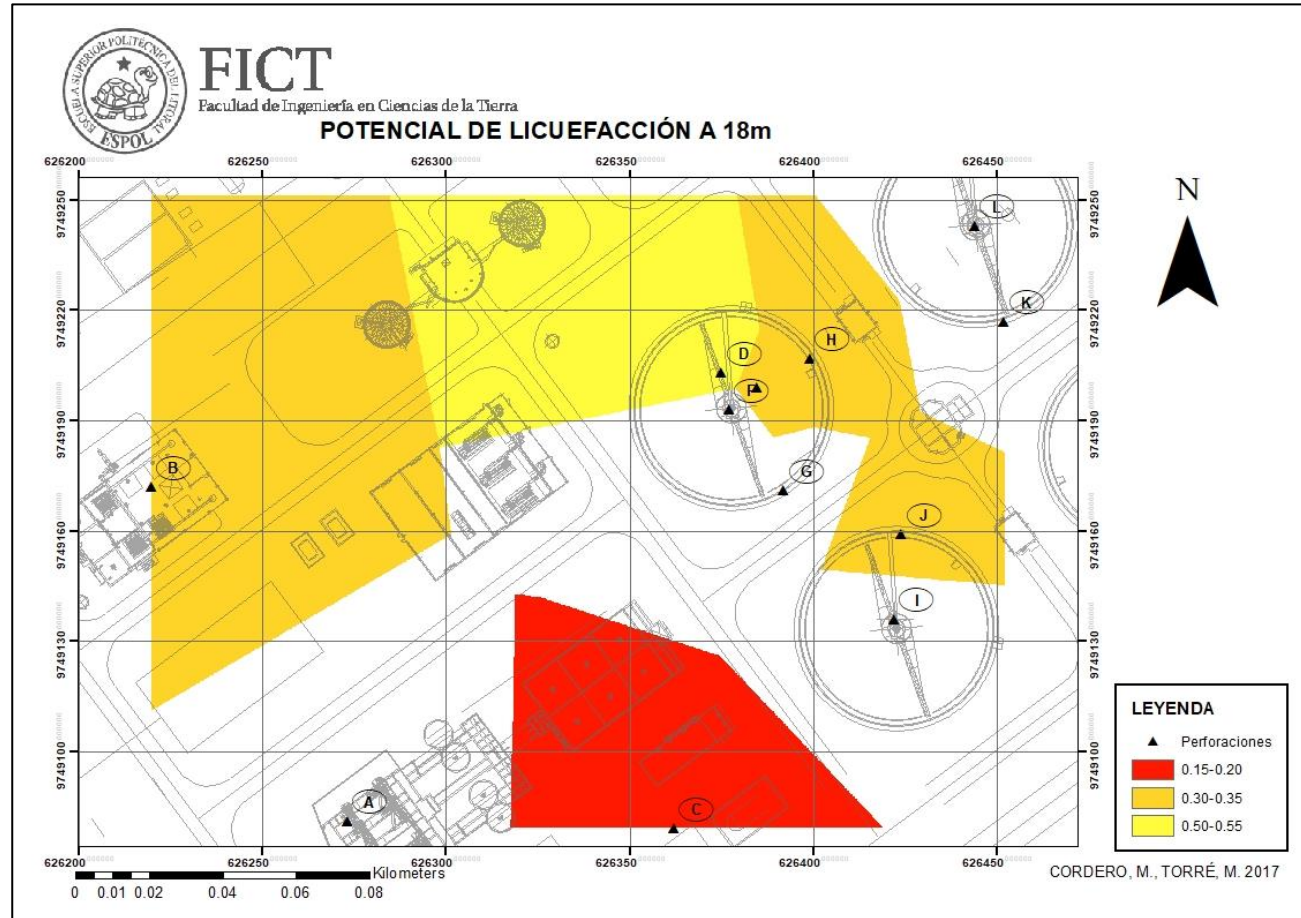
Figura 5.6. Mapa representativo del Potencial de Licuefacción a 18m de profundidad. Fuente: Cordero, M., Torre, M. 2017
