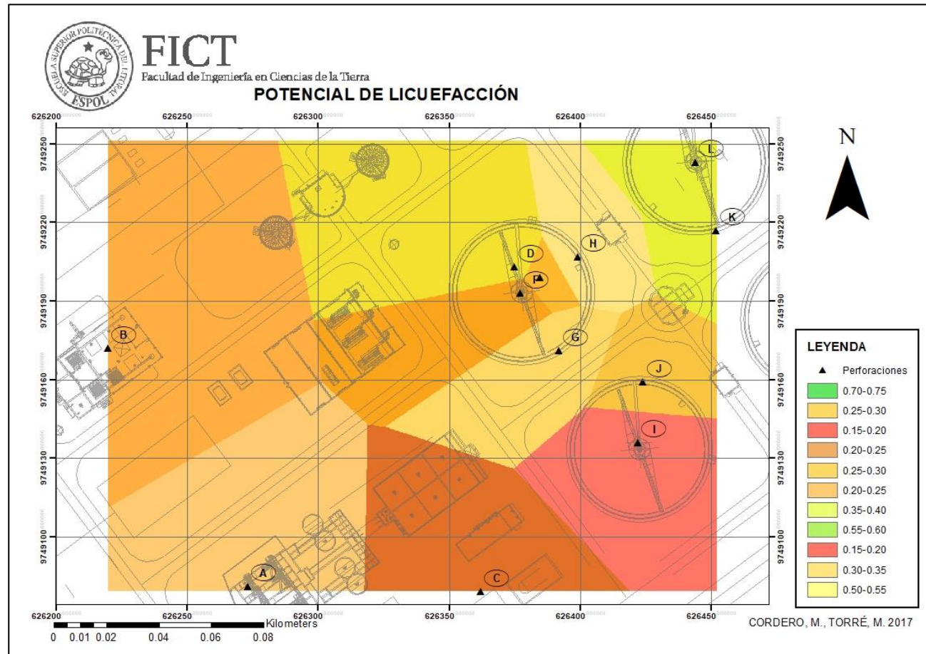
Figura 5.7. Mapa representativo del Potencial de Licuefacción para cada Perforación. Fuente: Cordero, M., Torre, M. 2017
