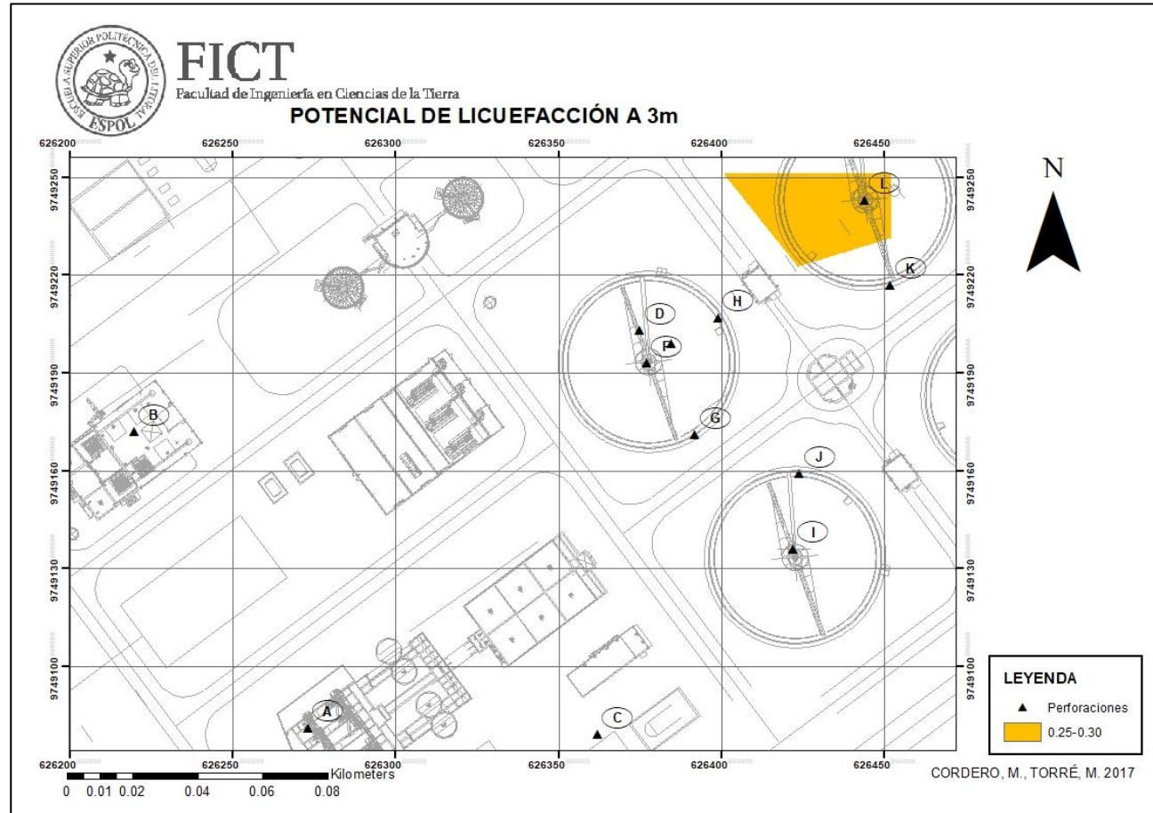
Figura 5.2. Mapa representativo del Potencial de Licuefacción a 3m de profundidad.
