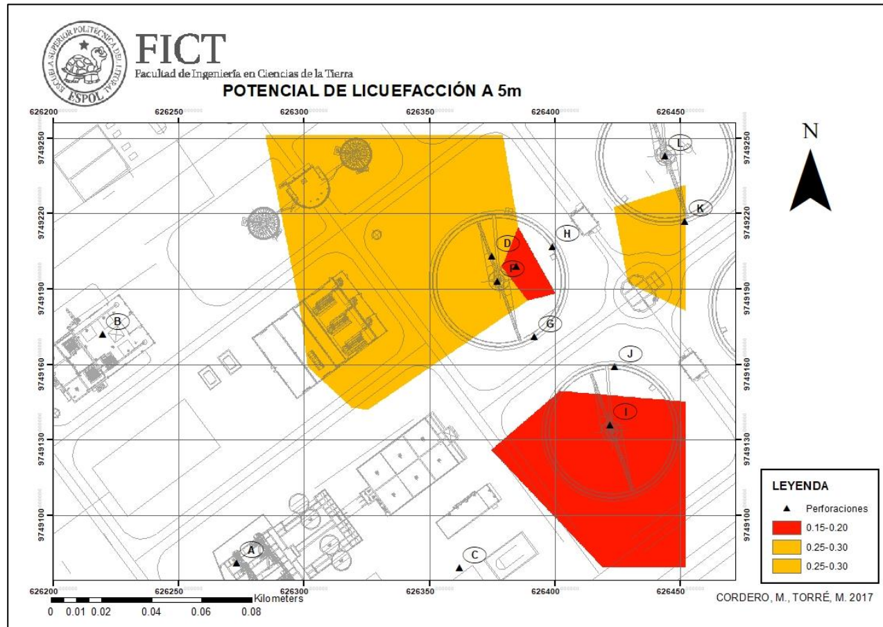
Figura 5.3. Mapa representativo del Potencial de Licuefacción a 5m de profundidad.
