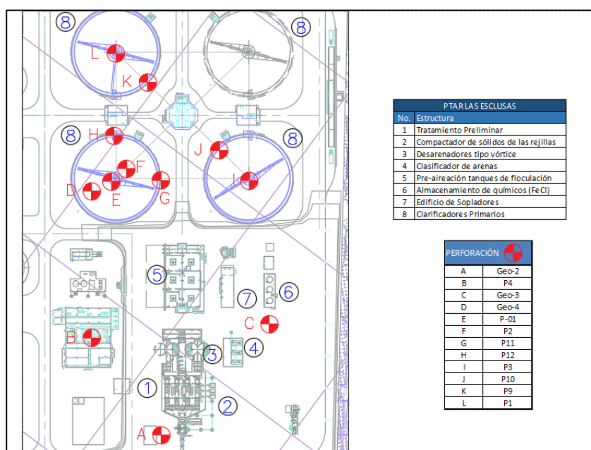
Figura 2.2. Ubicación de las Perforaciones. Fuente: Cordero, M., Torr , M. 2017
