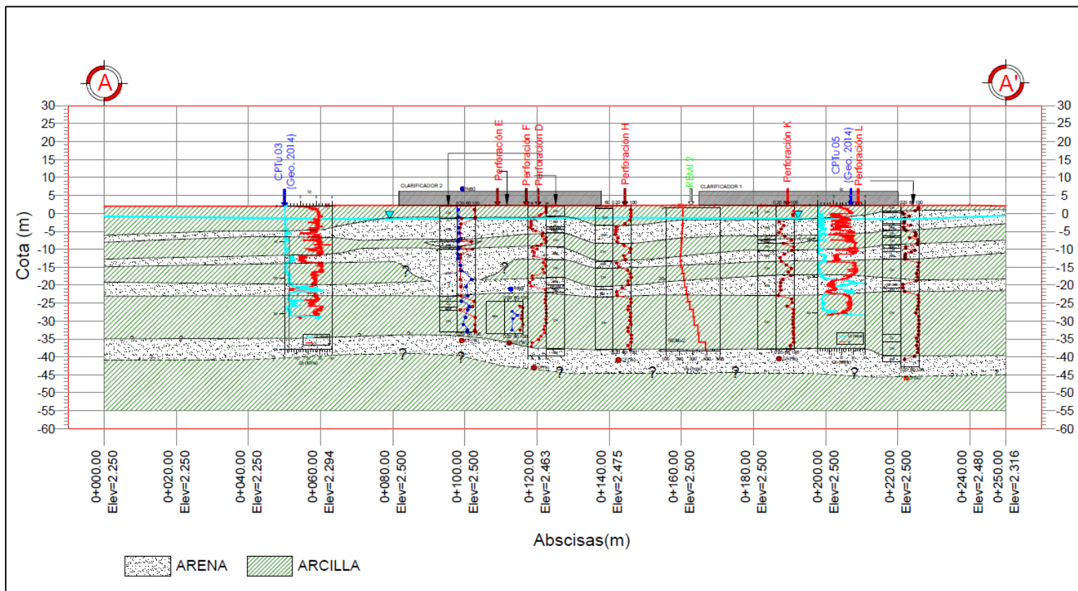
Figura 3.1. Perfil estratigráfico A-A'.- Se observan capas de suelo arena limosa a diferentes profundidades. Fuente: Cordero, M., Torr , M. 2017
