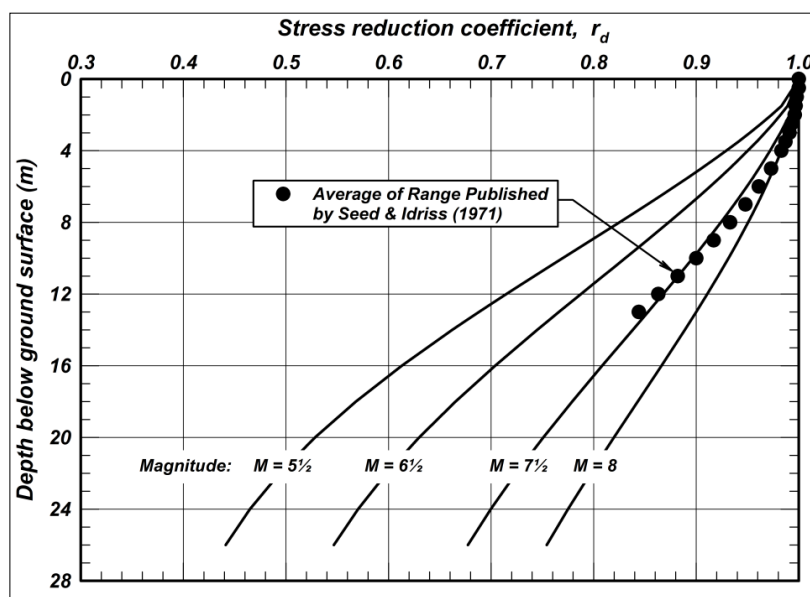
Figura 4.2. Coeficiente de Reducción ( r_d ). Fuente: Seed, Idriss, 1971.
