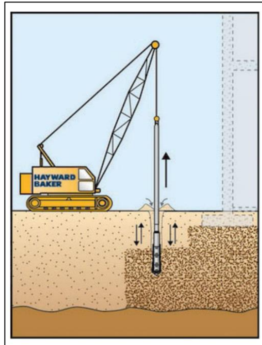
Figura 6.5. Vibro Compactación. Fuente: Hayward Baker, 2009
