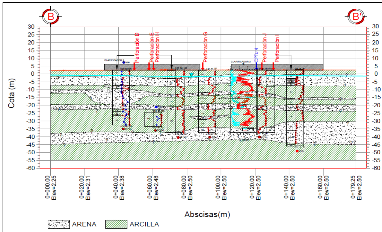
Figura 3.2. Perfil estratigráfico B-B'.- Se observan cuatro capas de suelo arena limosa a diferentes profundidades.
