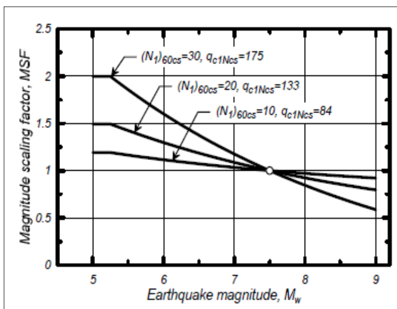
Figura 4.4. Variación de MSF con q_{c1Ncs} y N_{160cs} para suelos cohesivos.
