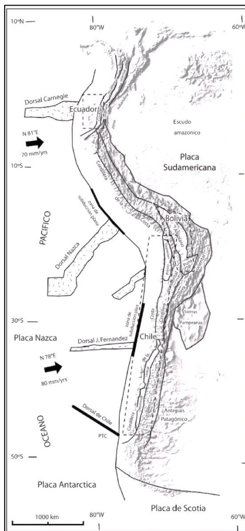
Figura 2.1. Ubicación de las Placas y fracturas involucradas en el sector.
