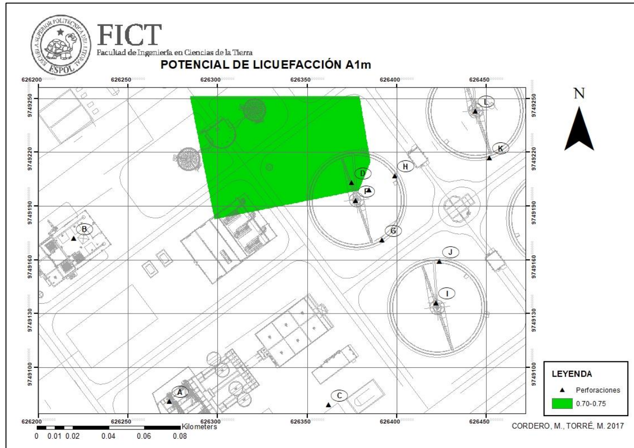
Figura 5.1. Mapa representativo del Potencial de Licuefacción a 1m de profundidad. Fuente: Cordero, M., Torre M. 2017
