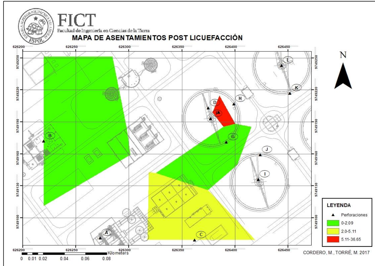
Figura 5.8. Mapa representativo de los asentamientos post-licuefacción. Fuente: Cordero, M., Torre, M. 2017
