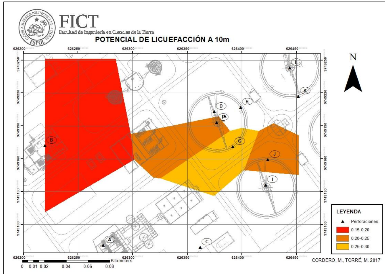
Figura 5.4. Mapa representativo del Potencial de Licuefacción a 10m de profundidad. Fuente: Cordero, M., Torre, M. 2017
