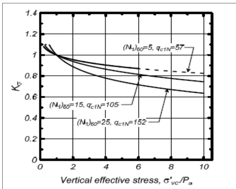
Figura 4.3. Factor de corrección por presión de confinamiento.
