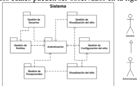
Figura 3. Casos de uso de alto nivel.
