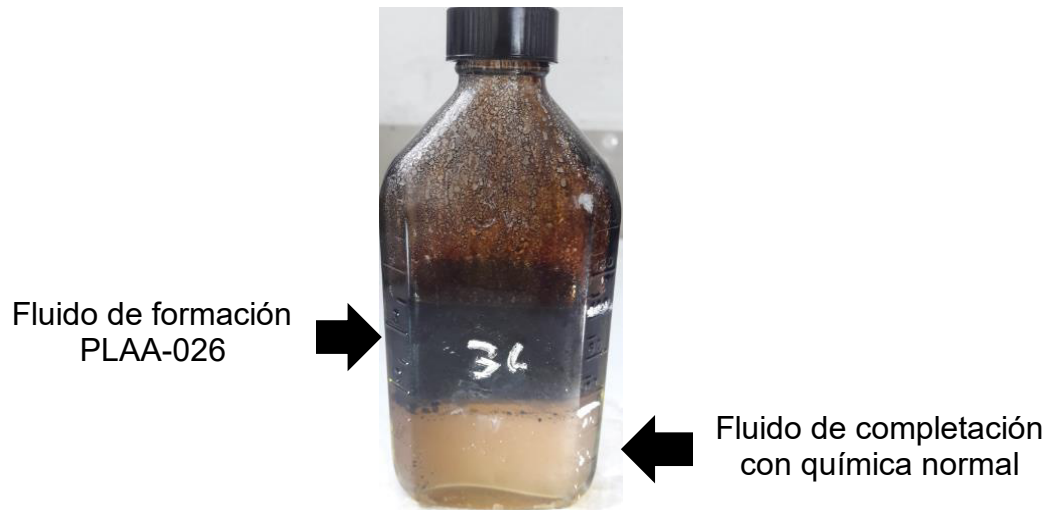
Figura 3.12. Resultado de la mezcla prueba 36 del PLAA-016 [Dynadrill S.A., 2018]
