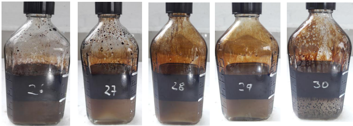
Figura 3.22. Resultado de la mezcla pruebas 27, 28, 29 y 30 de fluido de completación con nanotecnología del PLAD-034H [Dynadrill S.A., 2018]
