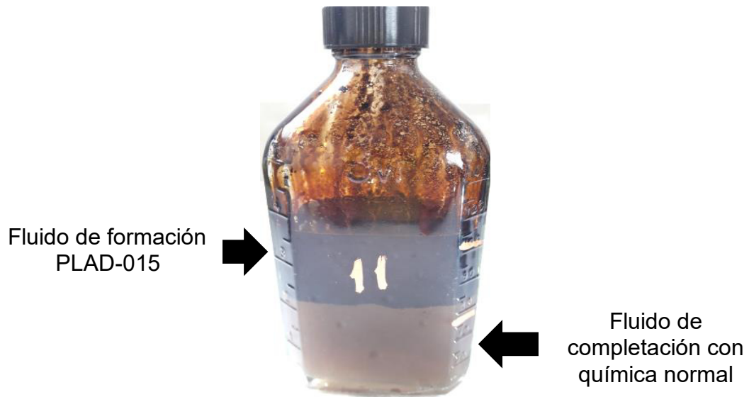
Figura 3.7. Resultado de la mezcla prueba 11 del PLAD-015 [Dynadrill S.A., 2018]
