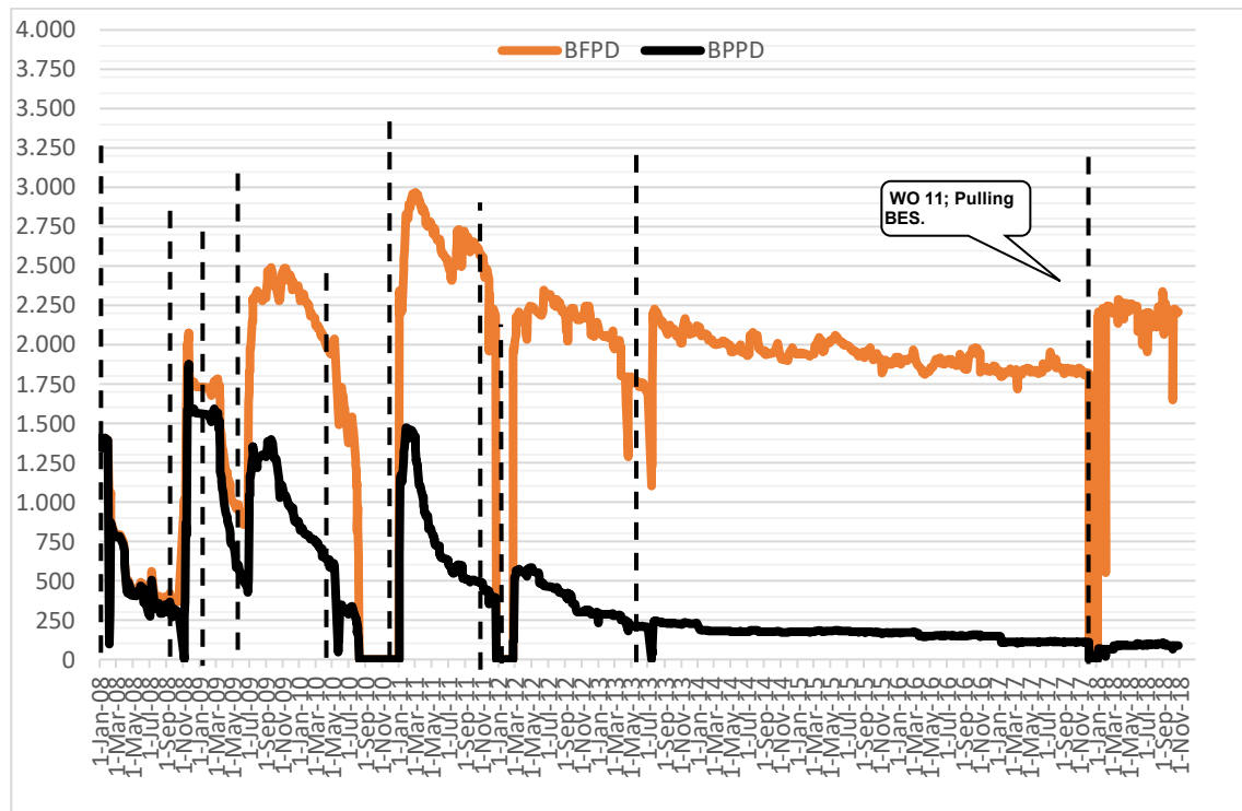
Figura 3.2 Historial de producción pozo Palo Azul-12 [Petroamazonas E.P., 2018]
