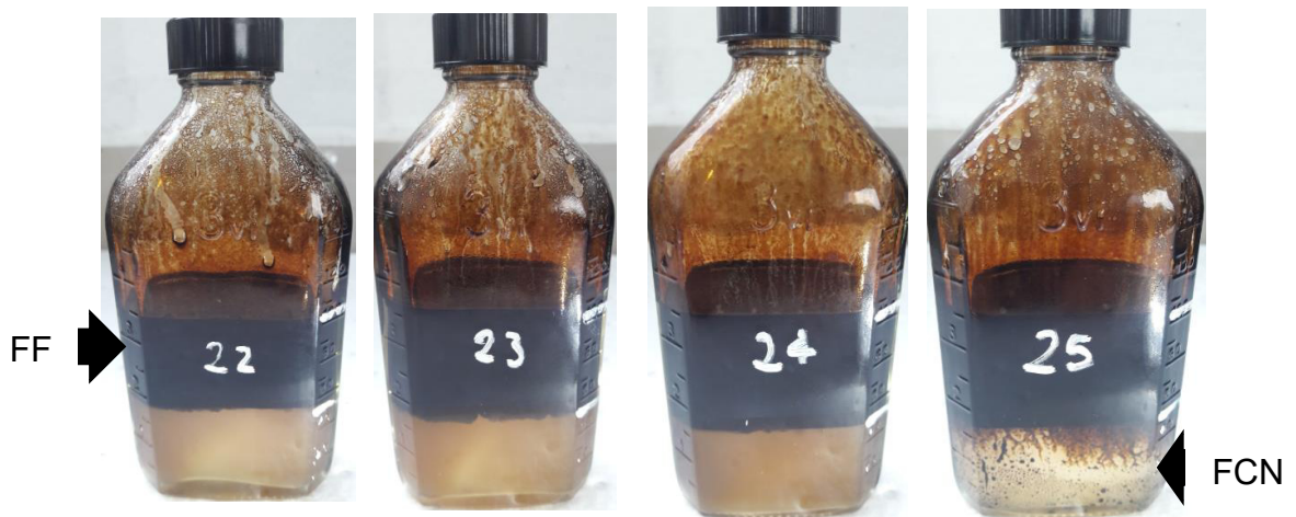
Figura 3.19. Resultado de la mezcla prueba 22, 23, 24 y 25 de fluido de completación con nanotecnología del PLAC-017 [Dynadrill S.A., 2018]
