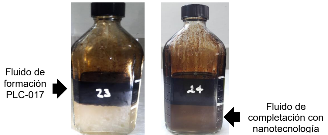
Figura 3.21. Resultado de la mezcla pruebas 23 y 24 de fluido de completación con surfactante diferente PLAC-017 [Dynadrill S.A., 2018]
