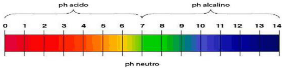
Figura 1.5. Escala de pH [Hopp,2005]
