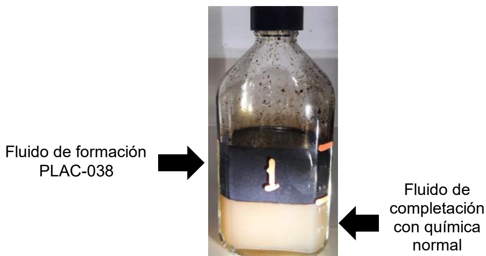
Figura 3.5. Resultado de la mezcla prueba 01 del PLAC-038 [Dynadrill S.A., 2018]
