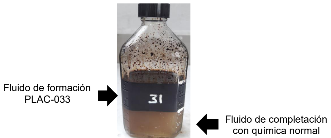
Figura 3.11. Resultado de la mezcla prueba 26 del PLAC-033 [Dynadrill S.A., 2018]
