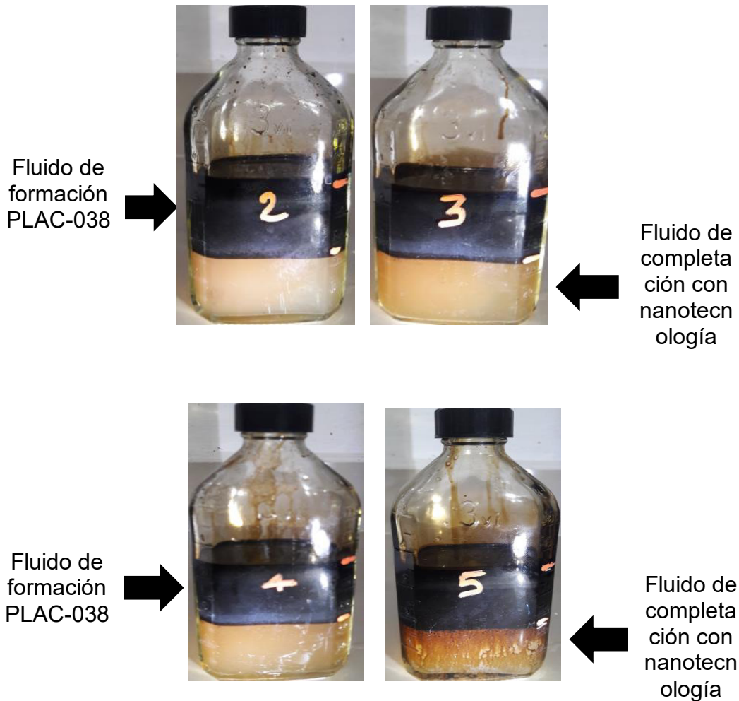
Figura 3.14. Resultado de la mezcla pruebas 02, 03, 04 y 05 de fluido de completación con nanotecnología del PLAC-038 [Dynadrill S.A., 2018]
