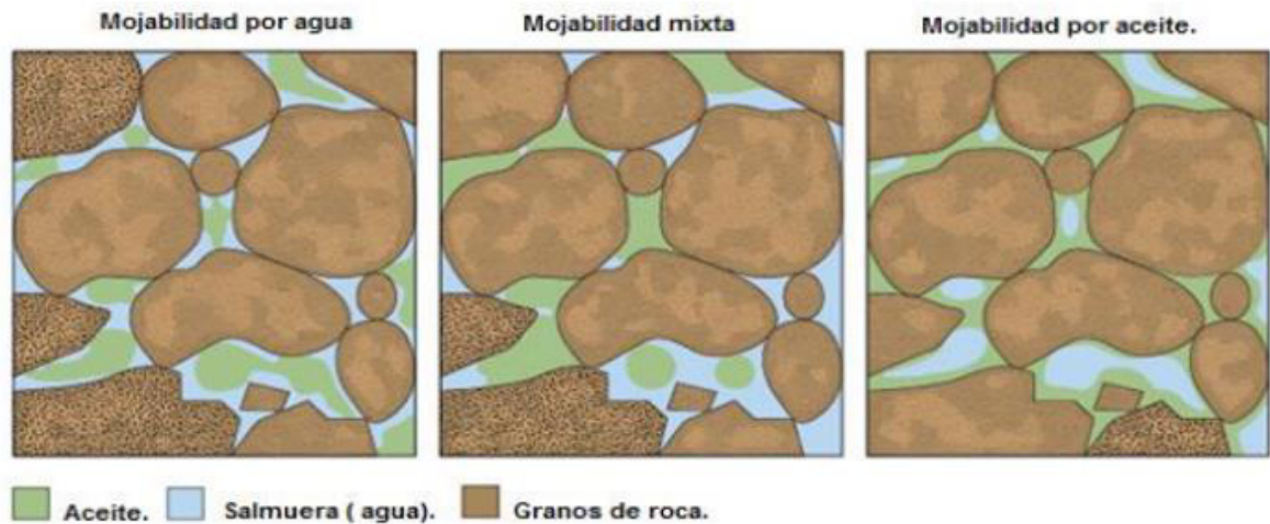
Figura 1.10. Tipos de mojabilidad roca/crudo/agua [Slumberger oilfield glosasary, 2007]
