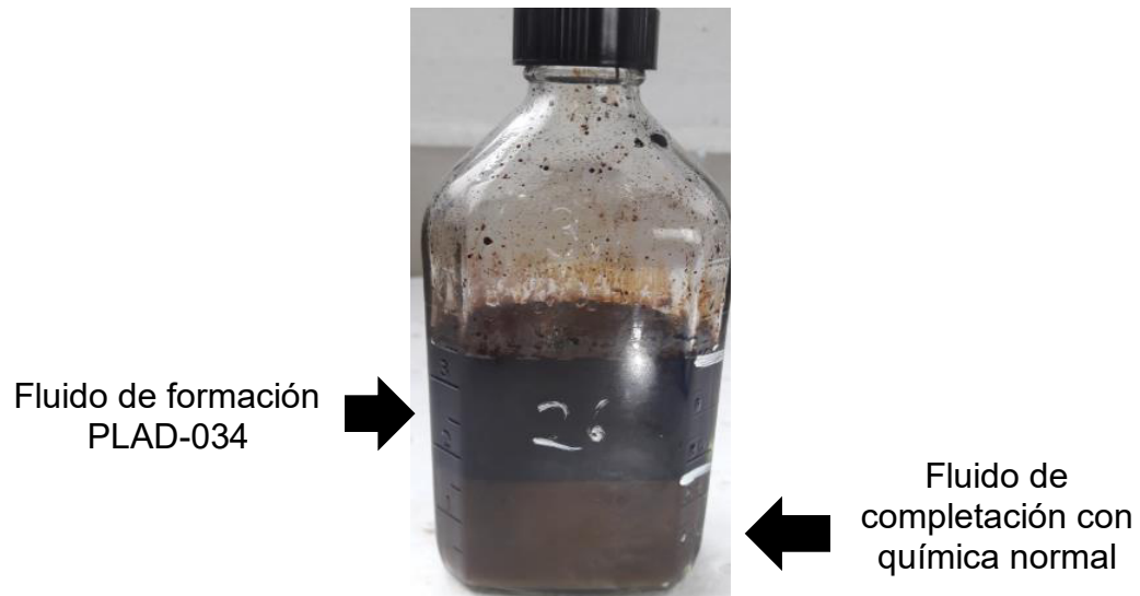
Figura 3.10. Resultado de la mezcla prueba 26 del PLAD-034 [Dynadrill S.A., 2018]
