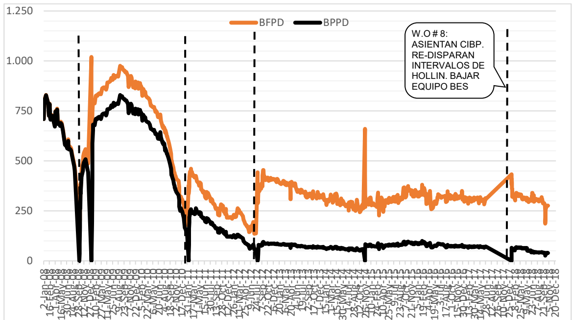
Figura 3.1. Historial de producción pozo Palo Azul-06 [Petroamazonas E.P., 2018]
