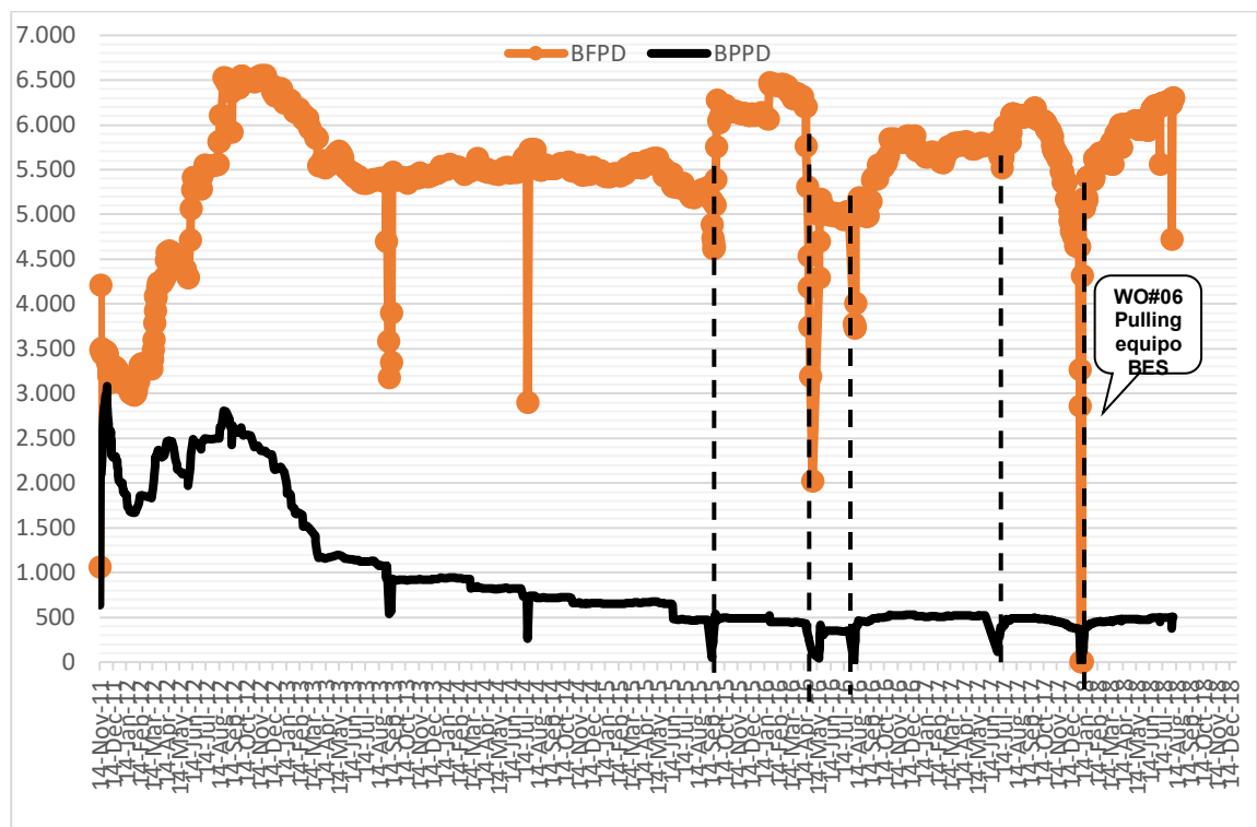
Figura 3.3 Historial de producción pozo Palo Azul-033H [Petroamazonas E.P., 2018]
