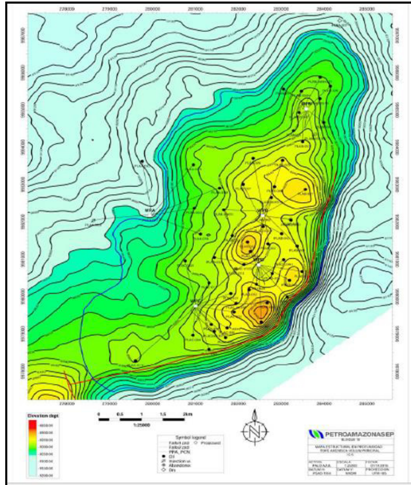
Figura 1.3. Mapa estructural del Bloque 18-Palo Azul [Petroamazonas EP, 2018]
