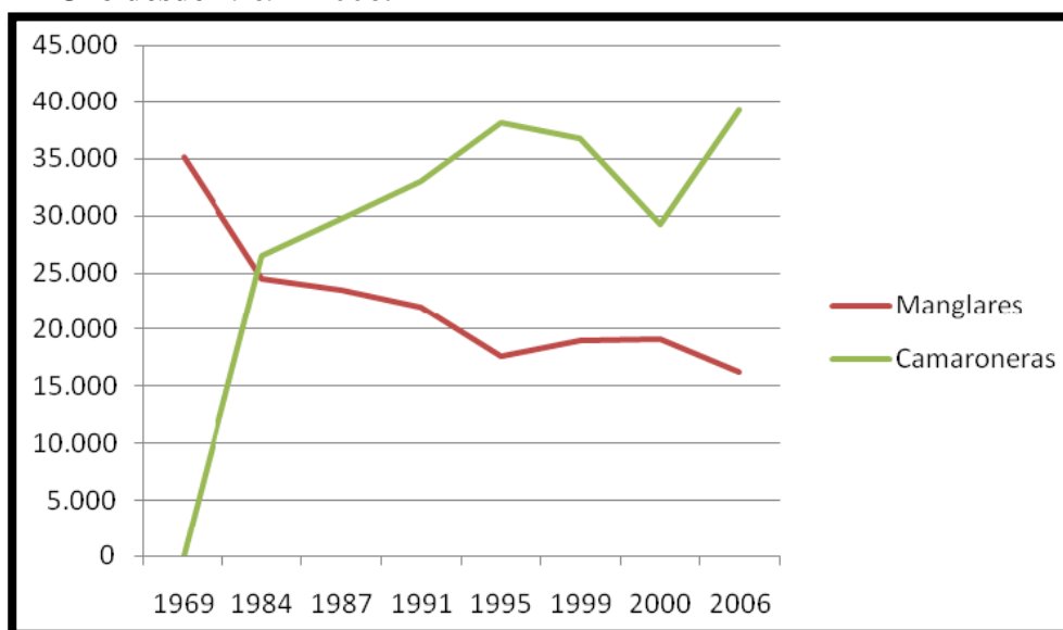
Figura # 38. Evolución de cobertura del manglar y camaroneras en El Oro desde 1969 - 2006.
