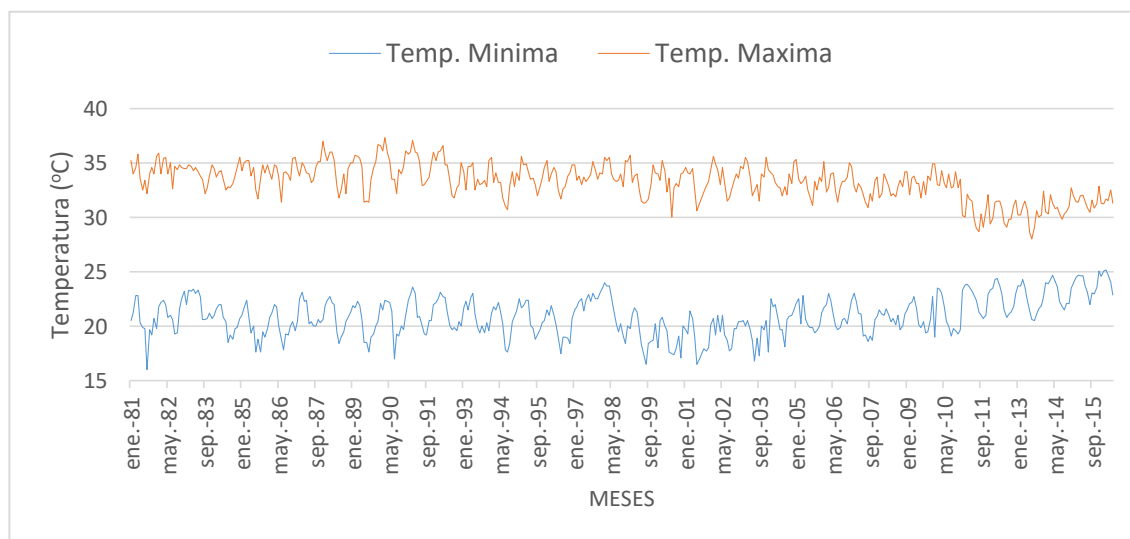
Gráfico 1. Temperatura (°C), del DAC- GUAYAQUIL (1981 -2016)
