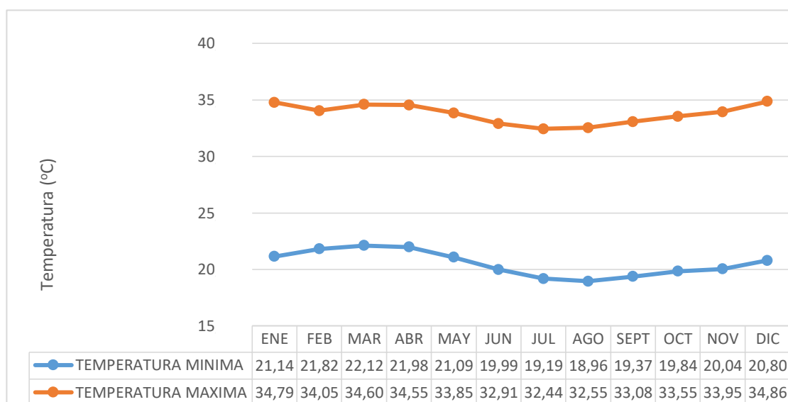
Gráfico 2. Temperatura Promedio mensual máxima y mensual mínima (°C) Fuente: DAC de Guayaquil 1981-2016
