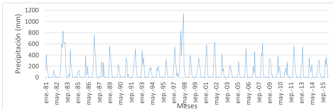
Grafico 3 . Precipitación (mm) (1981 - 2016) Fuente: DAC de Guayaquil 1981-2016
