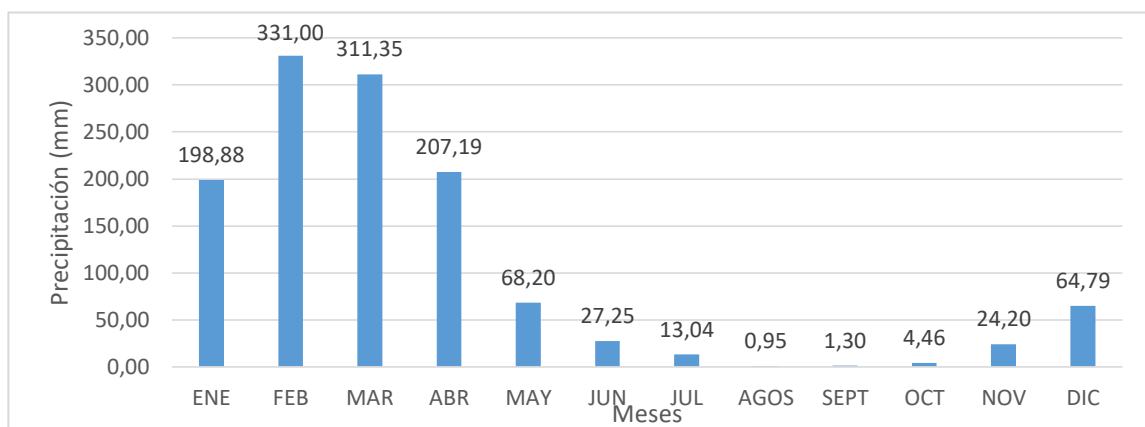
Grafico 4. Datos meteorológicos de la Estación DAC. Precipitaciones Promedio mensual desde 1981 al 2014. Fuente: DAC de Guayaquil 1981-2016
