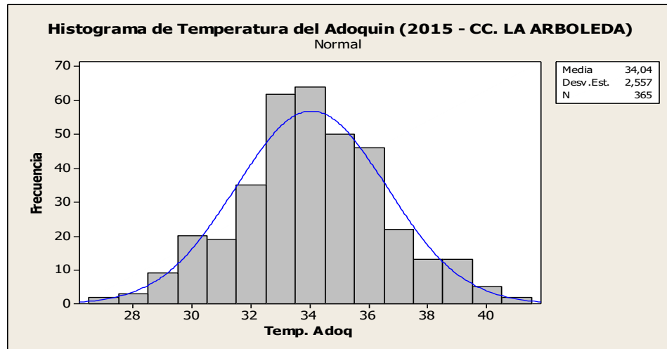
Grafico 13. Histograma de temperatura del Adoquin.
