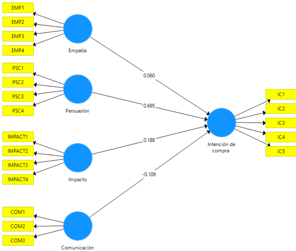
Figura 3.3 Coeficientes del modelo
