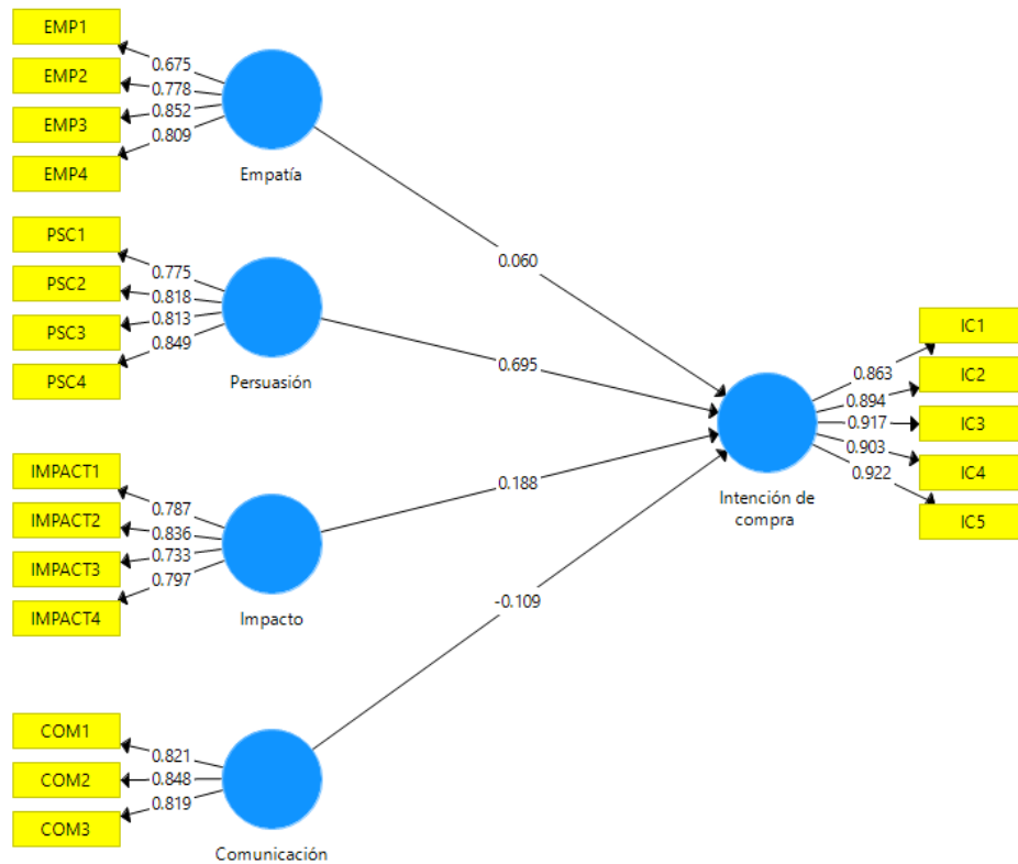
Figura 3.2 Cargas factoriales por dimensión
