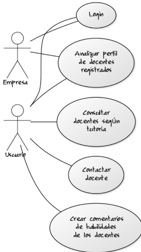
DIAGRAMA GENERAL CASOS DE USO
