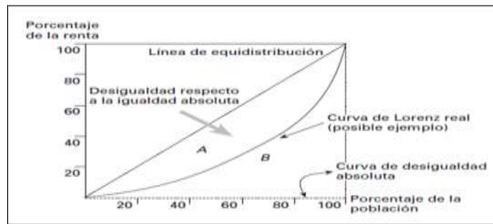
Figura 1 Curva de Lorenz
