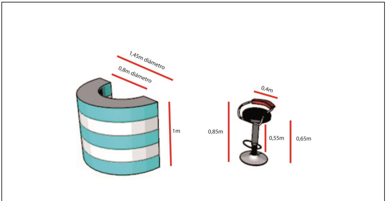
Anexos 17: Medidas counter y silla
