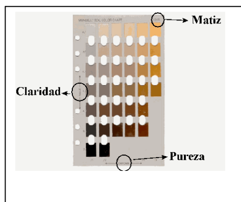
Figura 3.1 Hojas de Matices de la tabla Munsell para describir el color del suelo (modificado de Munsell Color Co., 1976).
