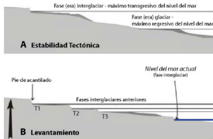
Figura 2.4 Formación de las Terrazas Marinas: (A) En una costa tectónicamente estable, las líneas de costa de las diferentes fases glaciares e interglaciares se confunden. (B) En una costa en levantamiento las terrazas creadas durante los altos niveles del mar son preservadas de la erosión marina. T1 representa la terraza más antigua (Pedoja, 2002).
