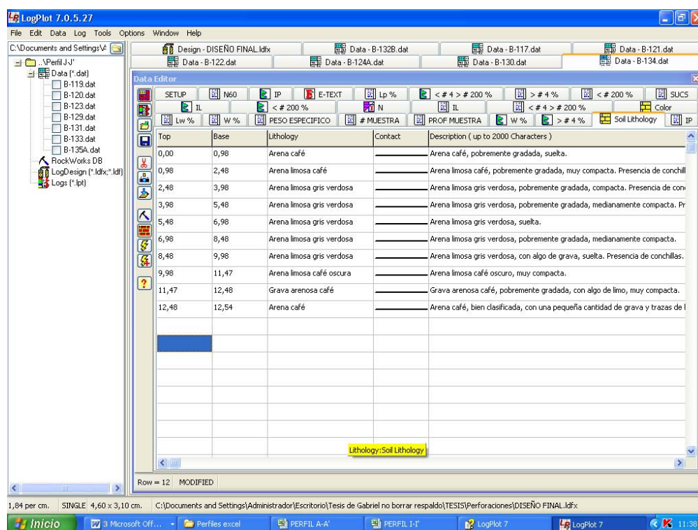
Fig. 3.7 Levantamiento de la base de datos para el Relevamiento Litológico en LogPlot 7 (RockWare Incorporad).
