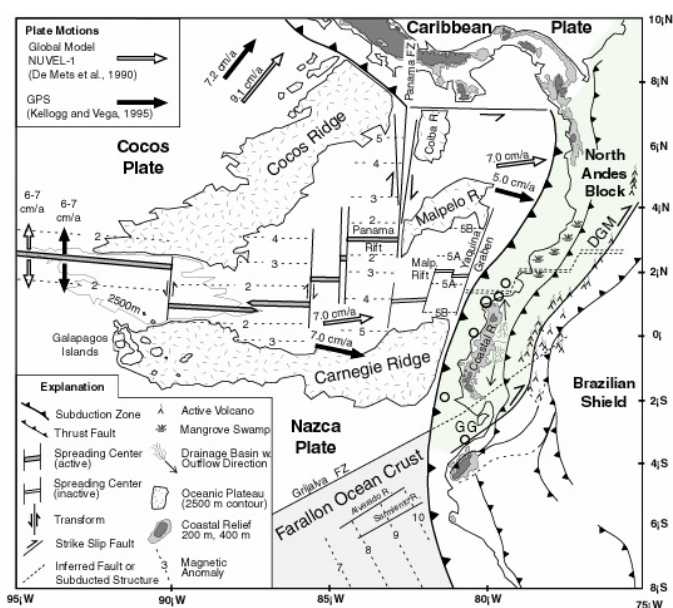
FIGURA 2.1 Contexto geodinámico y tectónico de la Margen del Ecuador y Norte de Perú (Gutscher et al , 1999)
