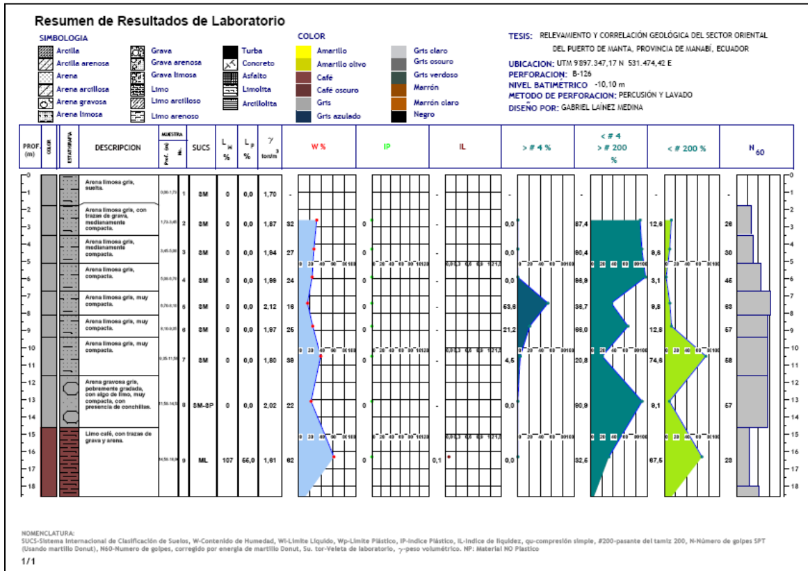
Sondeo B-126 (1/1)
