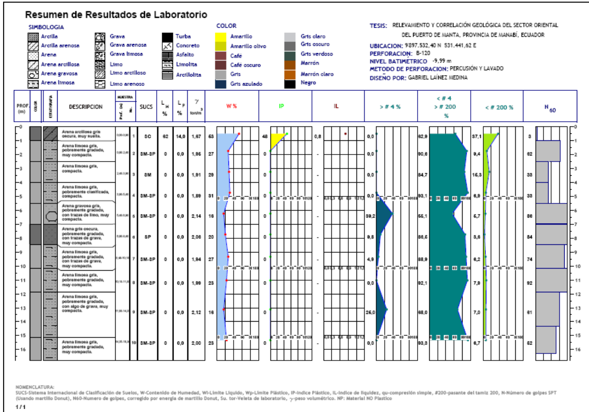
Sondeo B-120 (1/1)
