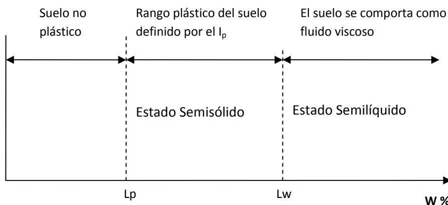
Figura 3.4.- Localización relativa de los límites plástico y líquido sobre la escala de contenido de humedad.
