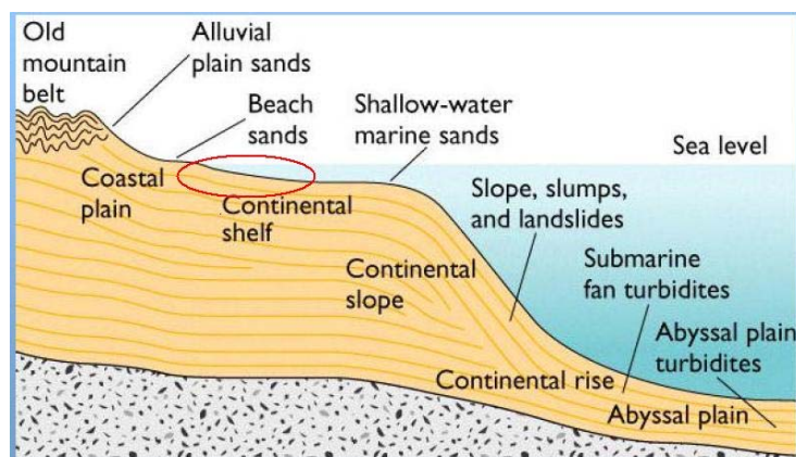
Fig. 4.1 Medio o Ambiente de Plataforma interna en el que se están depositando los sedimentos en el área de estudio (tomado de: www.geofisica.unam.mx ).
