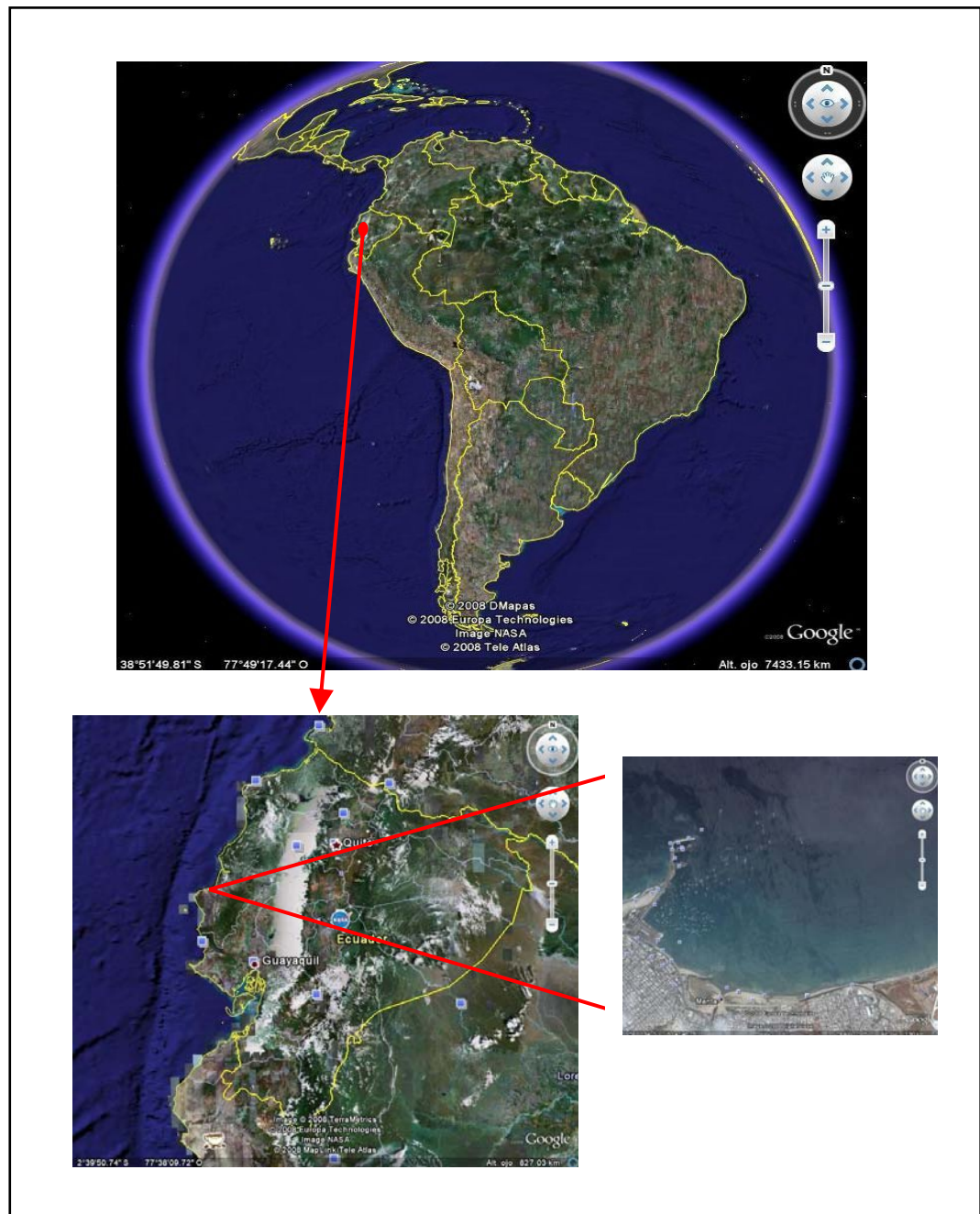
Fig.1.1 Ubicación de la zona de estudio. Imágenes NASA (tomado de Google-Earth 2008).
