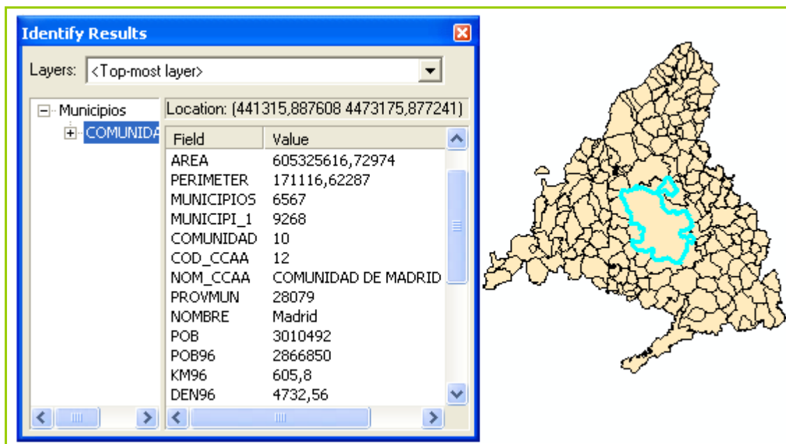
Figura 5-11: Ejemplo de consulta espacial en un SIG
