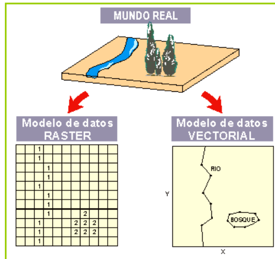
Figura 2-1: Modelos de datos raster y vectorial
