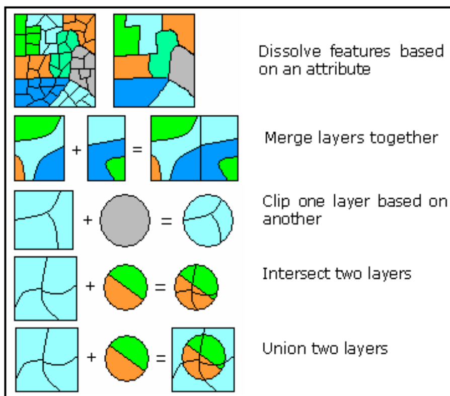
Figura 5-10: Operaciones con polígonos de GeoProcessing Wizard.
