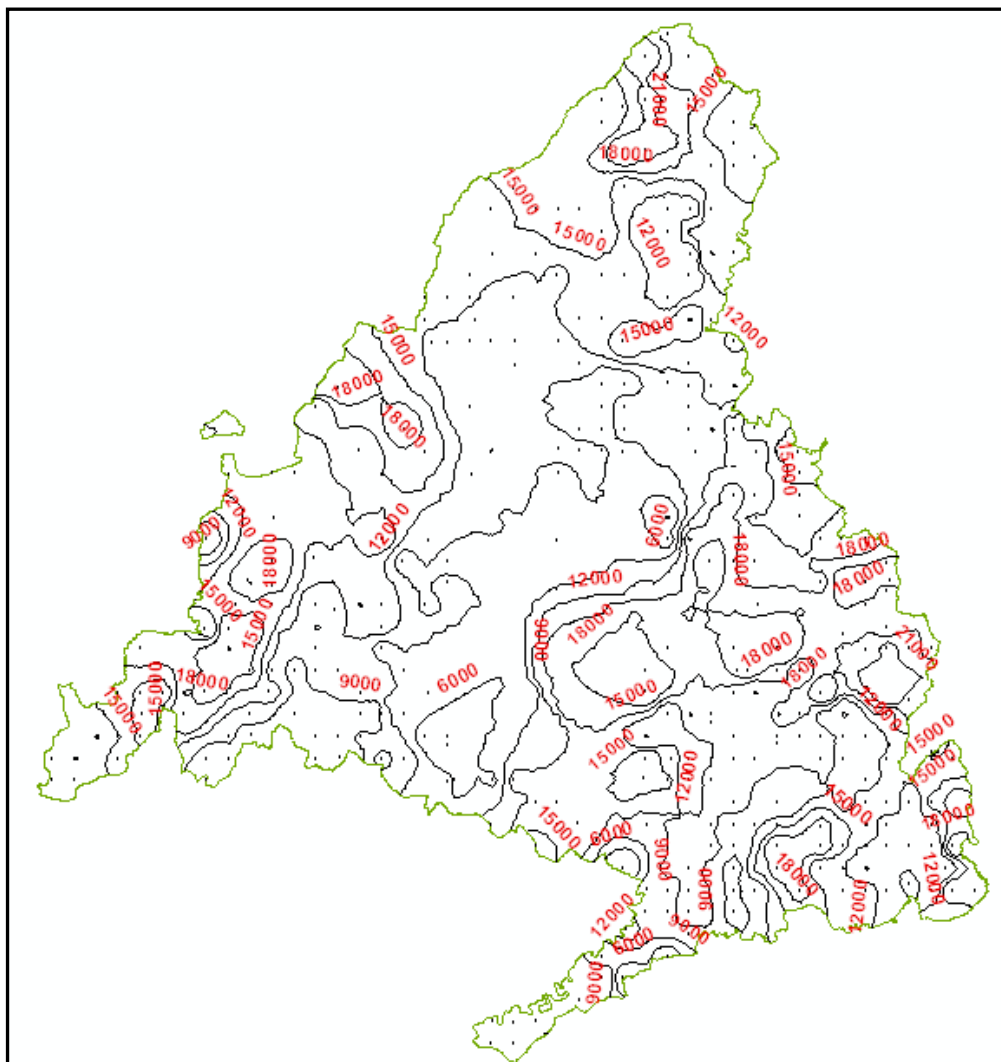
Figura 6-7: Líneas de igual concentración de Aluminio
