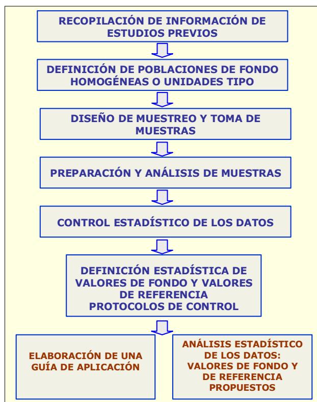
Figura 3-4: Secuencia de los trabajos realizados
