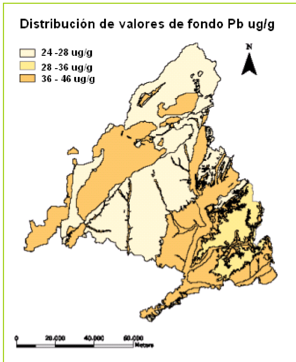
Figura 6-8: Distribución del Plomo dentro de la Comunidad de Madrid
