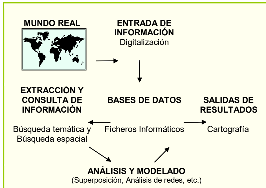
Figura 2-5: Funciones de los Sistemas de Información Geográfica
