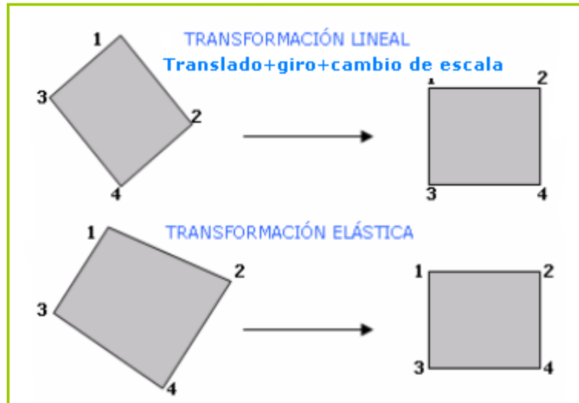
Figura 5-2: Transformación lineal y no lineal
