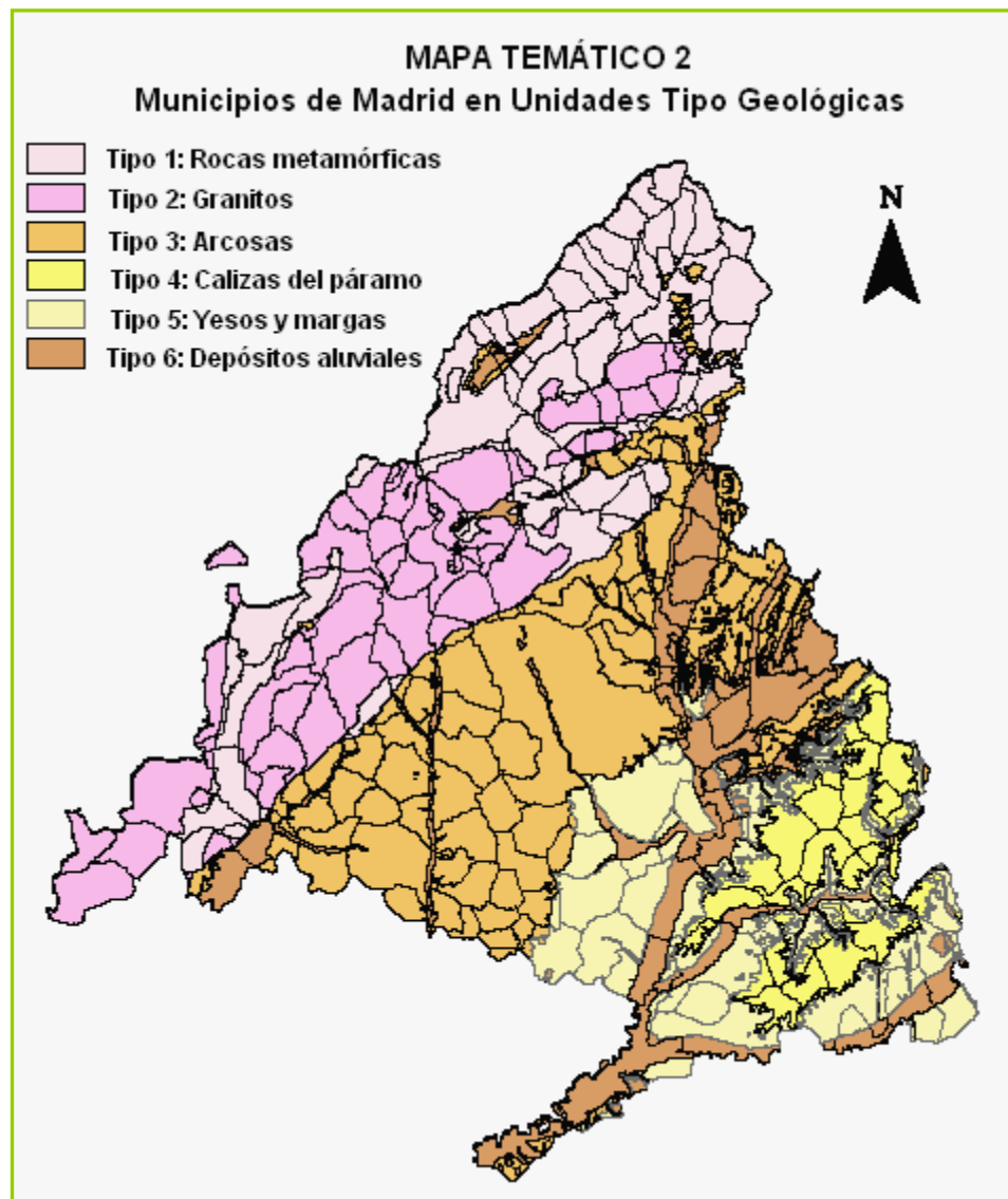
Figura 6-5: Municipios de Madrid en Unidades Tipo Geológicas
