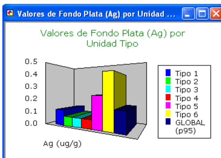
Figura 6-3: Valores de Fondo de Plata (Ag) por Unidad Tipo Geológica
