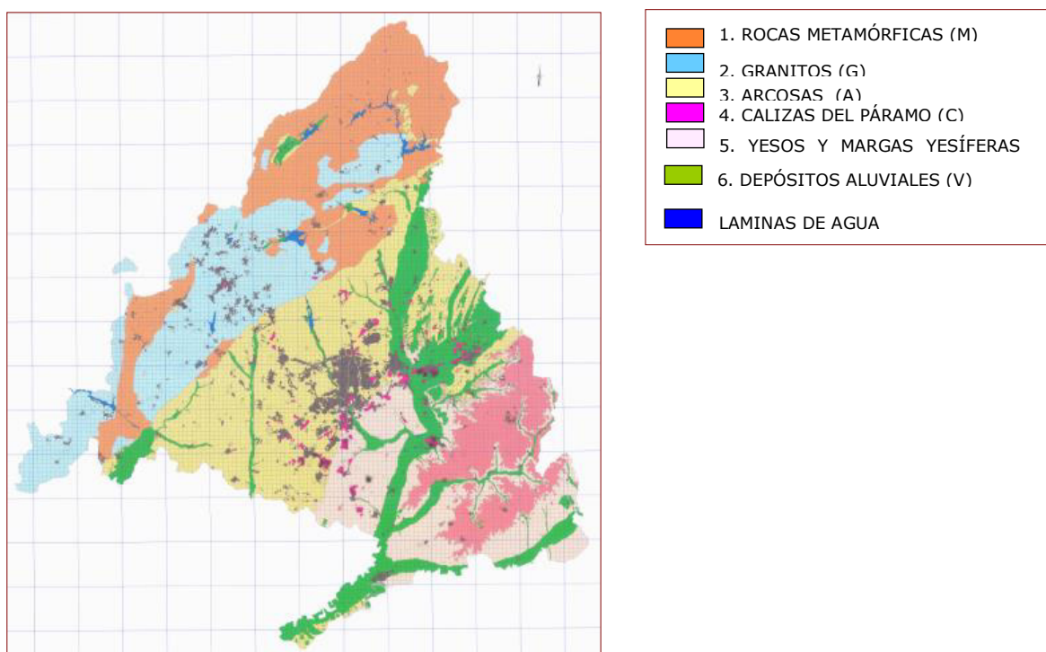
Figura 3-5: Mapa de Unidades Tipo
