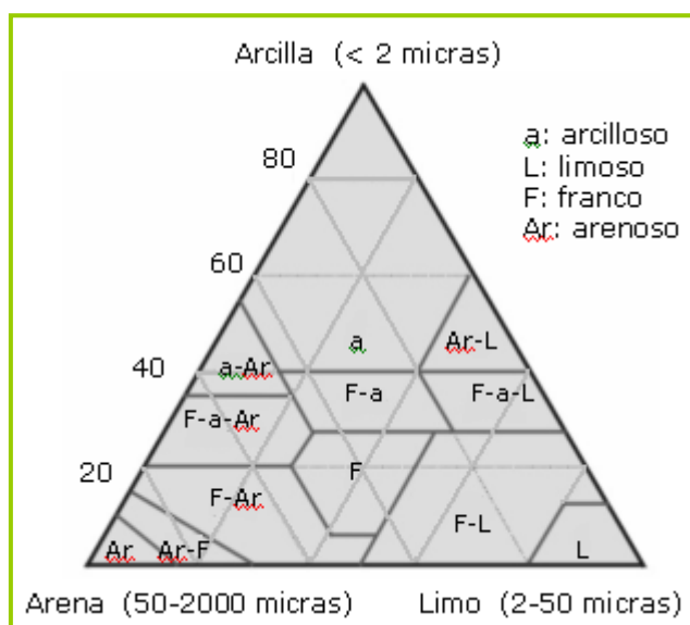
Figura 3-2: Esquema de la clasificación textural del suelo
