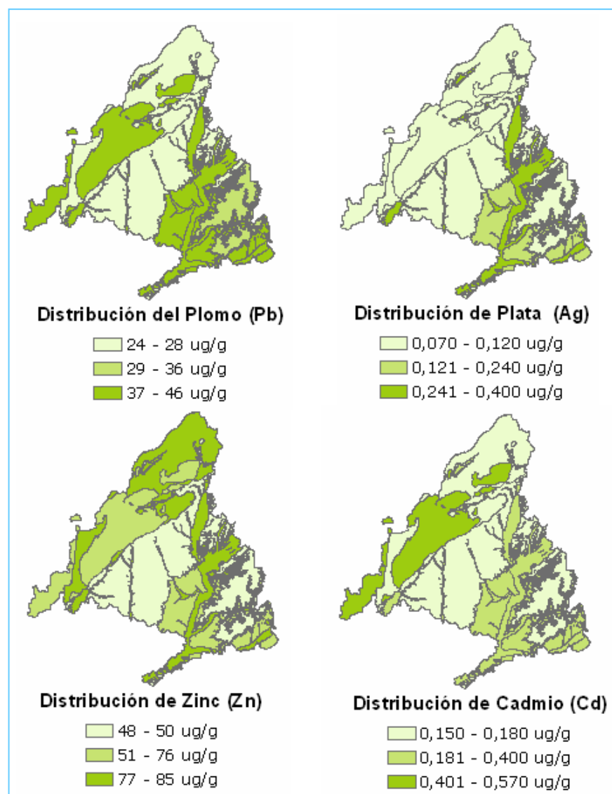
Figura 5-13: Distribución de valor de fondo de Pb, Ag, Zn y Cd
