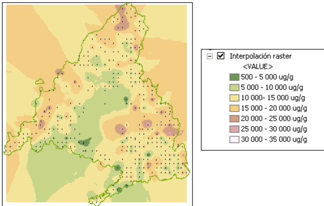
Figura 6-6: Interpolación a raster del contenido de Aluminio ( \mu\text{g/g} )
