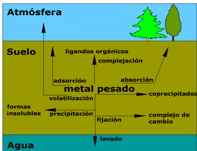
Figura 3-3: Los metales pesados incorporados al suelo
