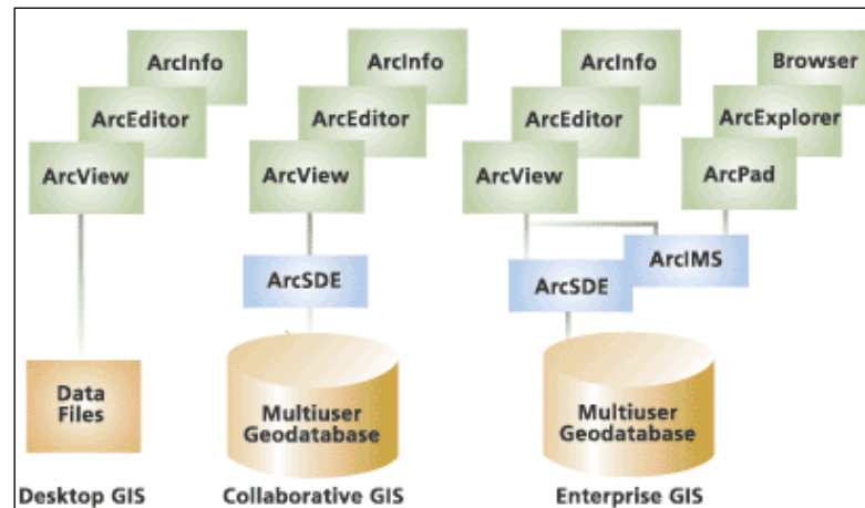
Figura 4-1: Componentes de ArcGis
