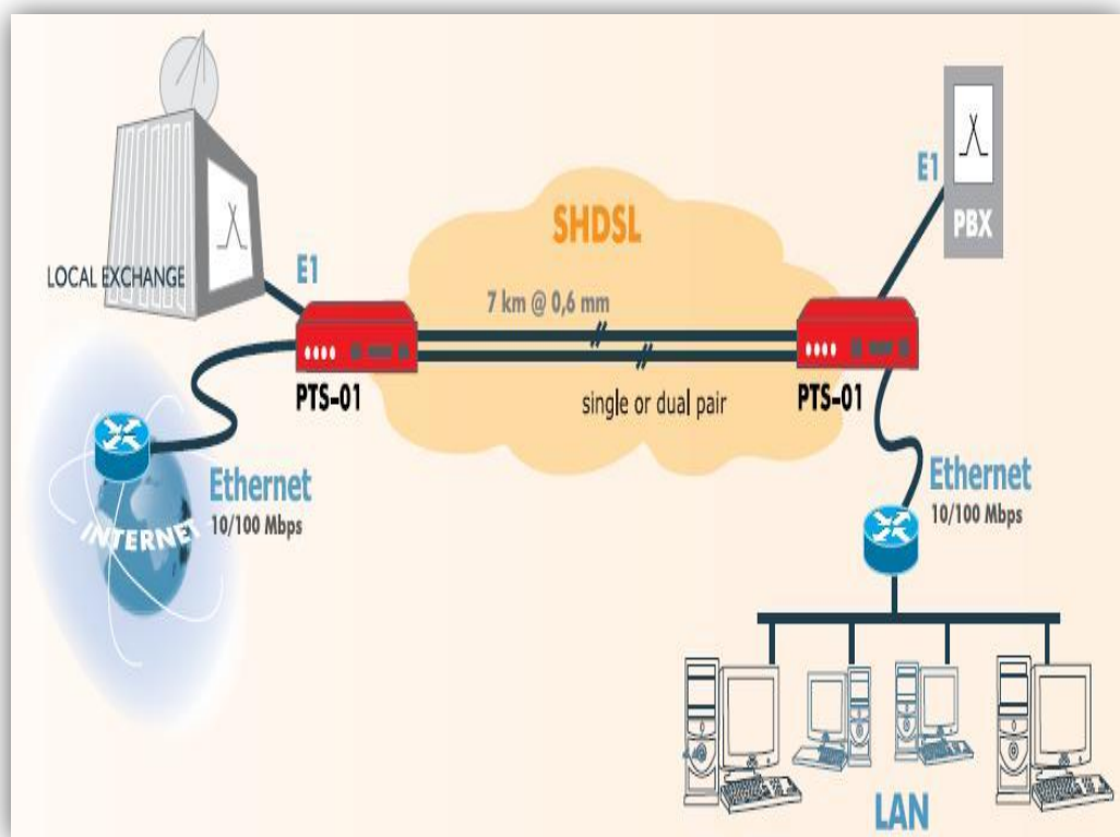
Figura 2.6 Esquema SHDSL [5]
