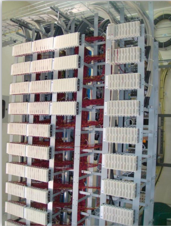
Figura 2.3 Regleta DSLAM
