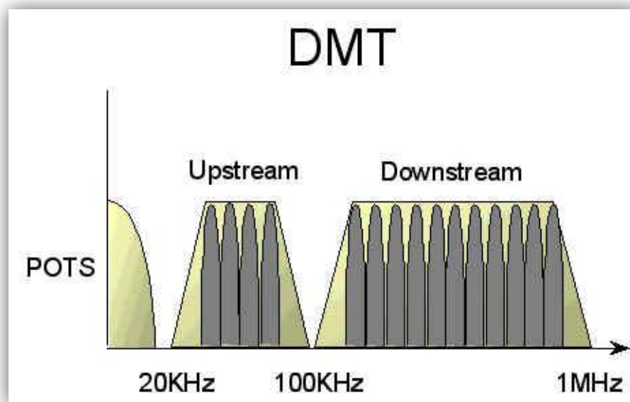
Figura 2.4 Modulación DMT [5]
