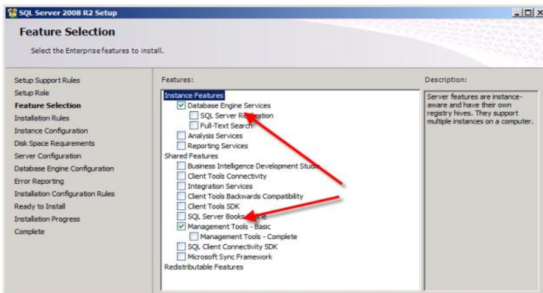
FIG 28.- INSTALACION SQL ROLES.
