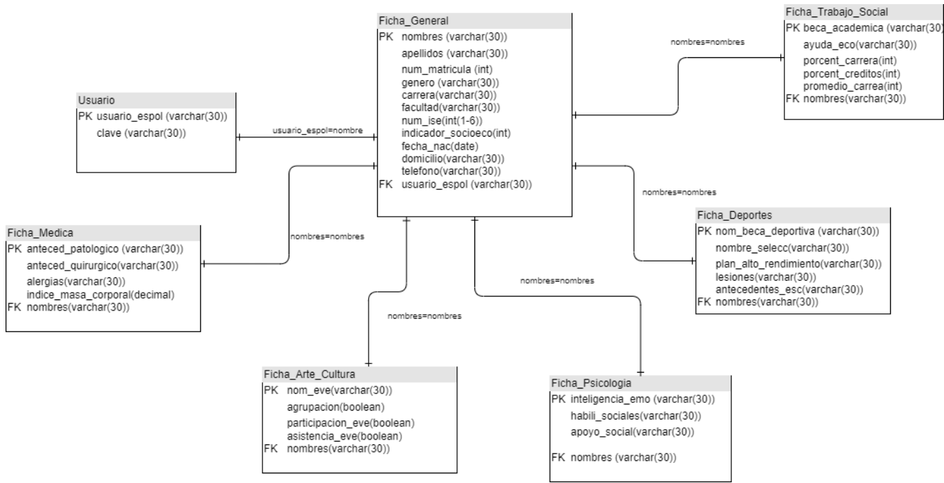
Figura 2.12 Diagrama de la Base de Datos [Autoría Propia]
