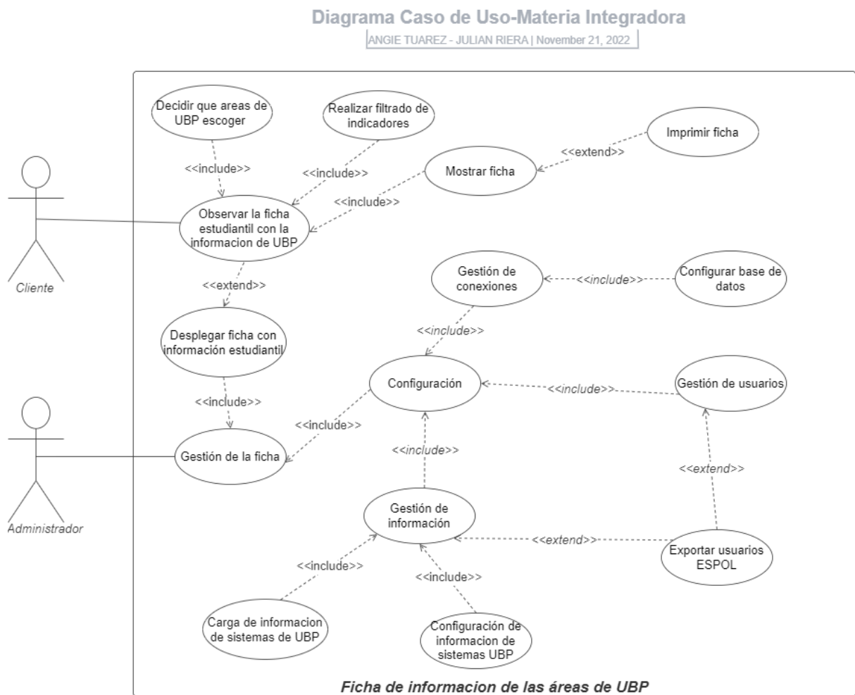
Figura 2.10 Diagrama de Caso de Uso [Autoría Propia]
