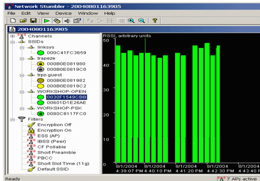
Figura 7.7. Herramienta de monitoreo Network Stumbler.
