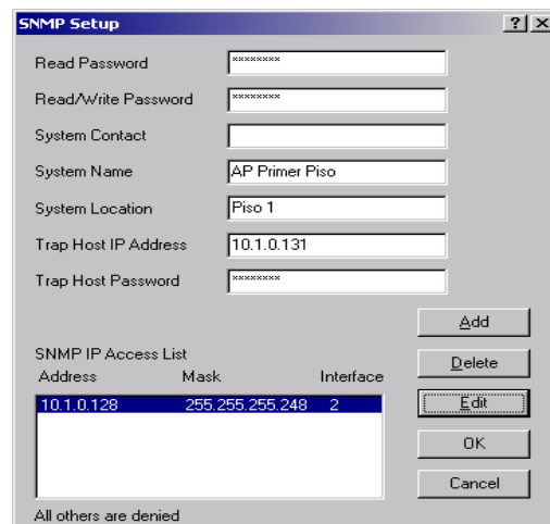
Figura 7.4. Configurando la Seguridad SNMP.
