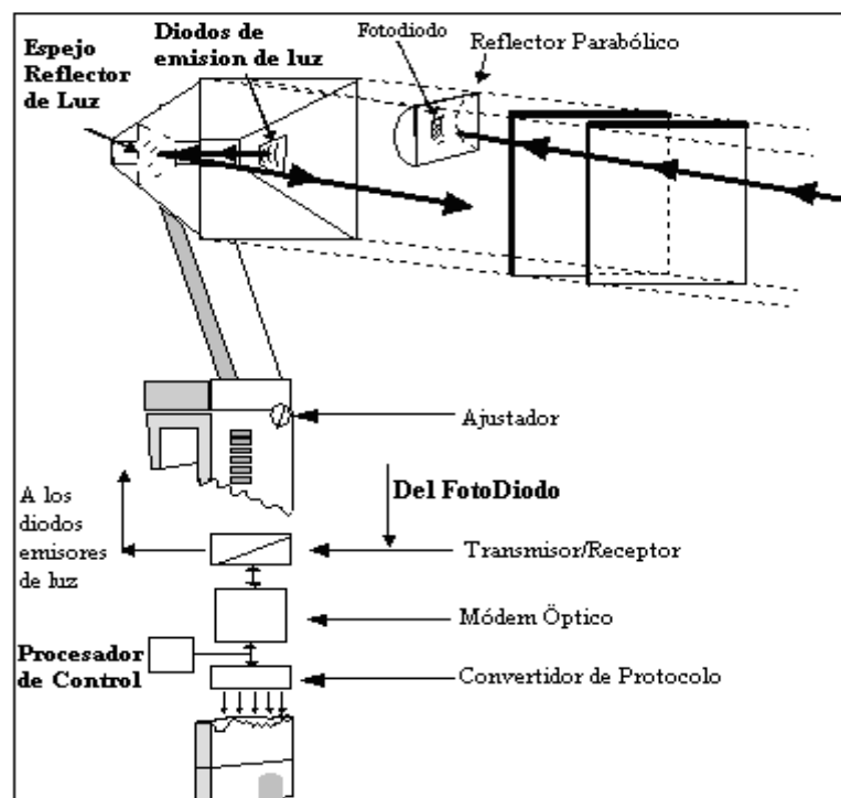
Figura 2.5. Transreceptor infrarrojo.
