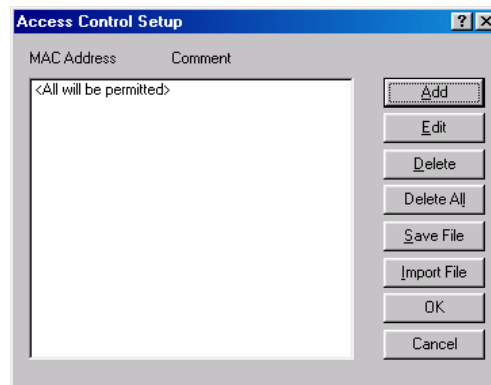
Figura 7.2. Control de Acceso por direcciones MAC
