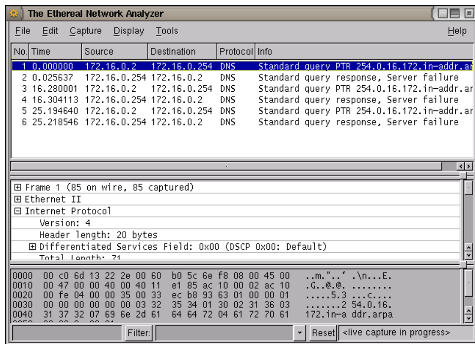
Figura 7.5. Herramienta de monitoreo Ethereal.
