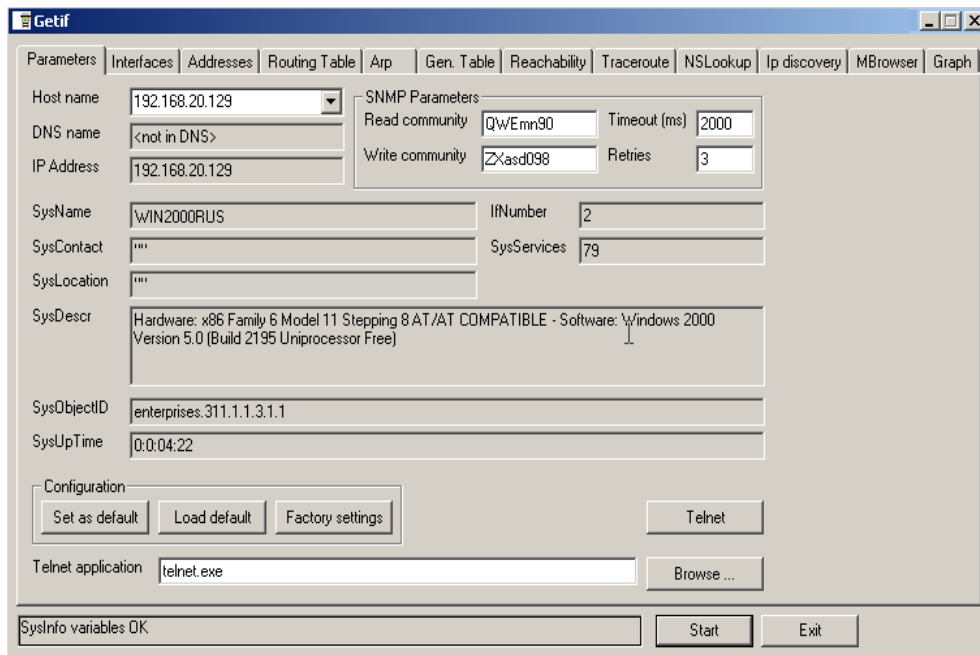
Figura 7.6. Herramienta de Monitoreo Getif.
