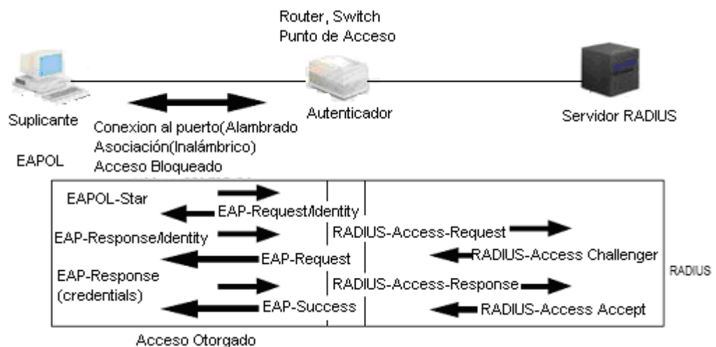
Figura 5.5. Diálogo EAPOL-RADIUS.
