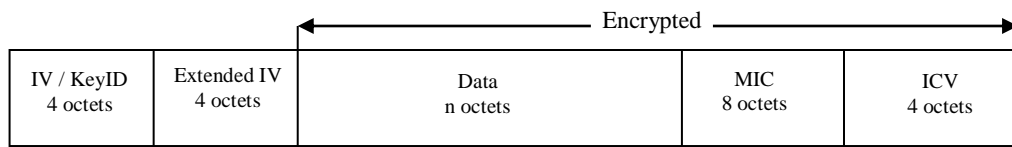
Figura 5.6. Estructura de encriptación de TKIP.
