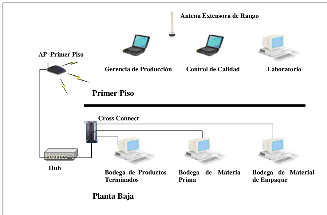
Figura 8.3. Diseño de la WLAN - LAN cableada.
