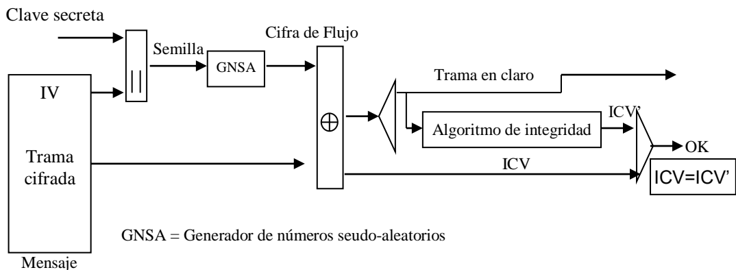
Figura 5.2. Funcionamiento algoritmo WEP en modalidad de descifrado.
