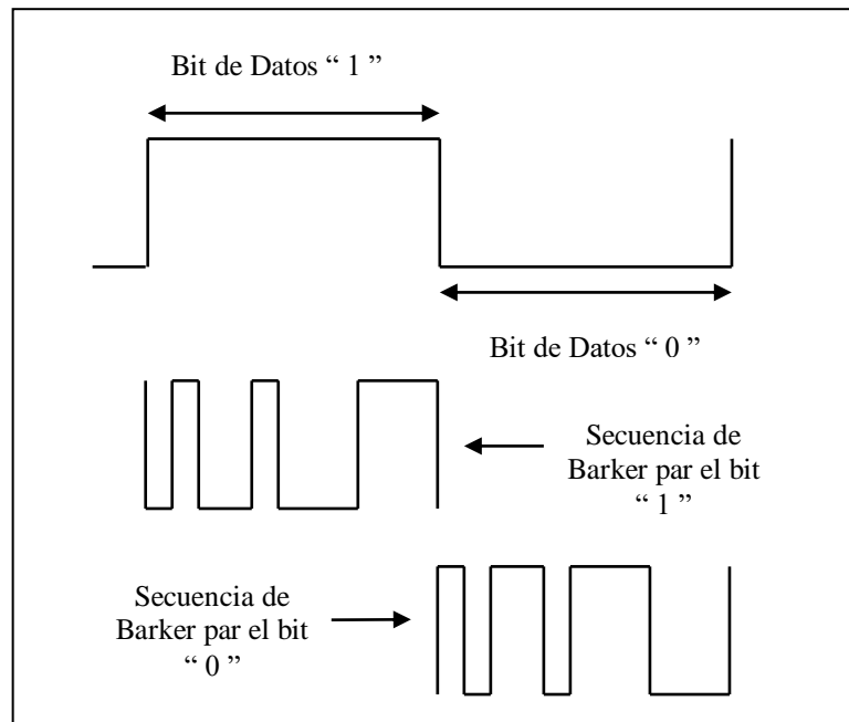
Figura 2.2. Codificación mediante la secuencia de Barker.
