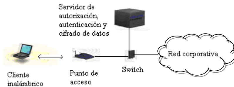
Figura 5.3. Estructura de una VPN para acceso inalámbrico seguro.
