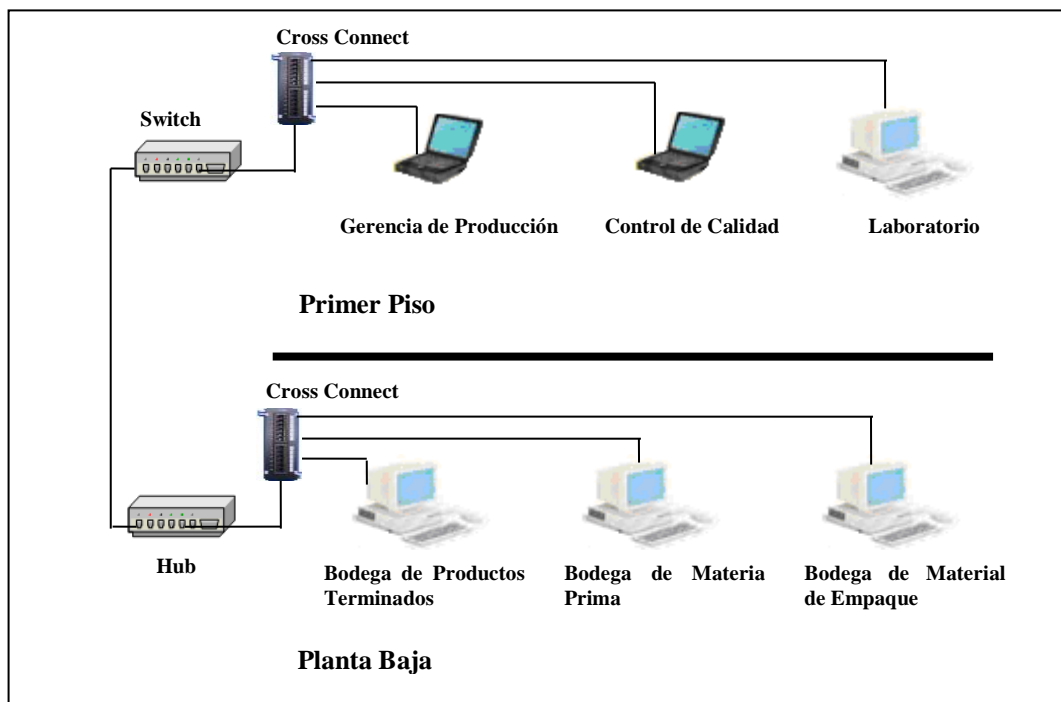
Figura 8.2. Diseño de la LAN cableada.
