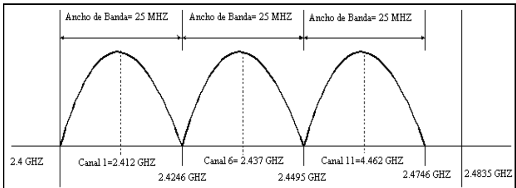
Figura 2.3. Operación de 3 canales independientes DSSS.
