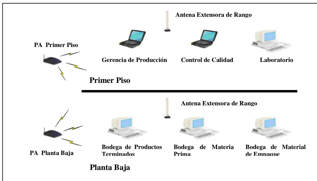
Figura 8.1. Diseño de la WLAN.
