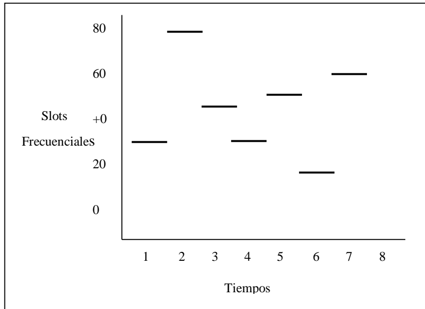
Figura 2.4. Modo de trabajo de la técnica FHSS.
