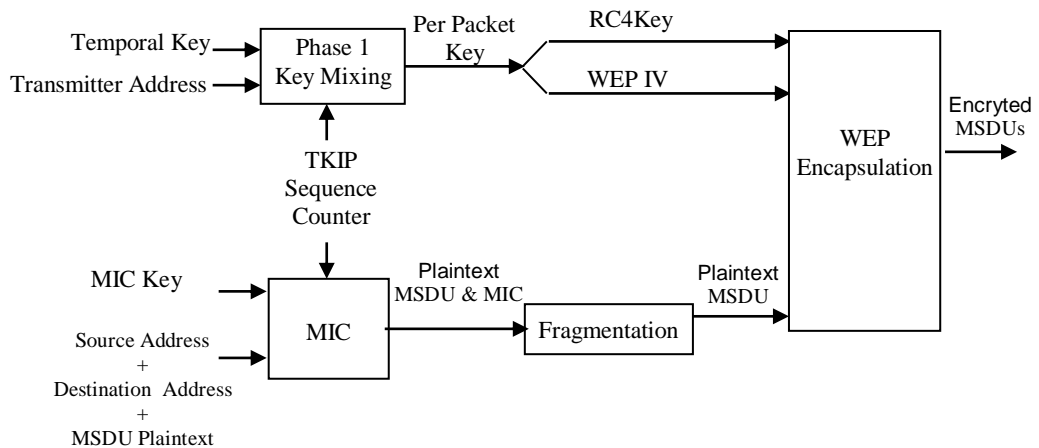
Figura 5.7. Proceso de encapsulación TKIP.
