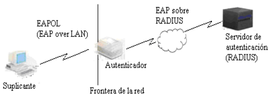
Figura 5.4. Arquitectura de un sistema de autenticación 802.1x.
