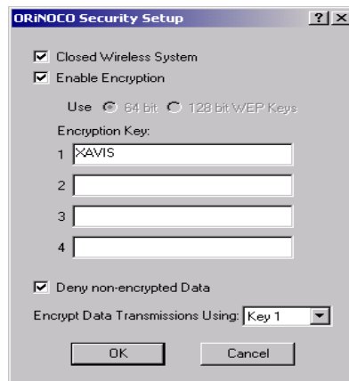
Figura 7.3. Configurando la Encriptación
