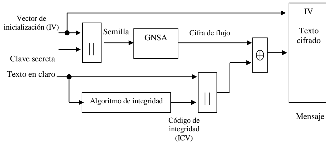
Figura 5.1. Funcionamiento del algoritmo WEP en modalidad de cifrado.
