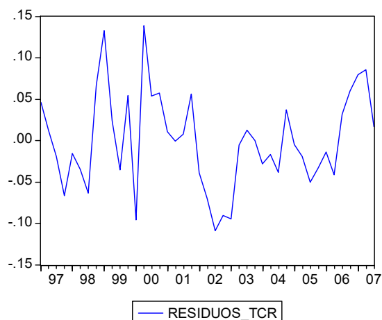
Gráfico 9: Residuos Tipo de Cambio Real
