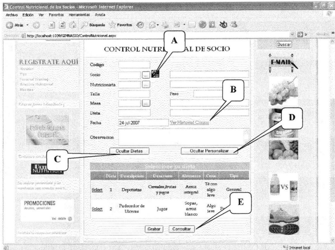
Figura 6.16 Página Proceso Control Nutricional de socio.
