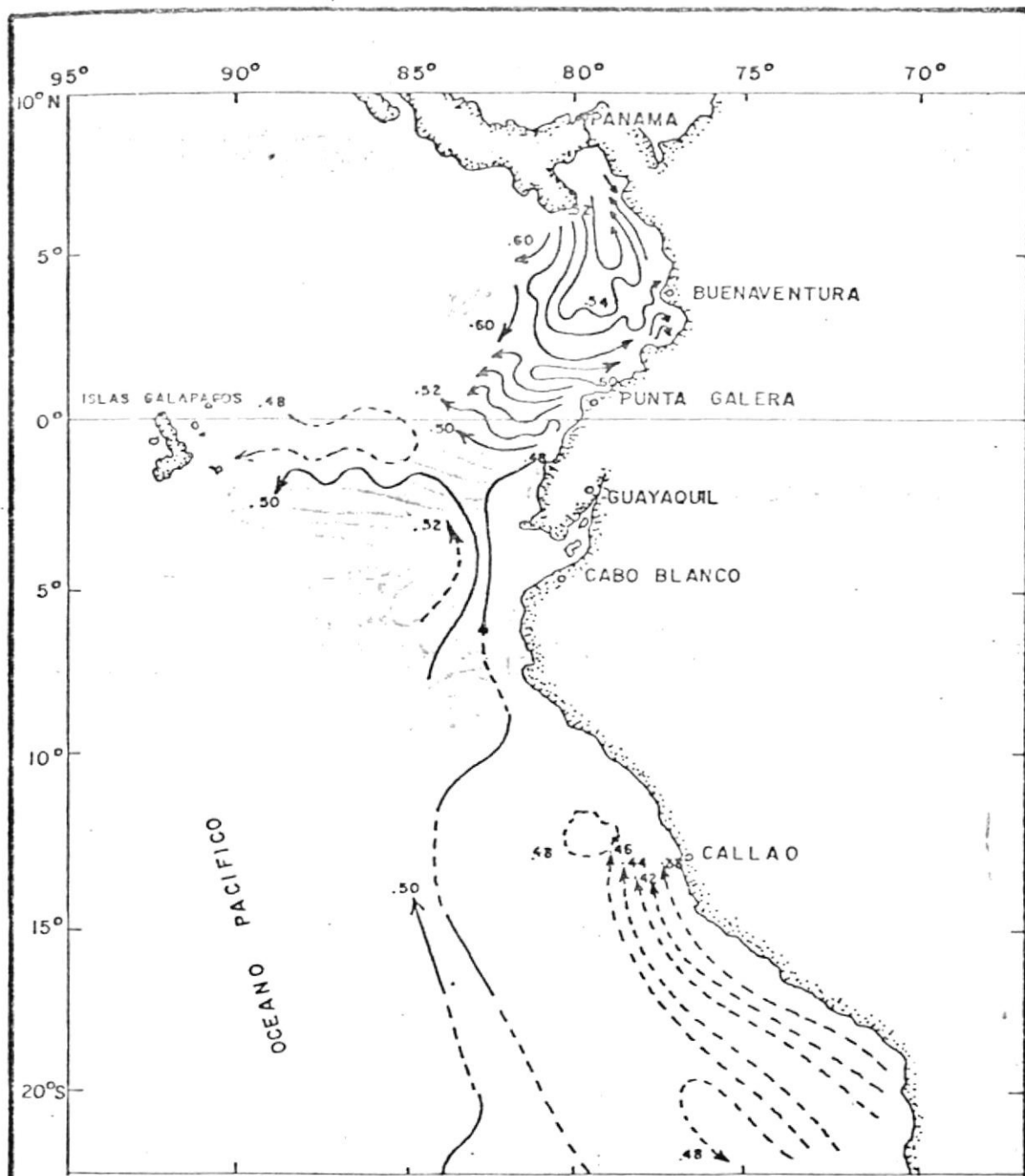
FIG. N° 7 .—— CIRCULACION SUPERFICIAL PROMEDIO ( m/seg) FRENTE A SUDAMERICA EN FEBRERO - MARZO
