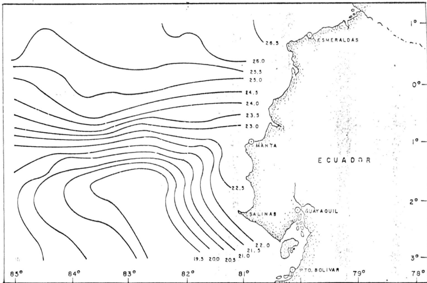
FIG. N° 9.- ESTRUCTURA TIPICA DEL FRENTE ECUATORIAL.
