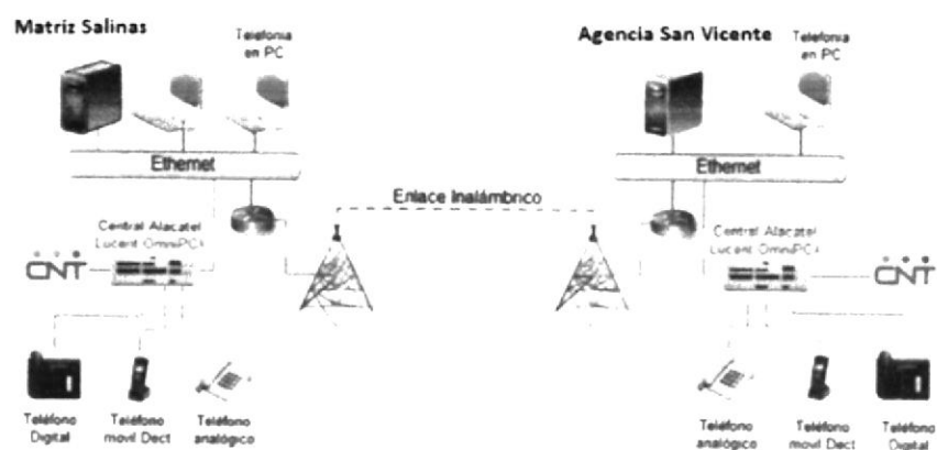
Gráfico 04.- Futura conexión entre las centrales
