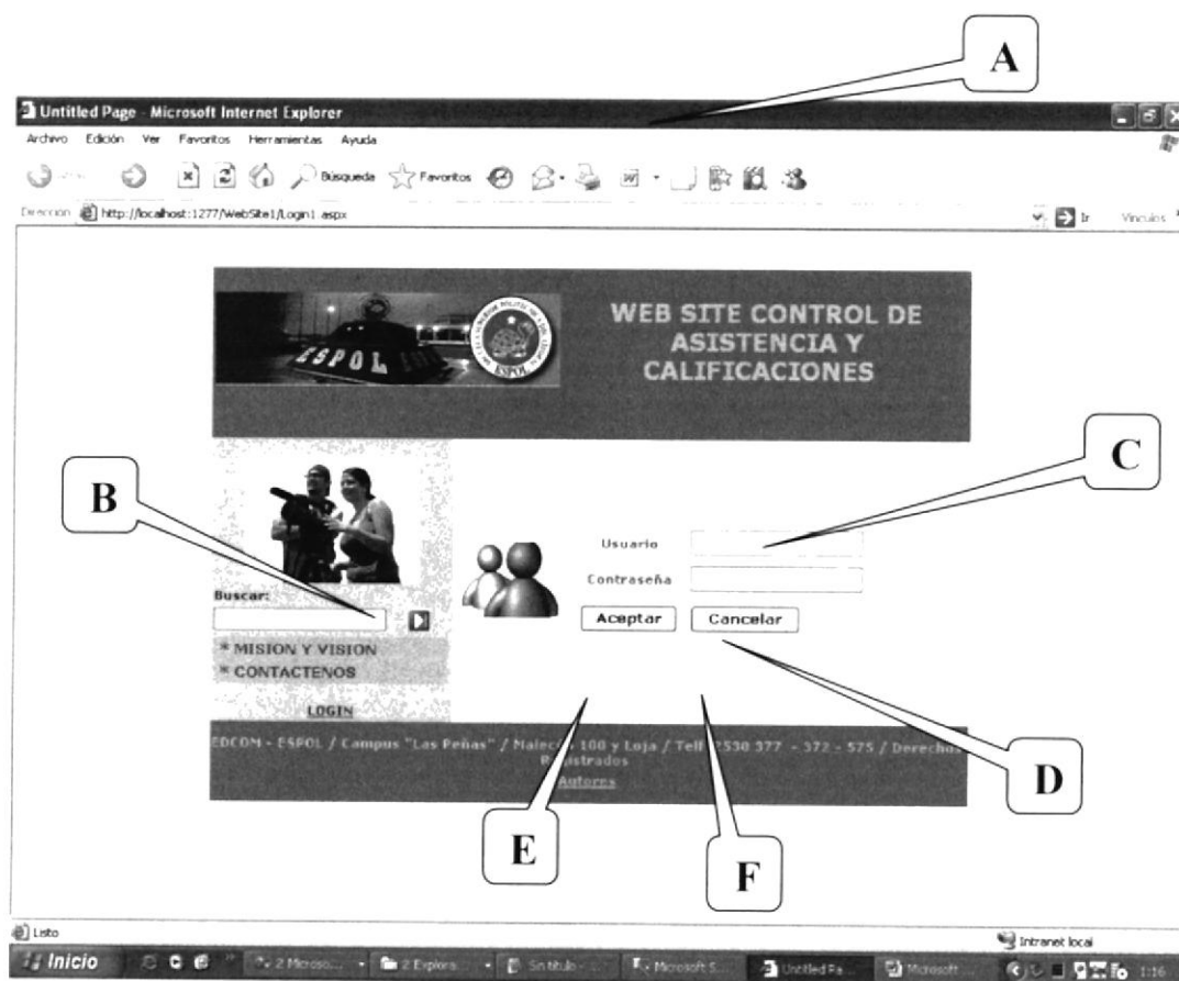
Figura 27. Login
