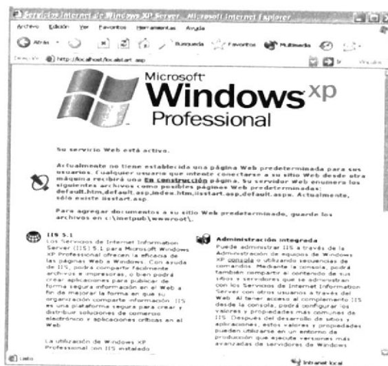
Figura 19. LocalHost
