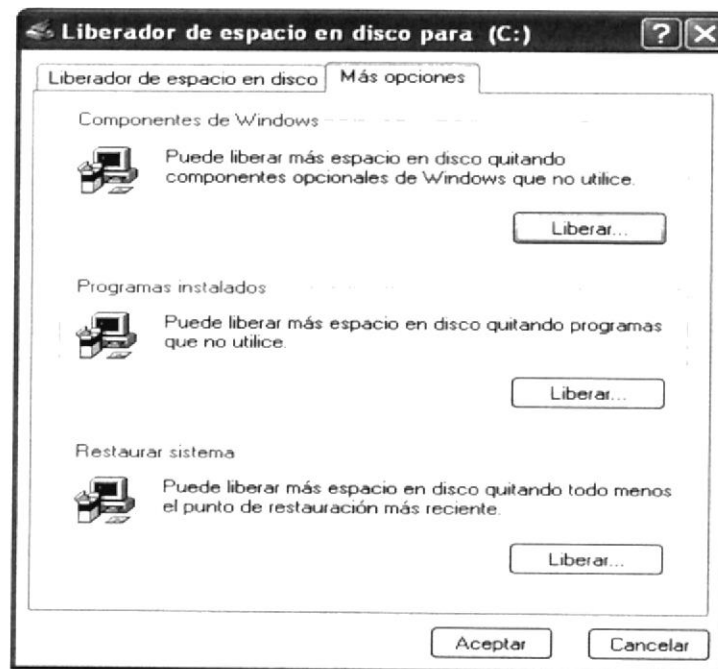
Figura 12. Más opciones
