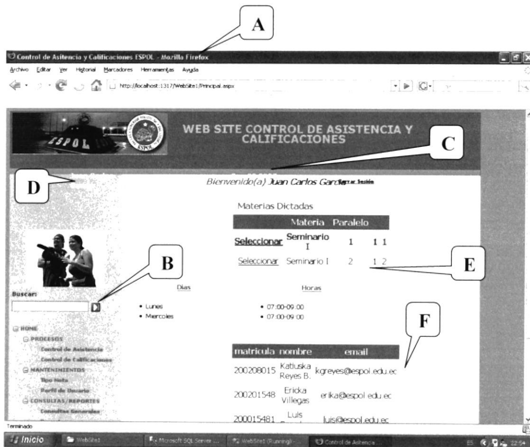
Figura 26. Página principal
