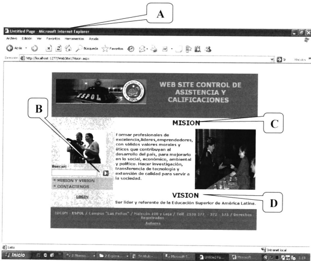
Figura 28. Página Visión
