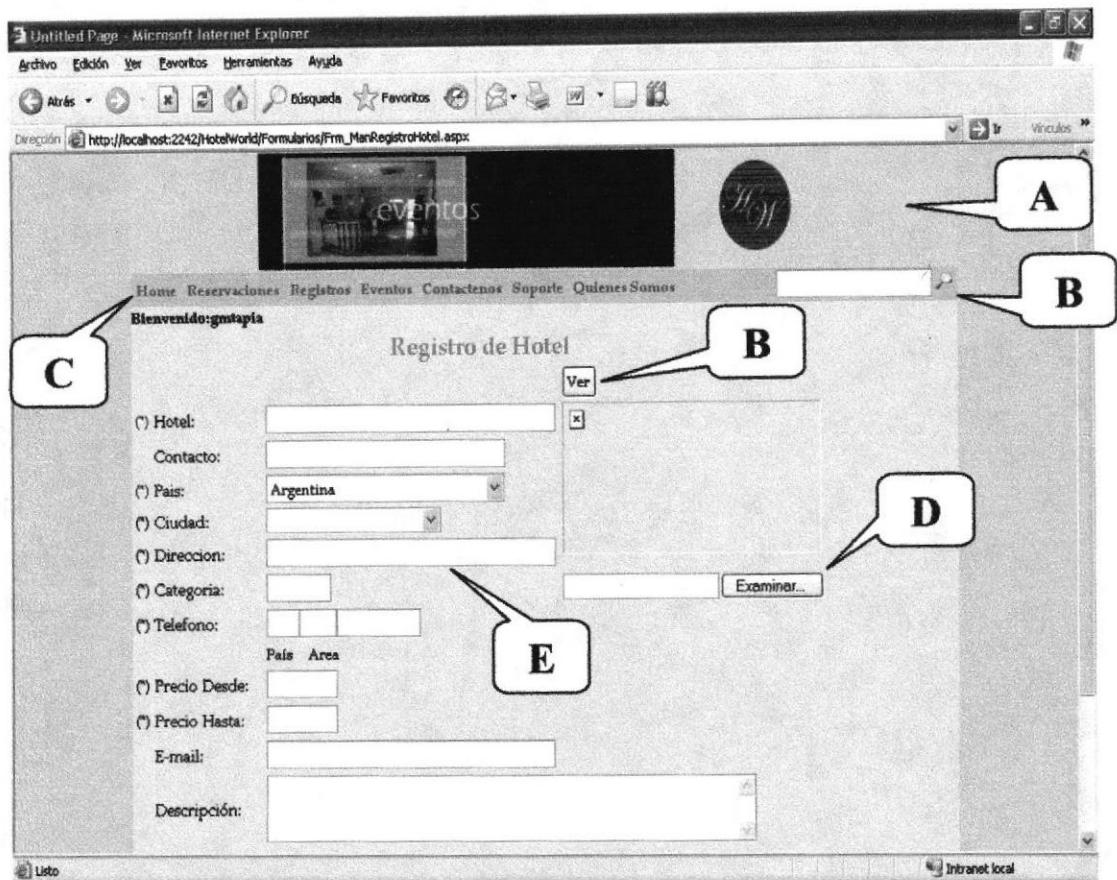
Figura 6.5.3 Página de Registro
