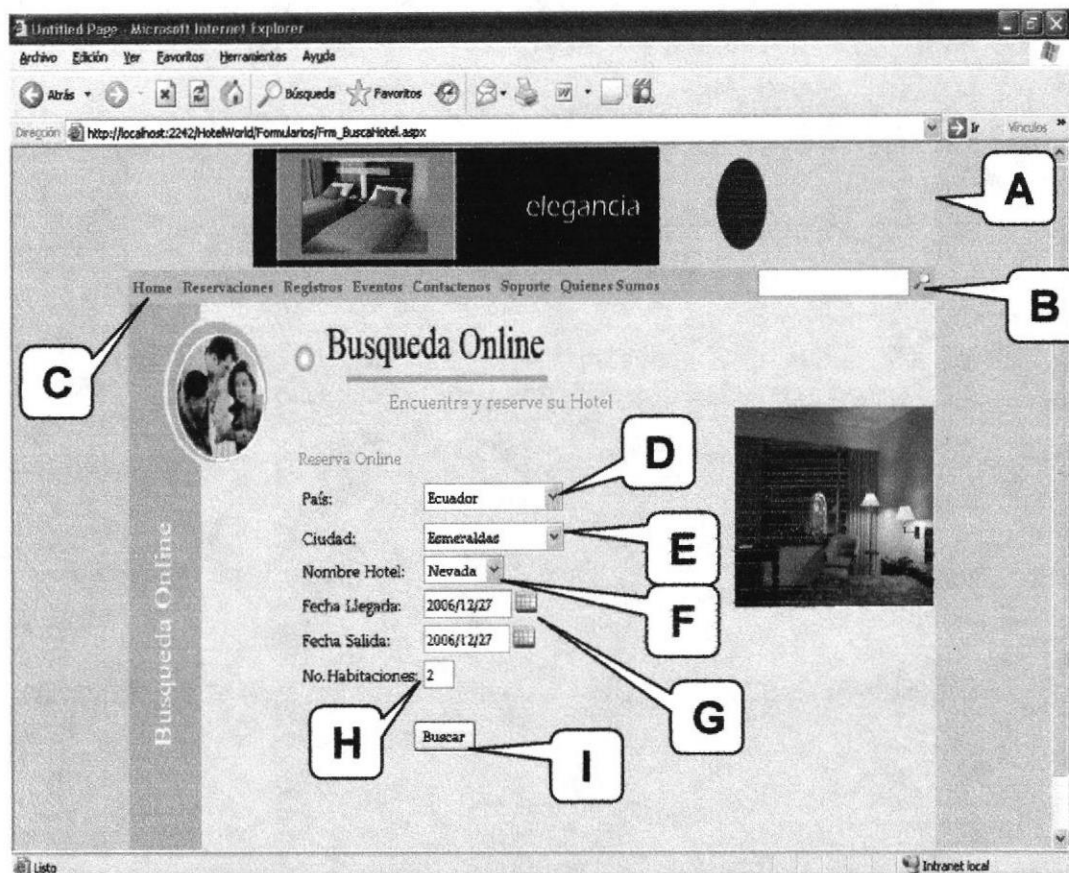
Figura 6.5.2 Página Búsqueda Online
