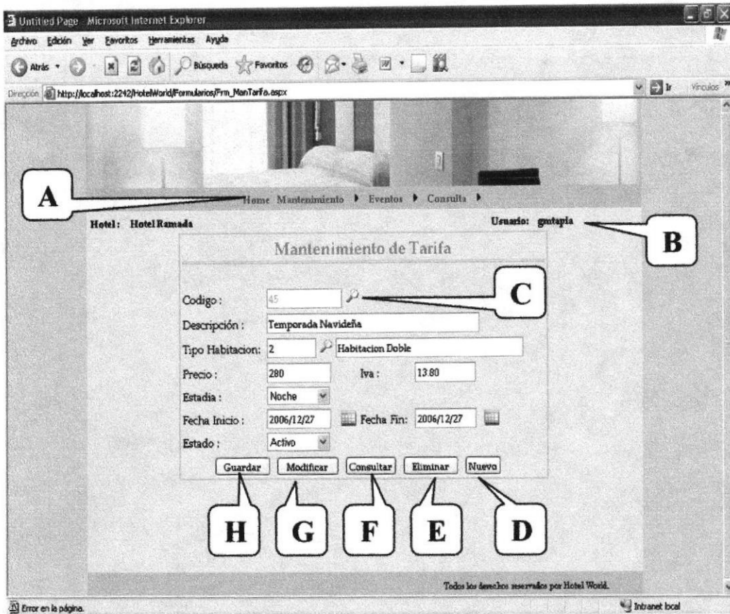
Figura 6.7.4 Mantenimiento de Tarifa.
