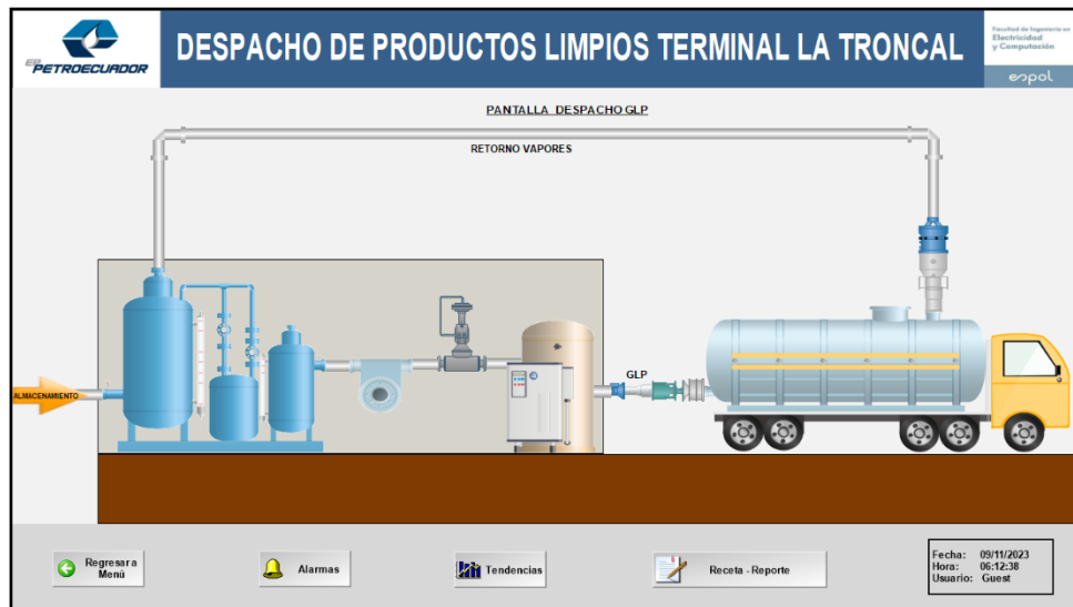
Figura 20. Pantalla Despacho GLP
