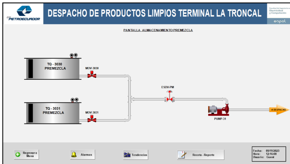
Figura 17. Pantalla Almacenamiento Premezcla
