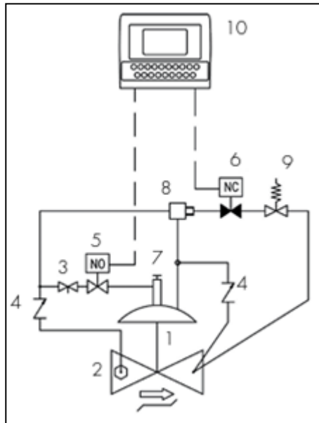
Figura 11. Esquema de control válvula de Tipo PCV autorregulable
