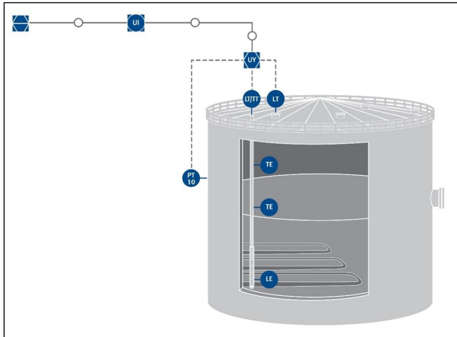
Figura 5. Esquema Integral Medición de Nivel Termina La Troncal
