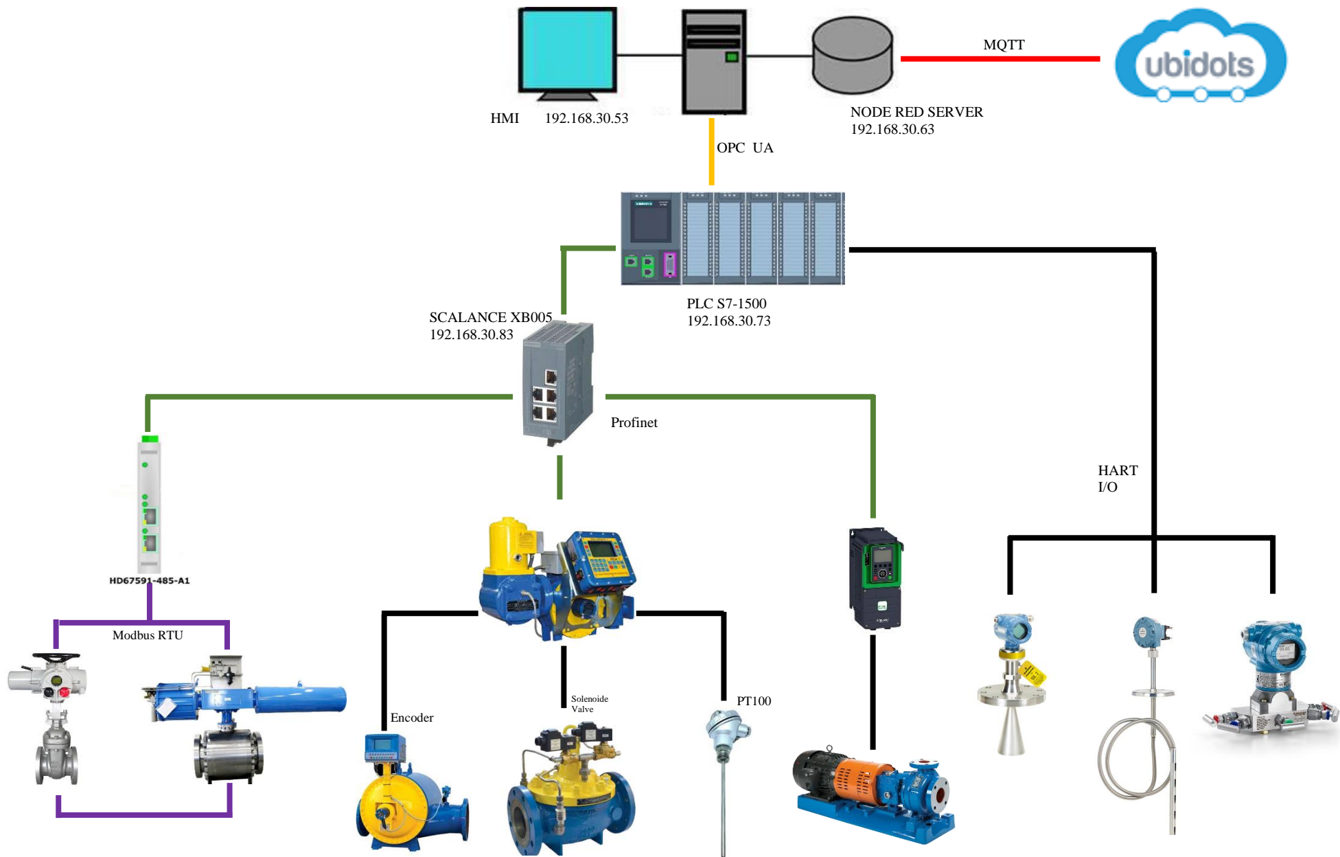
Figura 13. Topología de Red Integral del Sistema de Control
