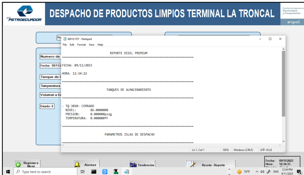
Figura 23. Pantalla de visualización e impresión de reporte de operaciones en formato txt
