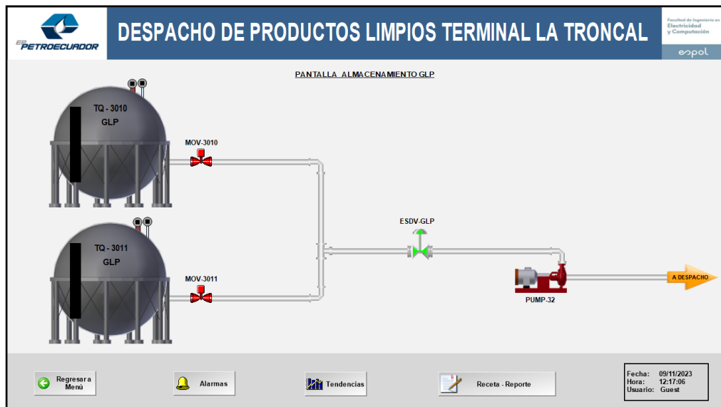
Figura 19. Pantalla Almacenamiento GLP
