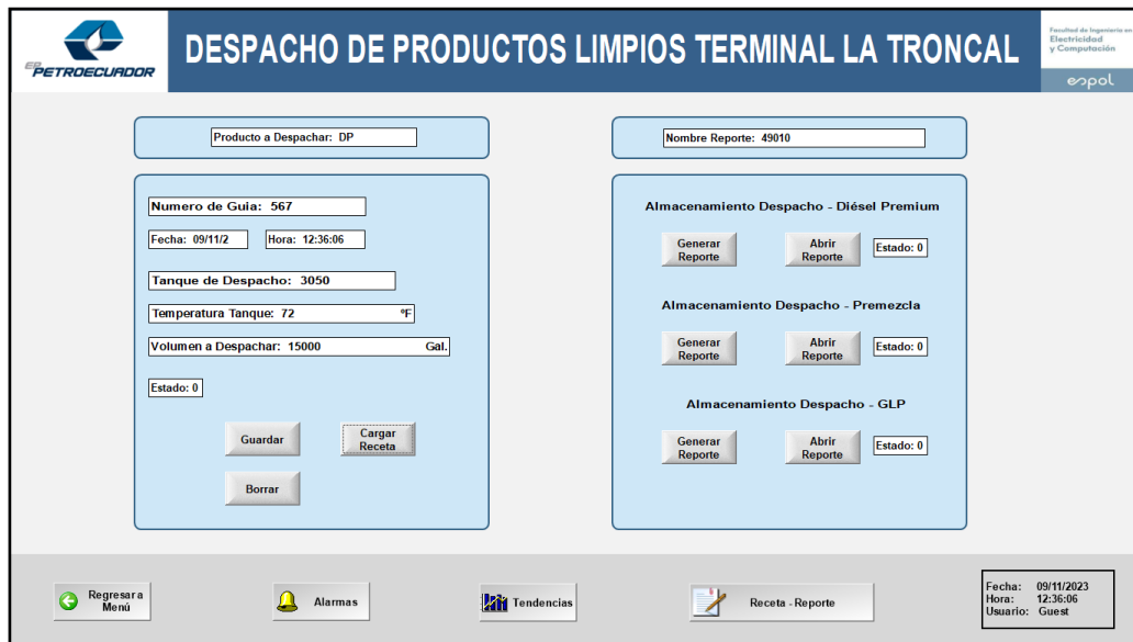
Figura 24. Pantalla de ingreso de los datos de las guías de despacho
