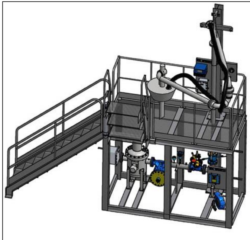
Figura 8. Diagrama Integral Islas de carga Terminal La Troncal
