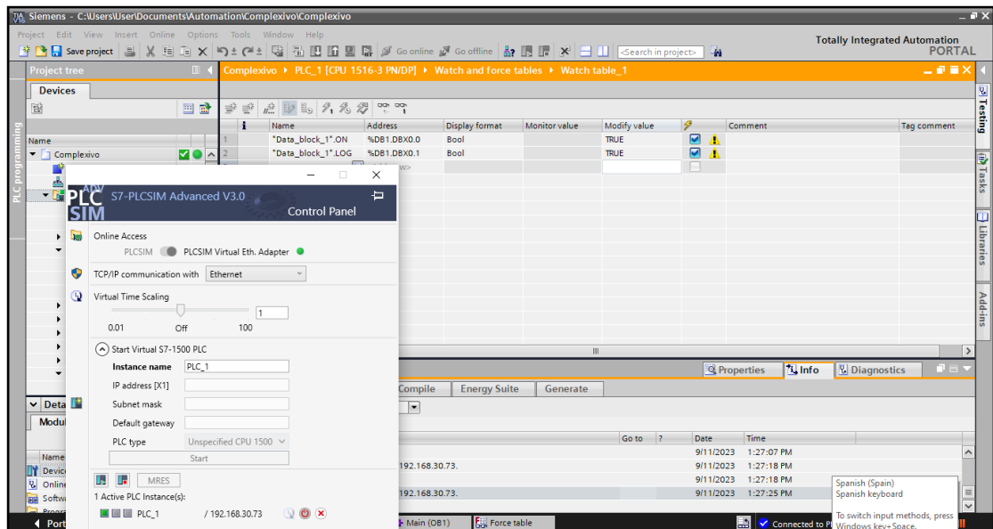
Figura 26. Simulación del PLC S7-1500 en TIA Portal
