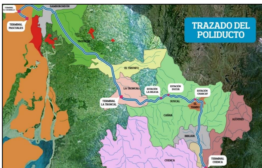
Figura 1. Trazado del Poliducto y Ubicación del Terminal La Troncal.
