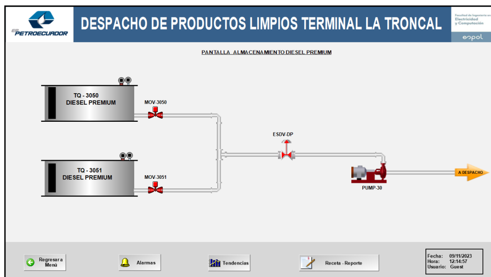
Figura 15. Pantalla Almacenamiento Diesel Premium
