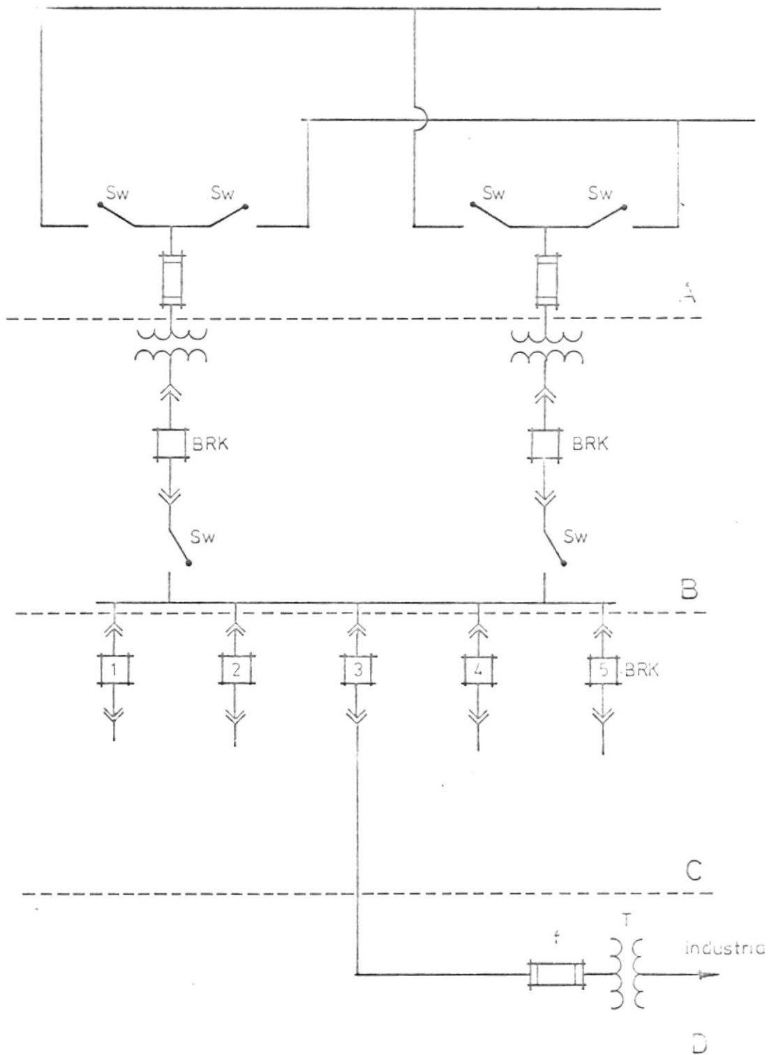
fig. 7-1 Esquema de proteccion del sistema.
