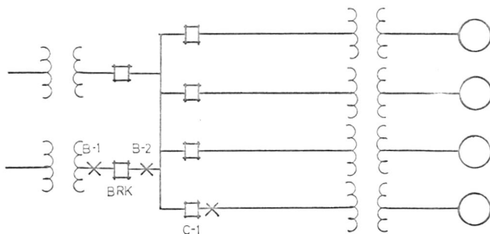
fig. 7-3 Diagrama unifilar del sistema
