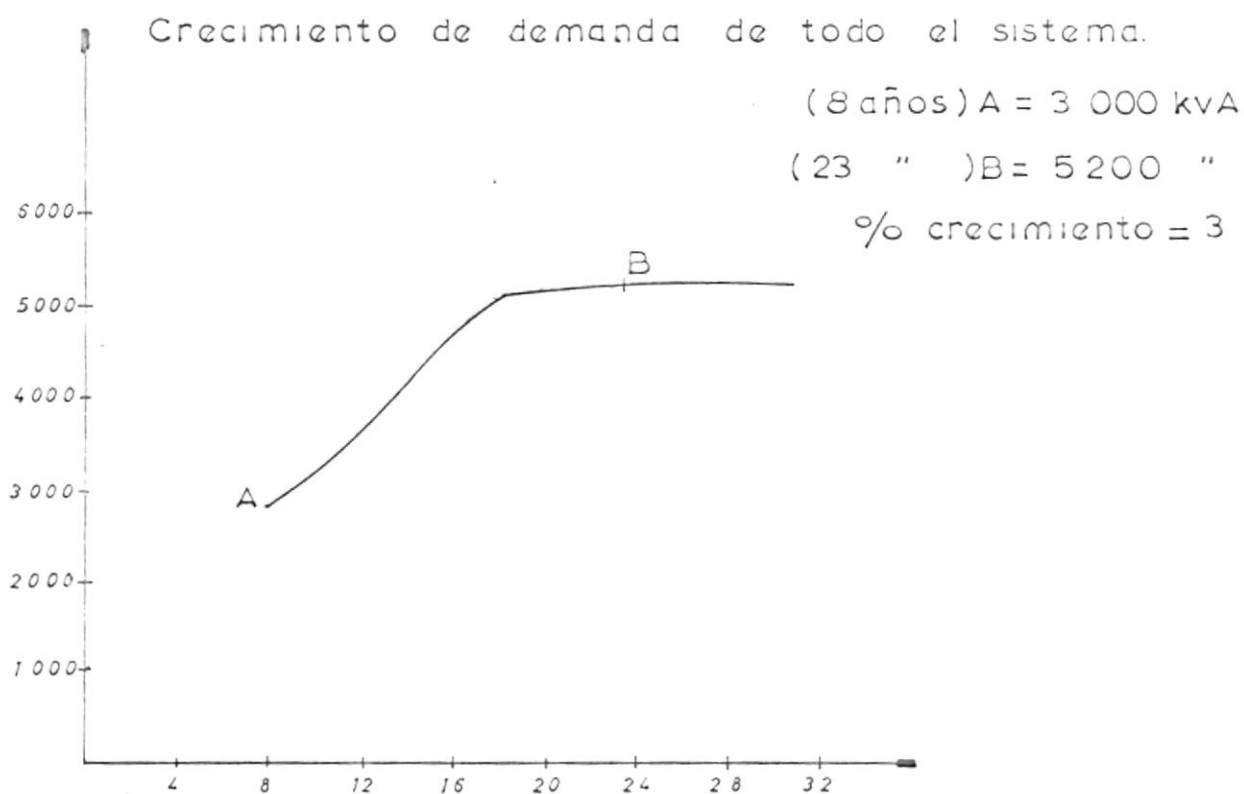
fig. 3-1 Curva de crecimiento
