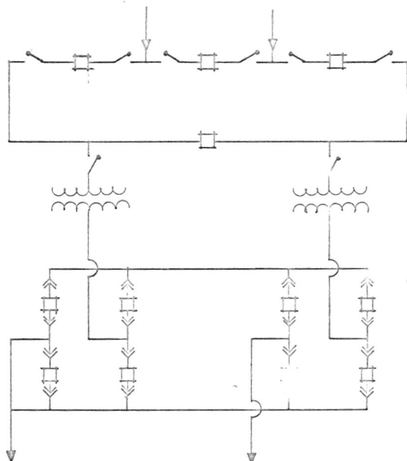
fig. 6-7 Subestaciones con arreglos especiales en las barras.
