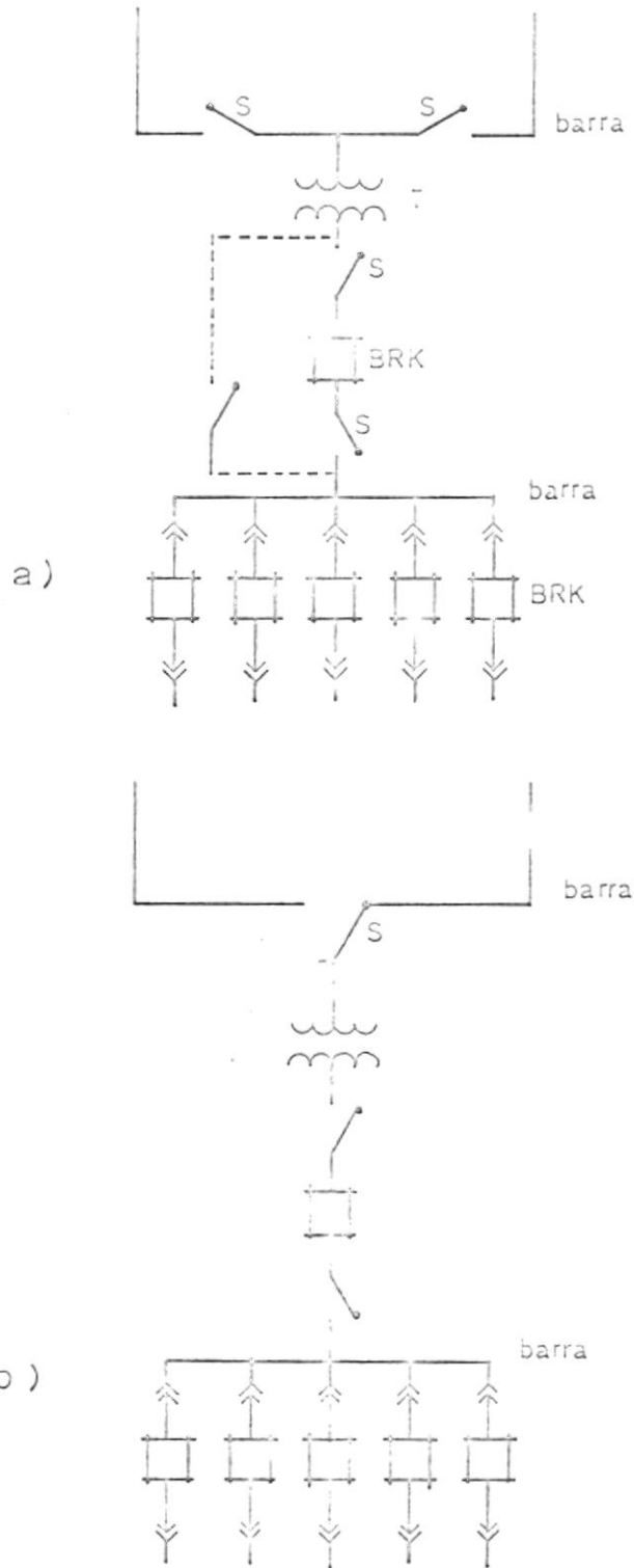
fig. 6-2 Subestación con alimentación alternativa.
