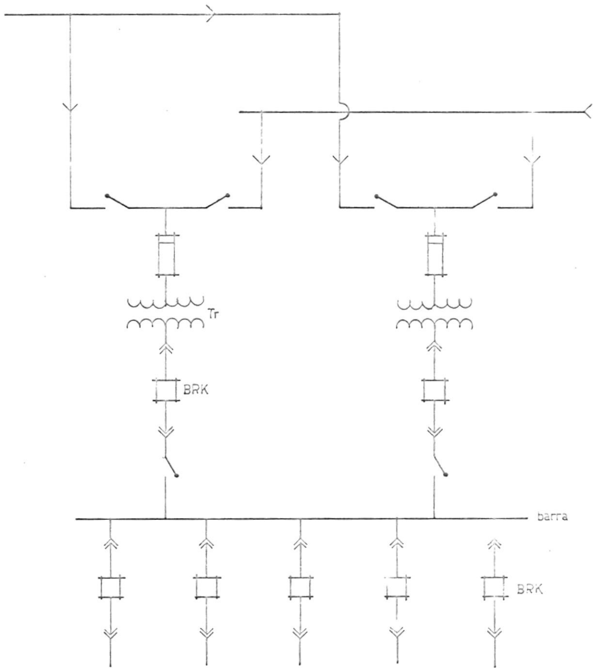
fig. 6-8 Subestación seleccionada
