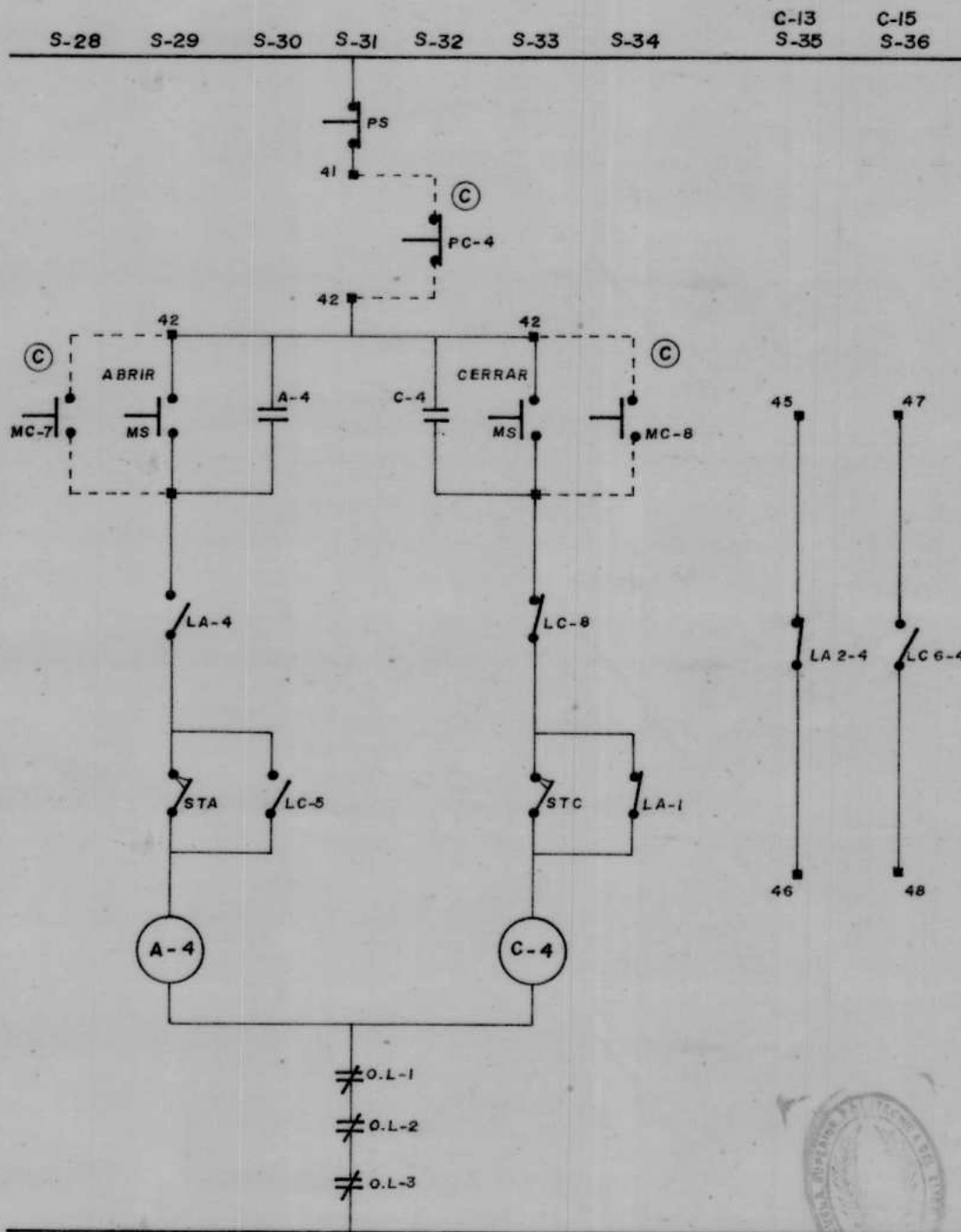
DIAGRAMA N° 4.2 EQUIPO EN SITIO PLANO N° 4/9 VALVULA MOTORIZADA VM-4
