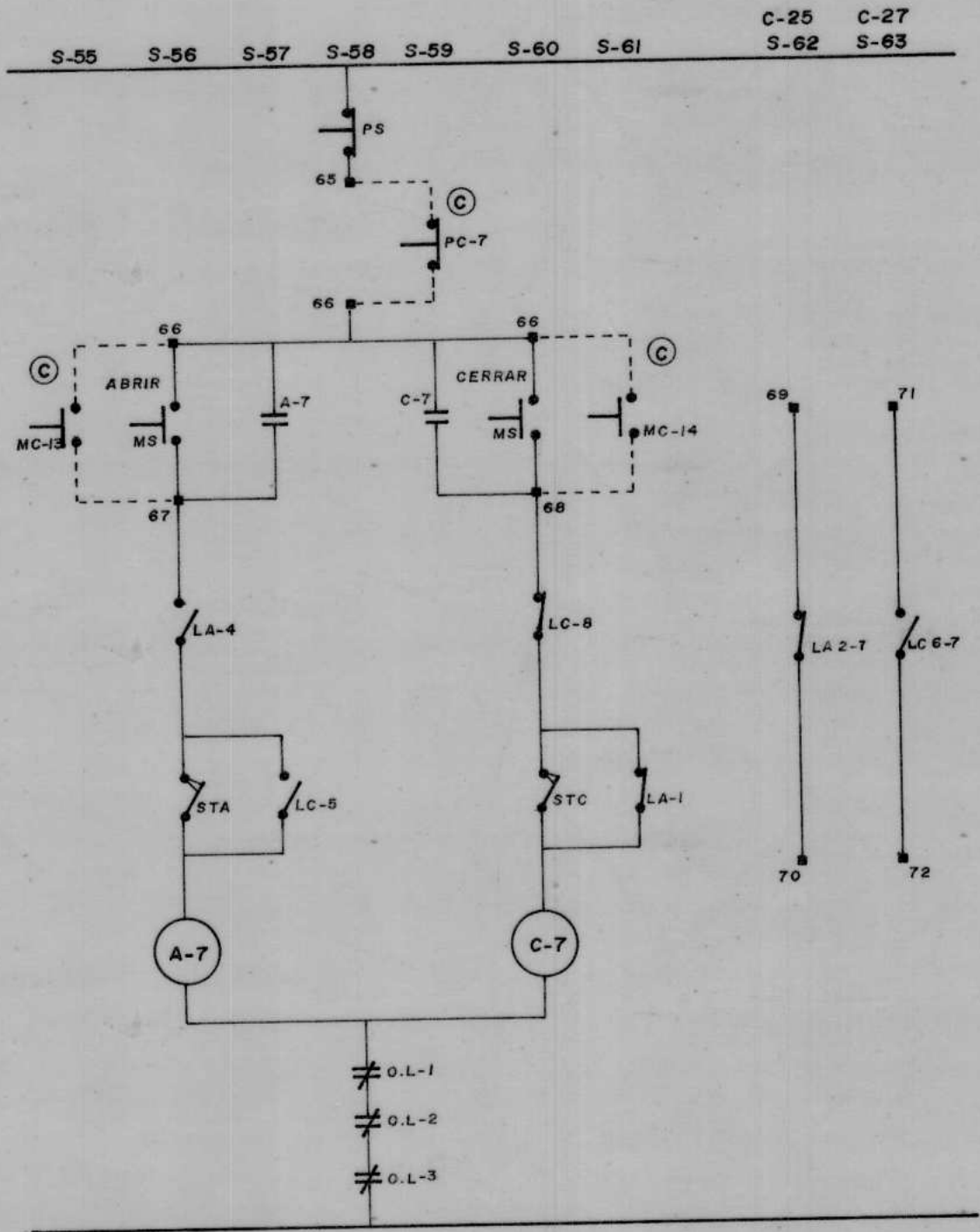
DIAGRAMA N° 4.2 EQUIPO EN SITIO PLANO N° 7/9 VALVULA MOTORIZADA VM-7
