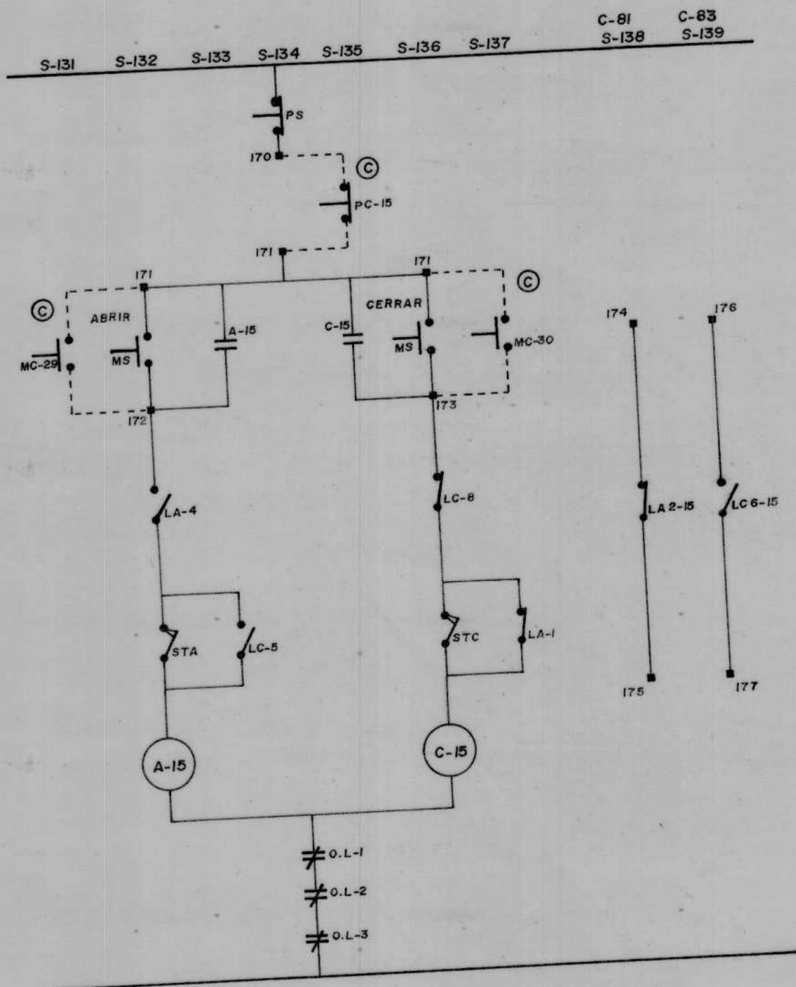
DIAGRAMA N° 4.5 EQUIPO EN SITIO PLANO N° 15/15 VALVULA MOTORIZADA VM-15
