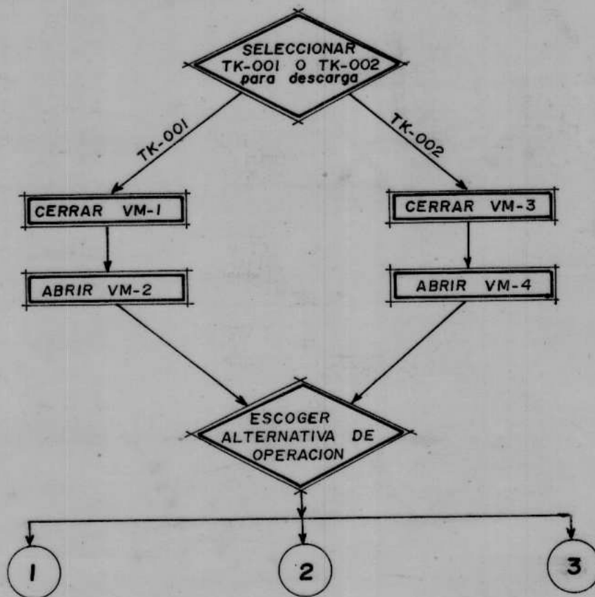
FIGURA N° 4.4 SECUENCIA DE OPERACION DEL TERMINAL DEL SALITRAL
