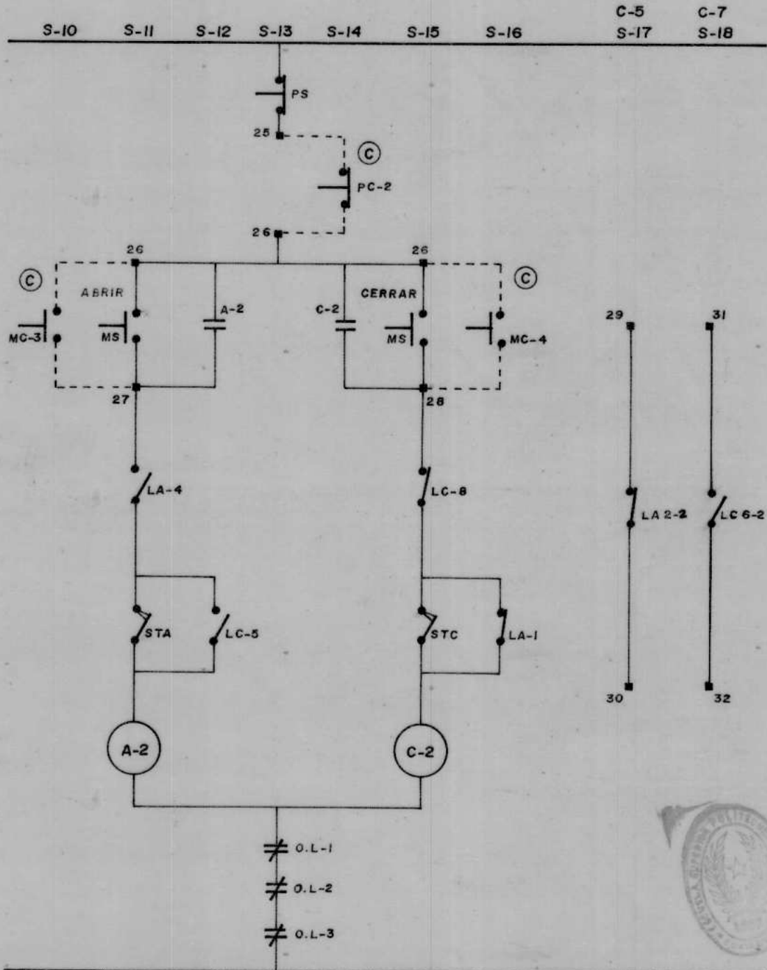
DIAGRAMA N° 4.2 EQUIPO EN SITIO PLANO N° 2/9 VALVULA MOTORIZADA VM-2
