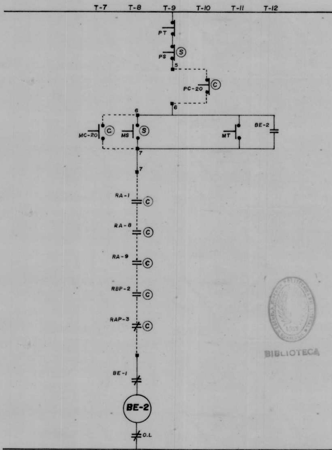
DIAGRAMA N° 4.4 TABLERO EN SUB-ESTACION PLANO N° 2/4 BOMBA DE ENGRANAJES BE-02
