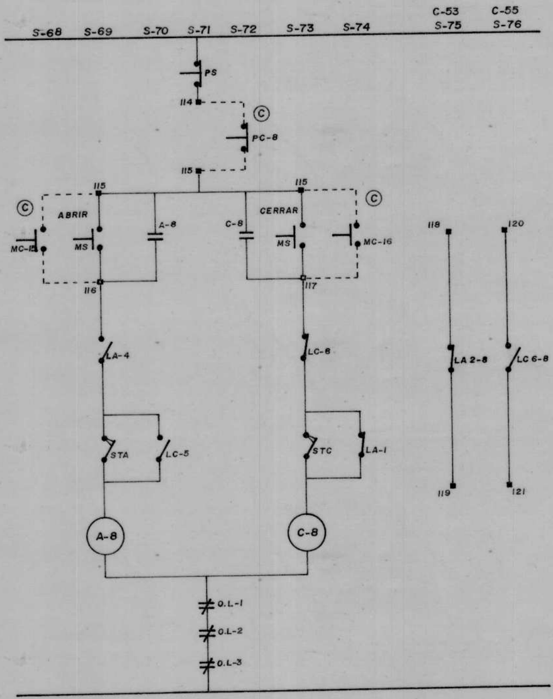
DIAGRAMA N° 4.5 EQUIPO EN SITIO PLANO N° 8/15 VALVULA MOTORIZADA VM-8
