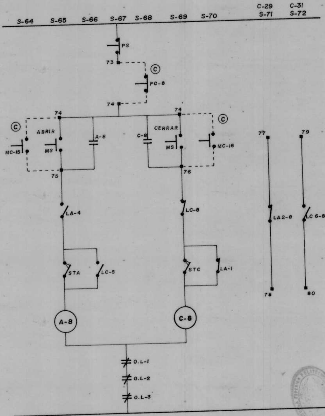
DIAGRAMA N° 4.2 EQUIPO EN SITIO PLANO N° 8/9 VALVULA MOTORIZADA VM-8
