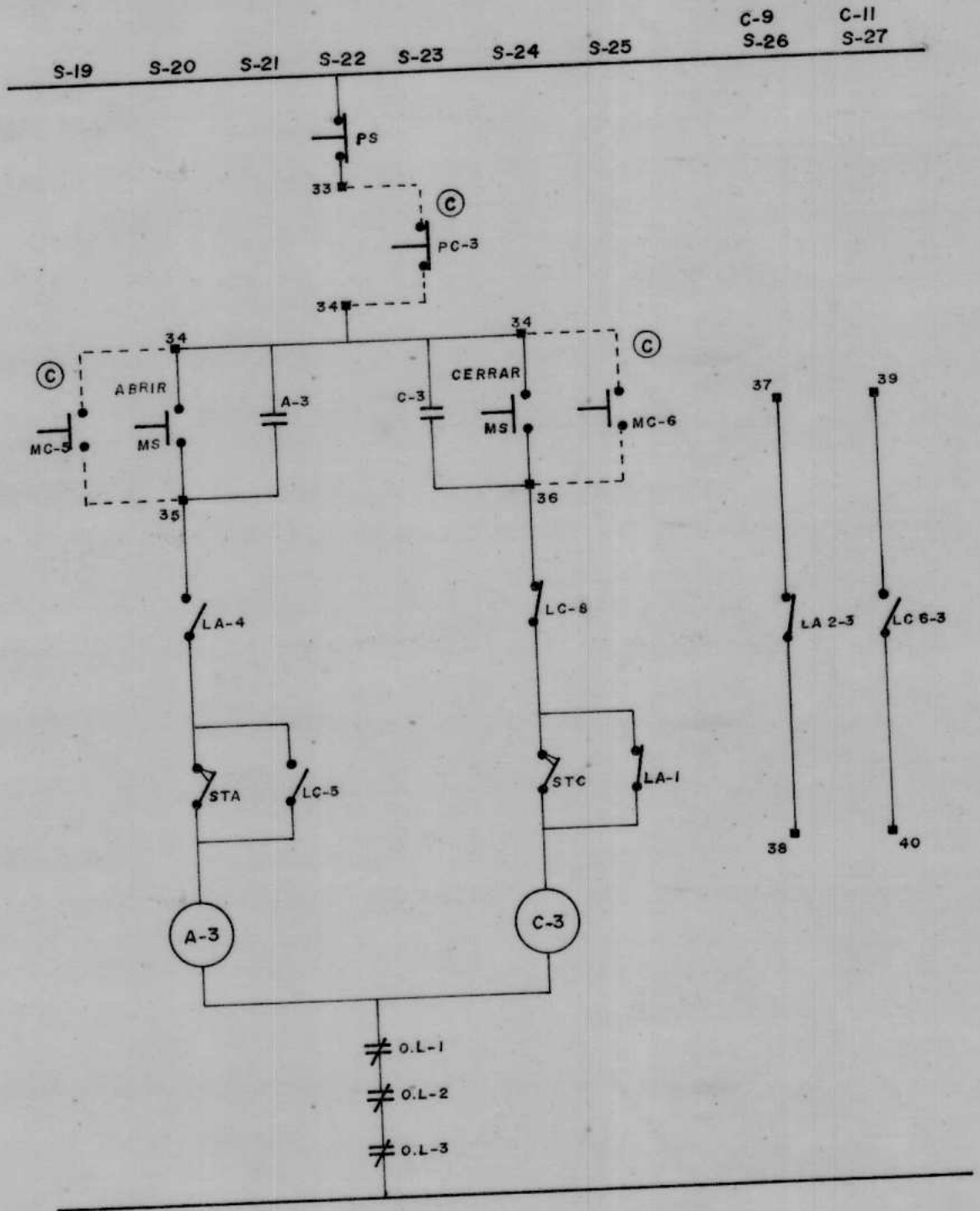
DIAGRAMA N° 4.2 EQUIPO EN SITIO PLANO N° 3/9 VALVULA MOTORIZADA VM-3
