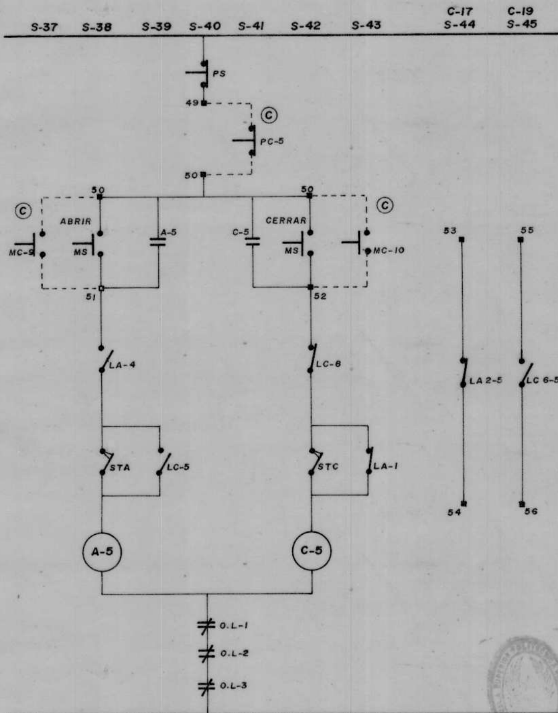
DIAGRAMA N° 4.2 EQUIPO EN SITIO PLANO N° 5/9 VALVULA MOTORIZADA VM-5
