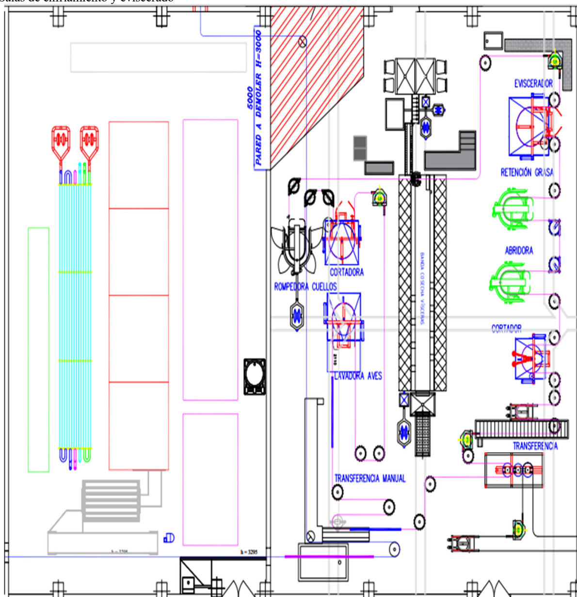
Figura 38 Salas de enfriamiento y eviscerado
