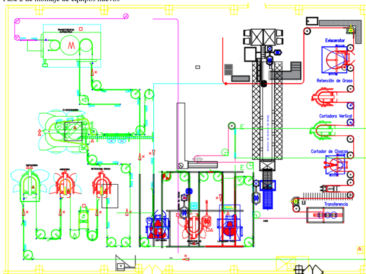
Figura 40 Fase 2 de montaje de equipos nuevos
