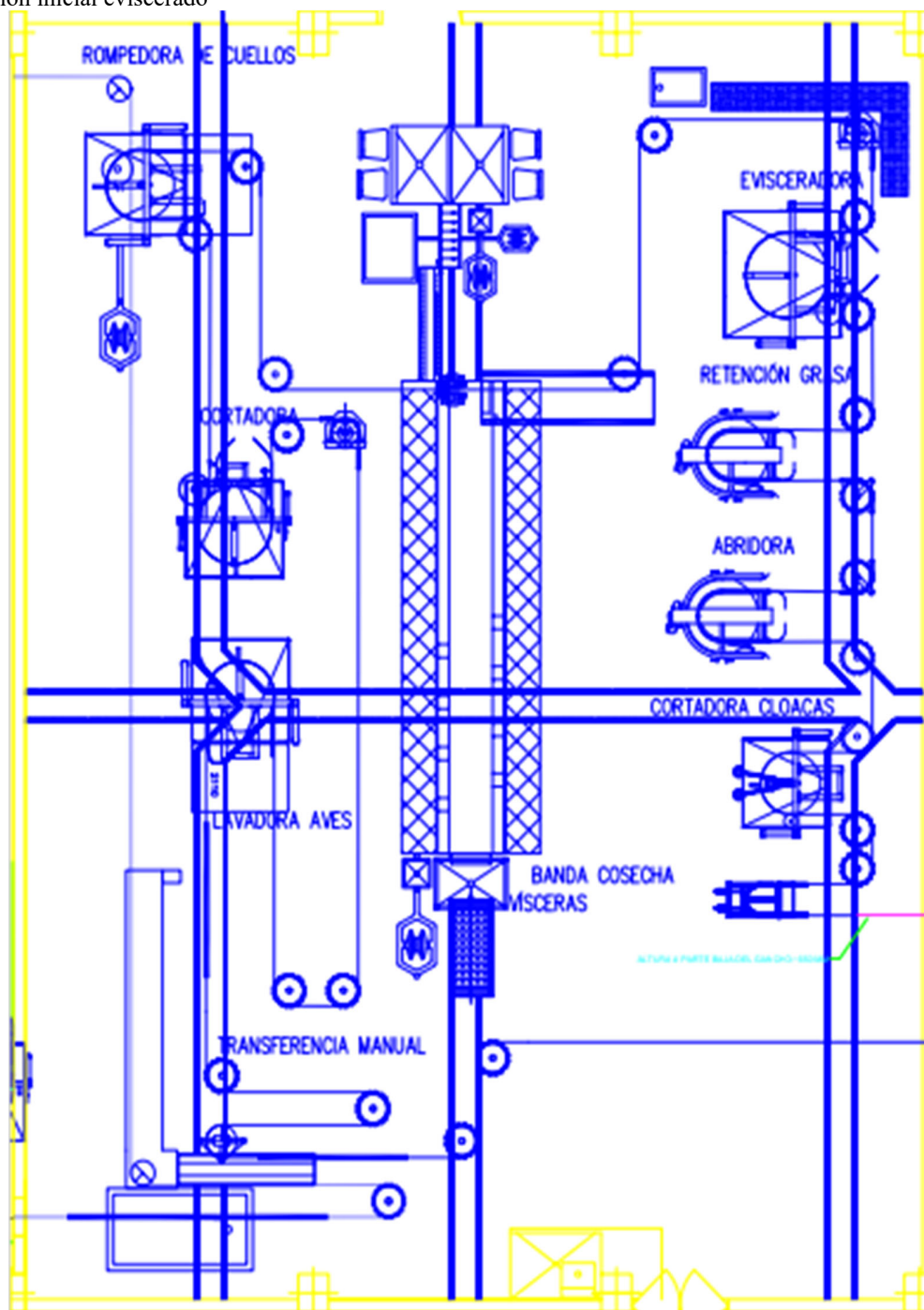
Figura 37 Implantación inicial eviscerado
