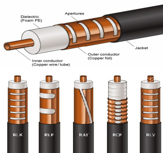
Figura 2.8 Cables radiantes
