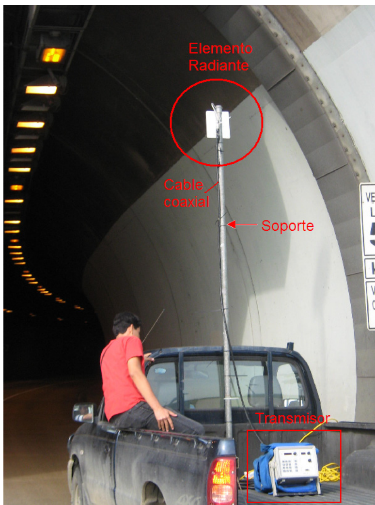
Figura 3.15 Equipamiento transmisor
