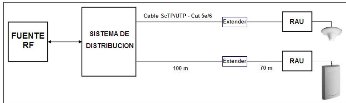
Figura 3.7 Esquema general del sistema
