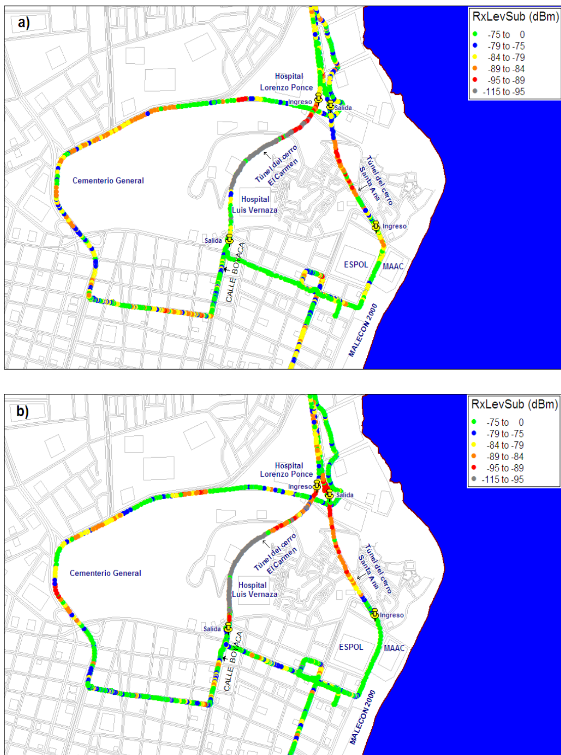
Figura 3.6 Niveles de señal en los exteriores del túnel del cerro El Carmen. a) Movistar y Alegre b) Porta
