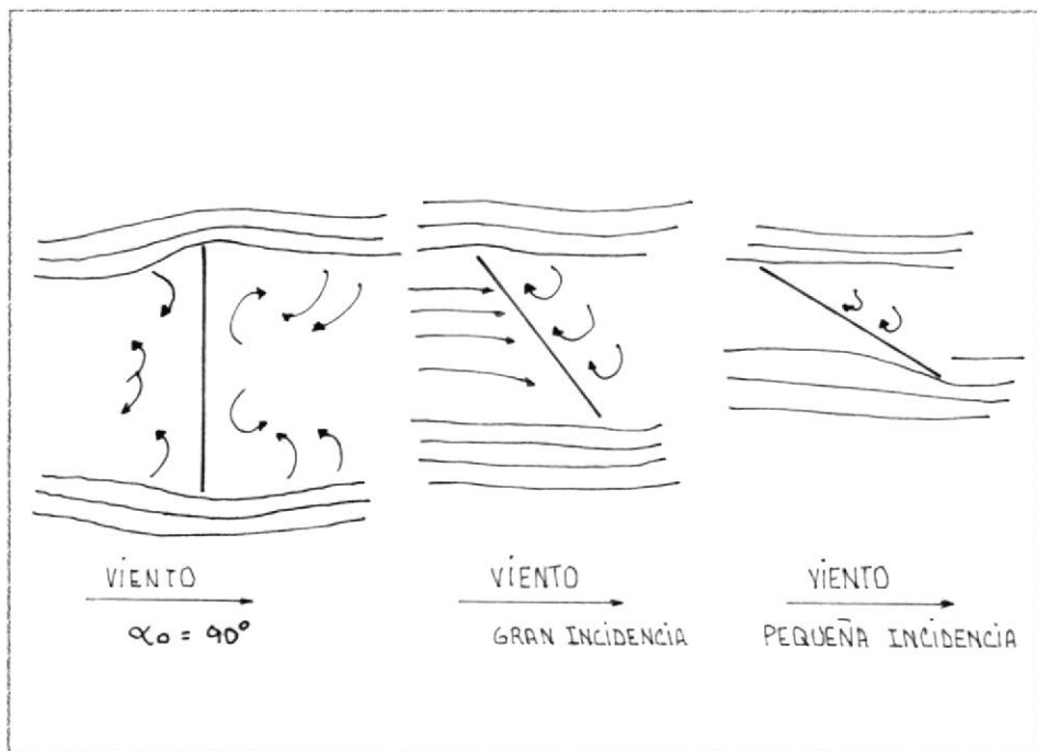
Fig.Nº5.9 ACCION DEL VIENTO SOBRE UNA PLACA PLANA Ref (6).
