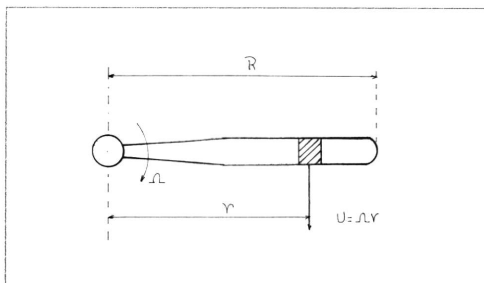
Fig.Nº5.6 DEFINICION DE LA RELACION DE VELOCIDADES Ref (15).
