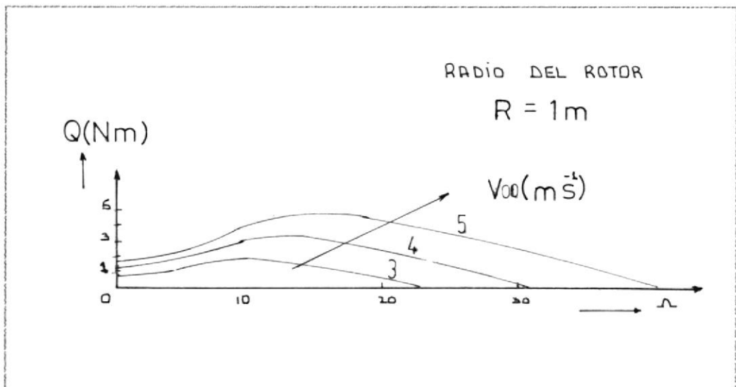
Fig.Nº5.18 TORQUE CARACTERISTICO DE UN MOLINO DE VIENTO DE ALTA VELOCIDAD Ref (15).
