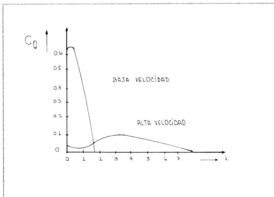
Fig.Nº5.7 C_D - CARACTERISTICOS DE MOLINOS DE EJE HORIZONTAL Ref (15).
