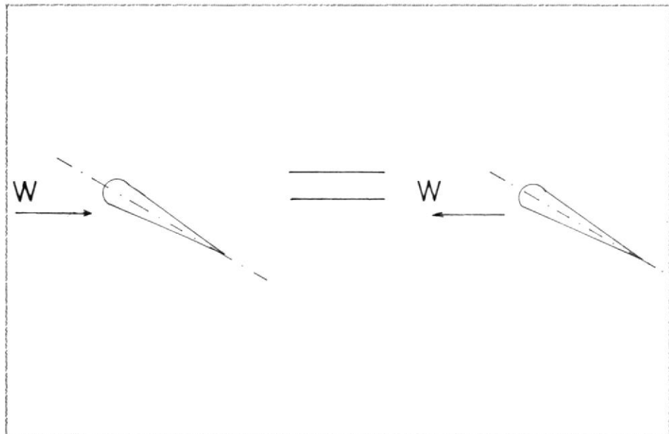
Fig. Nº5.14 VELOCIDAD RELATIVA EN UN ALABE Ref (15).
