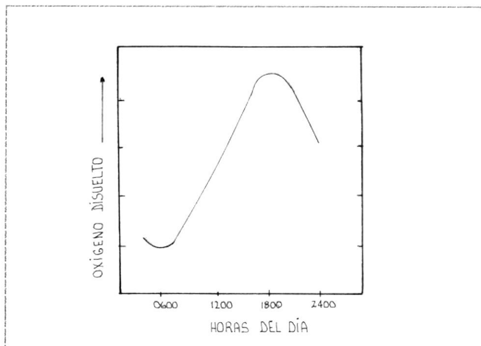
Fig.Nº2.1 FLUCTUACIONES TÍPICAS DE OD EN UN ESTANQUE CON ELEVADAS CANTIDADES DE FOTOSÍNTESIS Y RESPIRACIÓN Ref (ii).
