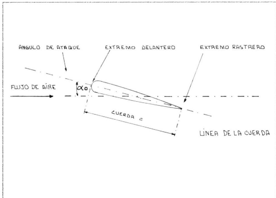
Fig. Nº5.13 CUERDA DEL PERFIL Y ANGULO DE ATAQUE Ref (15).
