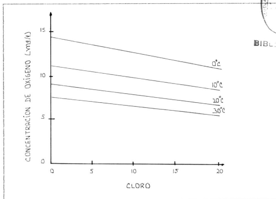
Fig. N.º 2.4 CONCENTRACION DE SATURACION DE OXIGENO EN AGUA A DIFERENTES TEMPERATURAS Y GRADOS DE SALINIDAD Ref (19).
