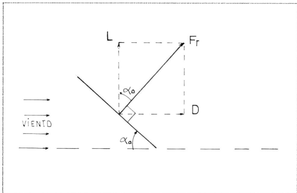
Fig.Nº5.10 DESCOMPOSICION DE LA FUERZA RESULTANTE Ref (6).
