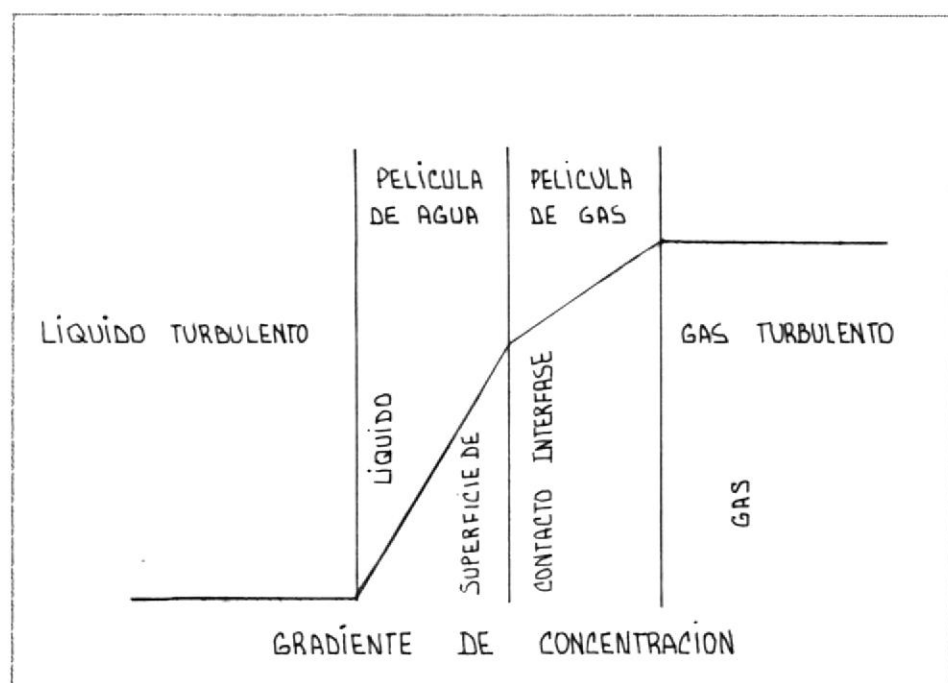
Fig.Nº3.3 INTERCAMBIO DE GASES A TRAVES DE DOS PELICULAS ESTACIONARIAS Ref(18).
