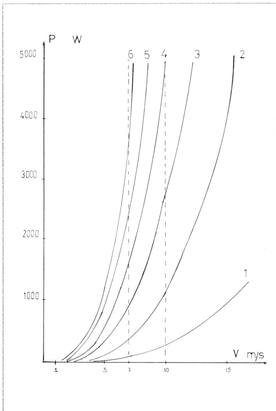
Fig. Nº5.5 LIMITES DE BETZ PARA DIFERENTES DIÁMETROS DE ROTOR P = 0.29 D^2 * v^3 Ref (6).
