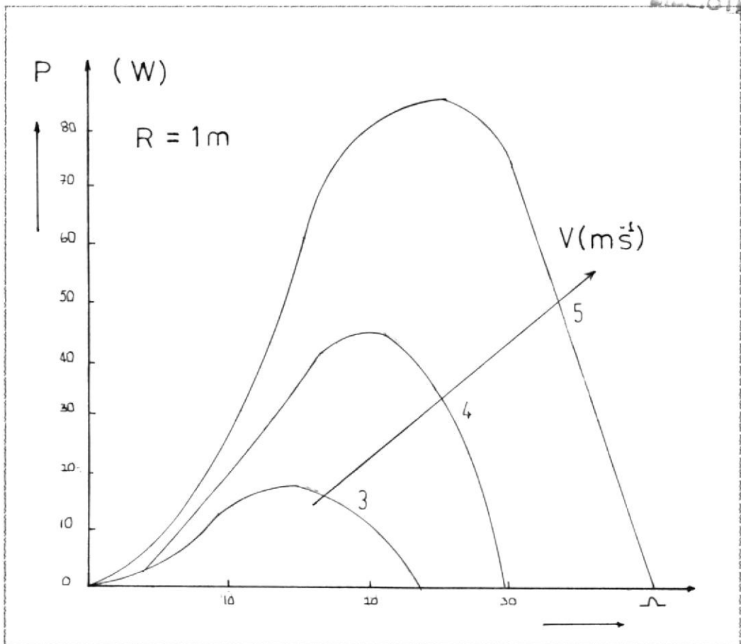
Fig. Nº5.20 POTENCIA CARACTERISTICA DE UN MOLINO DE VIENTO DE ALTA VELOCIDAD Ref (15).
