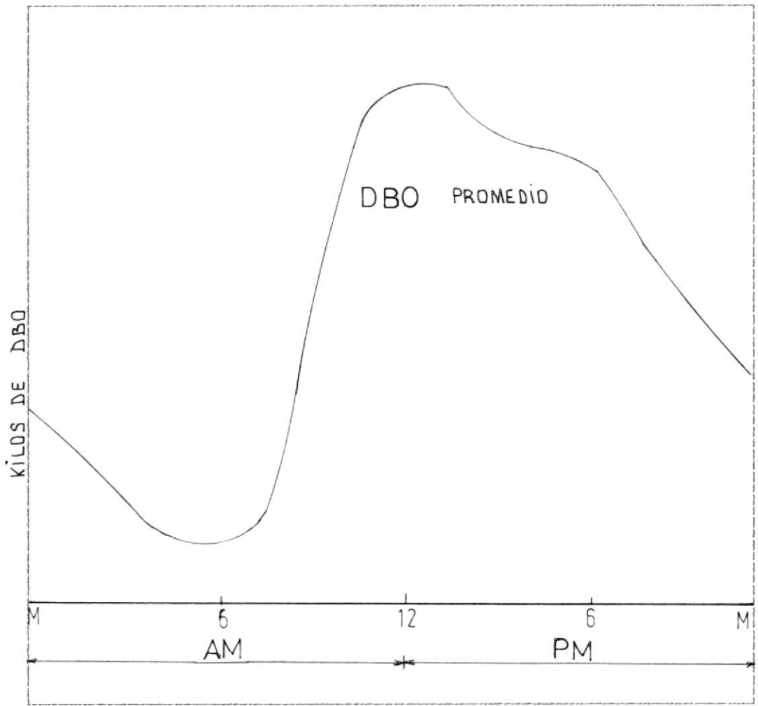
Fig. Nº2.5 VARIACIONES DEL DBO PROMEDIO DURANTE EL DIA EN UNA LAGUNA DE OXIDACION Ref (7).
