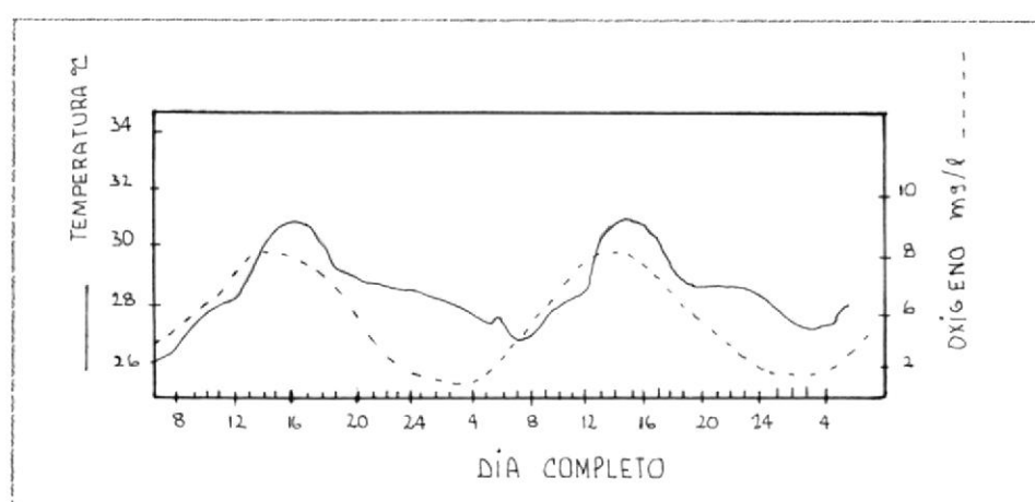
Fig.Nº2.2 EJEMPLO DE VARIACIONES DIARIAS DE TEMPERATURA Y OXIGENO DISUELTO Ref (ii).
