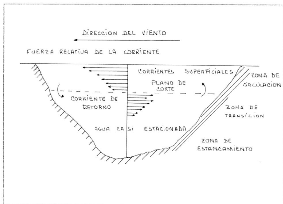
Fig.Nº4.1 DIRECCION Y VELOCIDAD HORIZONTAL RELATIVA DE LAS CORRIENTES QUE PRODUCE EL VIENTO EN UN LAGO O ALMACENAMIENTO (IDEALIZADO) Ref (8).
