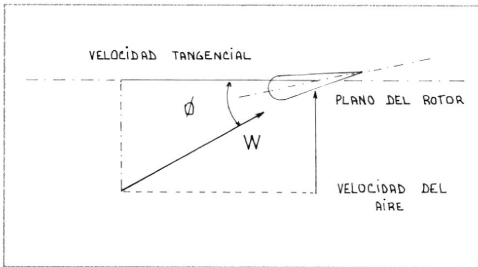
Fig.Nº5.15 VELOCIDAD RELATIVA EN EL ÁLABE DE UN ROTOR Ref (15).
