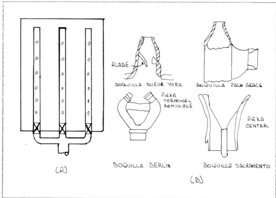
Fig.Nº4.3 AERADOR FOR ASPERSION Y BOQUILLAS A) AERADOR DOTADO DE BOQUILLAS B) BO- QUILLAS PARA AERADORES Ref (8).
