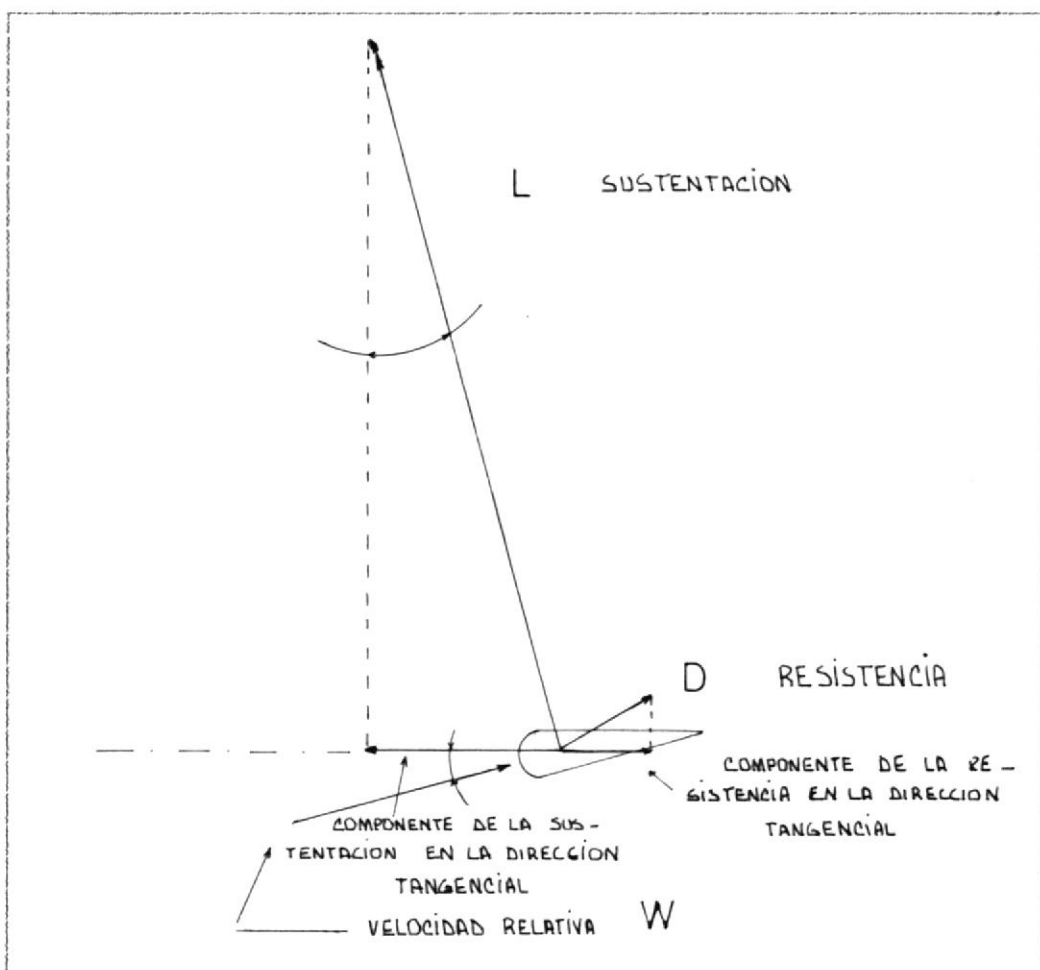
Fig.Nº5.16 COMPONENTES DE SUS-TENTACION Y RESISTENCIA SEGUN EL PLANO DE ROTACION Ref (15).
