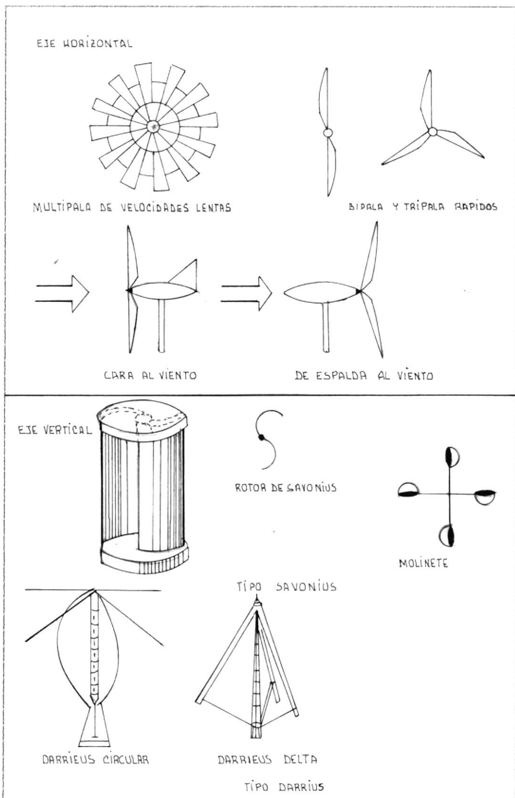
Fig. Nº5.4 CLASIFICACION DE LOS ARTEFACTOS EOLICOS. Ref (6).
