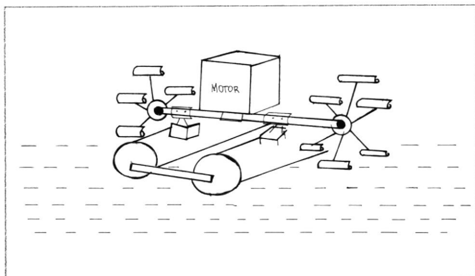
Fig.Nº4.8 ESQUEMA DE UN AERADOR FLOTANTE Ref (11).
