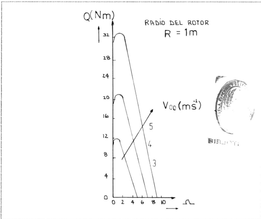
Fig.Nº5.17 TORQUE CARACTERISTICO DE UN MOLINO DE VIENTO DE BAJA VELOCIDAD Ref (15).
