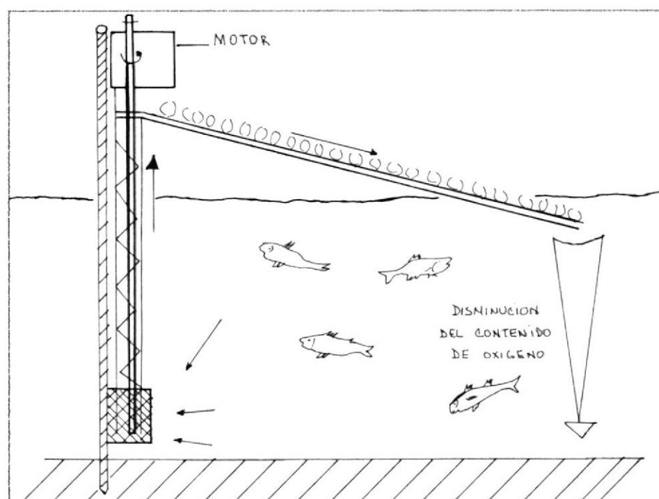
Fig.Nº4.7 ESQUEMA DE UN AERADOR DE FONDO PARA ESTANQUE Ref(11).
