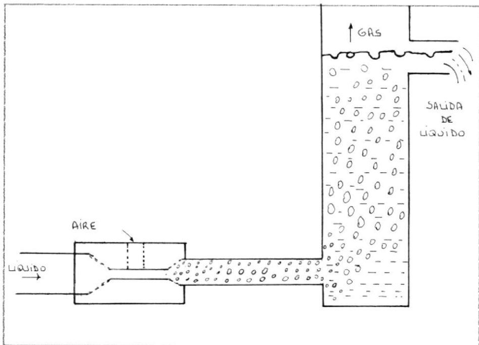
Fig.N°4.6 AERADOR TIPO VENTURI Ref (19).
