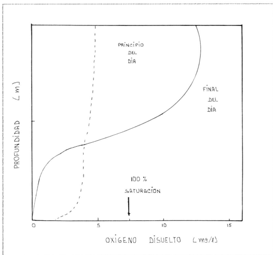
Fig.Nº2.3 PERFILES TÍPICOS DE OXÍGENO DISUELTU EN AGUA AL PRINCIPIO (----) Y AL FINAL (—) DEL DÍA EN UN ESTANQUE SIN AGITACION Ref (11).
