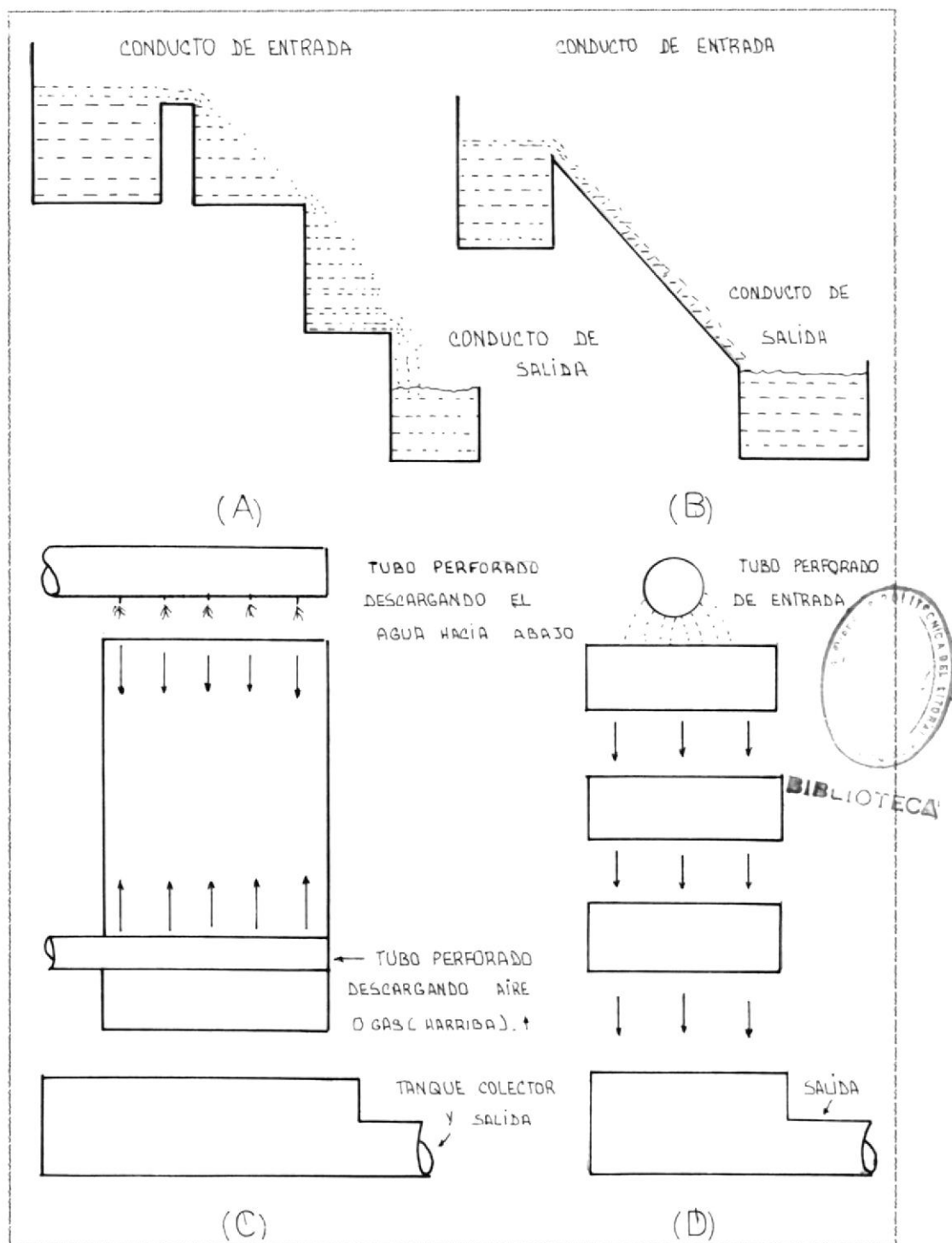
Fig. Nº4.2 AERADORES POR GRAVEDAD A) DE CÁSCADA; B) DE PLANO INCLINADO C) DE TORRE CON FLUJO A CONTRACORRIENTE DE AIRE (GAS) Y AGUA; D) COLUMNA DE CHAROLAS PERFORADAS CONTENIENDO POSIBLEMENTE MEDIO DE CONTACTO Ref (8).
