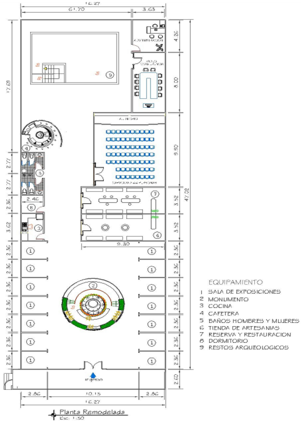
Plano de la nueva propuesta
