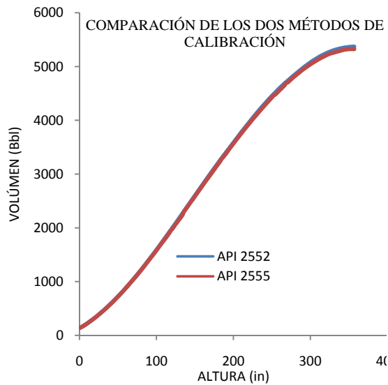
Figura 9. Comparación de los dos métodos de calibración
