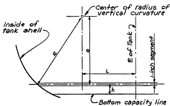
Figura 5. Calculo de los radios interiores por cada pulgada
