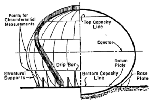
Figura 2. Tanque esferoidal
