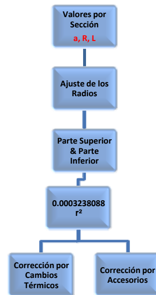
Figura 7. Procedimiento para la corrección de los radios interiores
