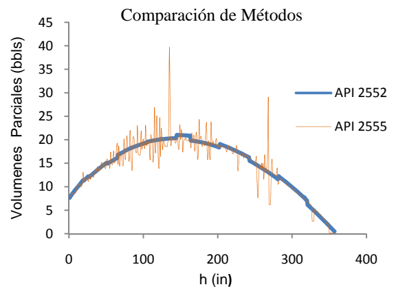
Figura 8. Gráfico comparativo de volúmenes parciales versus altura
