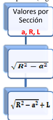
Figura 6. Procedimiento para calcular los radios interiores
