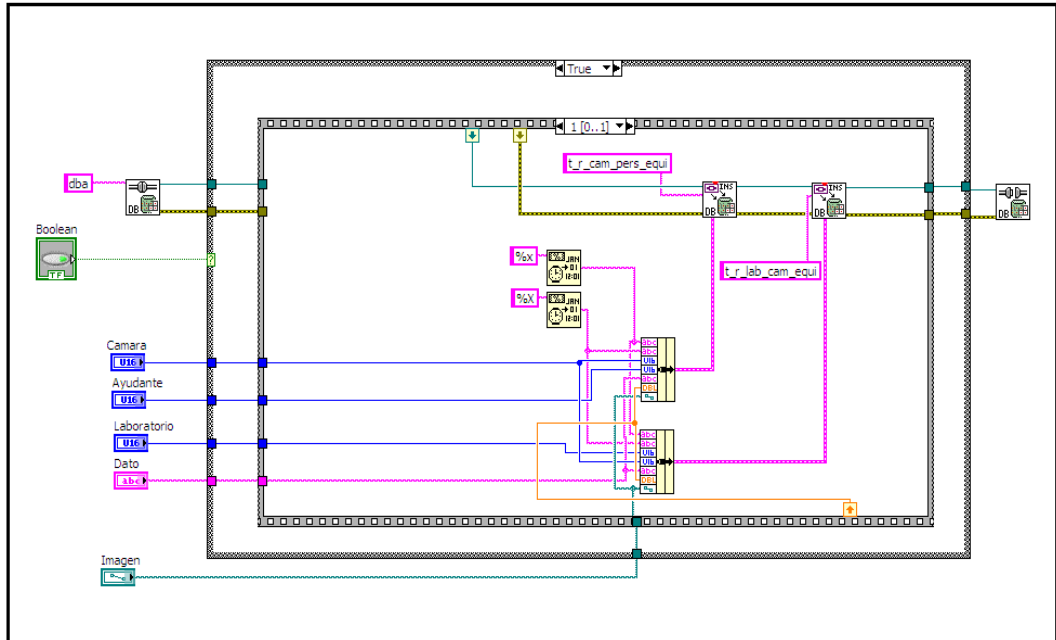
Figura 3.15 Segunda secuencia del SubVI Base de Datos.
