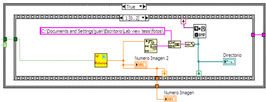
Figura 3.12 Secuencia de almacenamiento de imagen.
