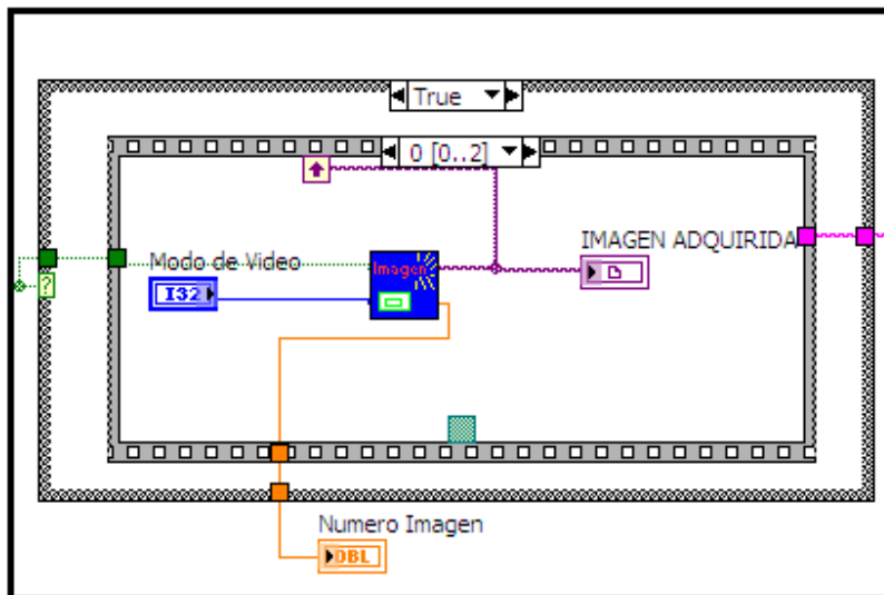
Figura 3.5 Secuencia de Manejo de Imágenes.
