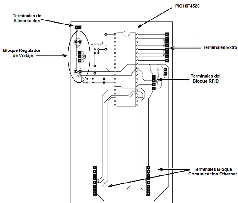
Figura 4.1 Circuito Impreso del Sistema.
