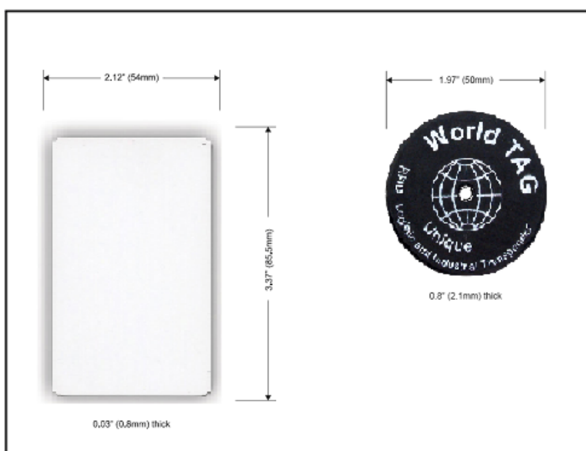
Figura 2.23 Etiquetas del Módulo RFID #28140. 11
