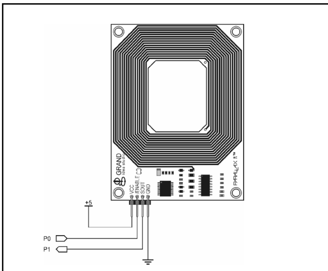
Figura 2.22 Lector RFID # 28140. 10
