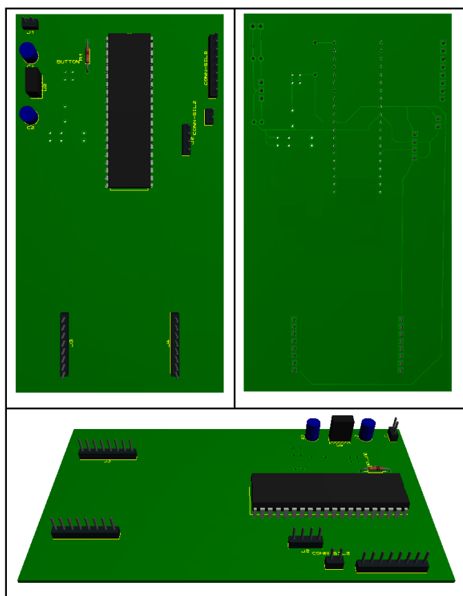
Figura 3.3 Simulación del Circuito Impreso.
