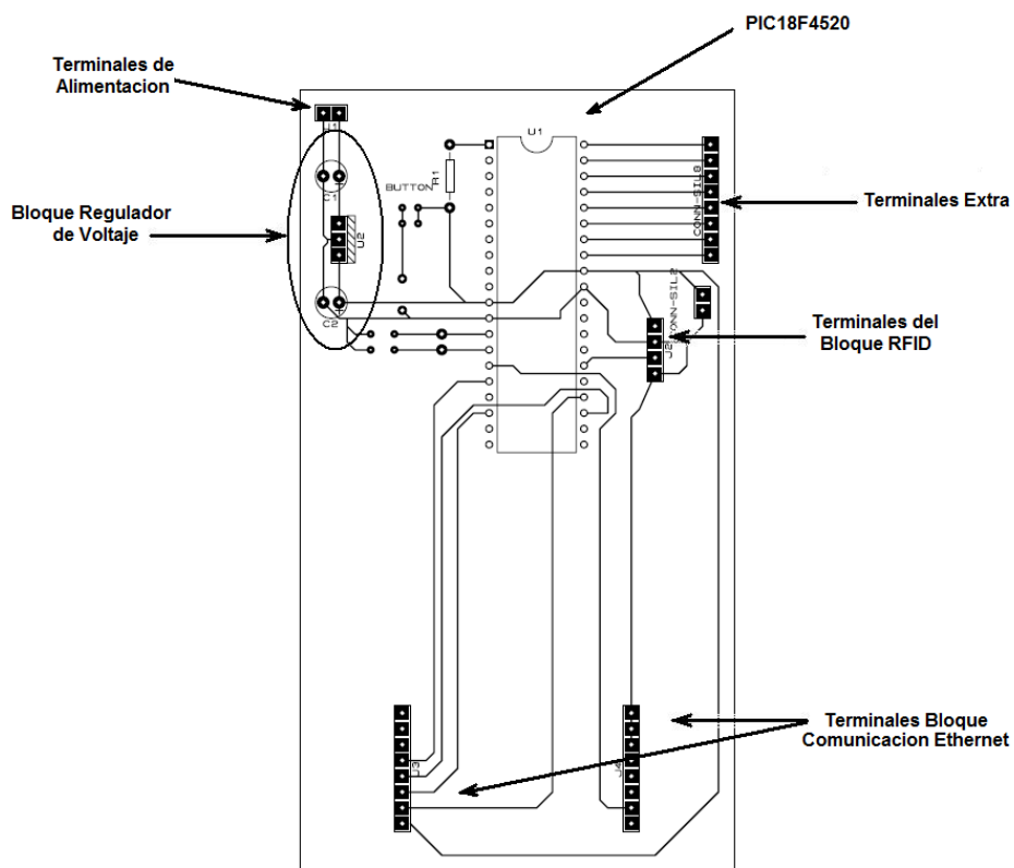
Figura 3.2 Detalle del diseño del Circuito Impreso.
