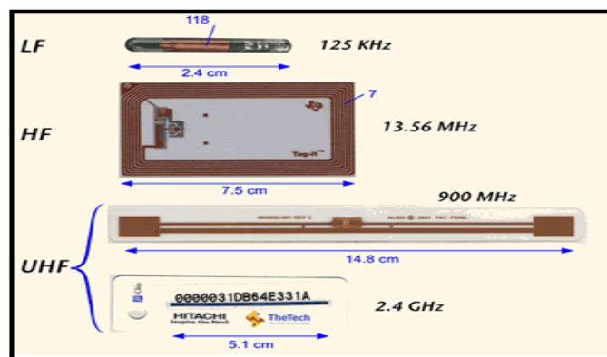
Figura 2.5 Clasificación de Sistemas RFID. 6
