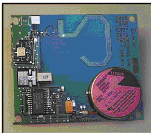
Figura 2.2 Tag Semipasivo 3 .
