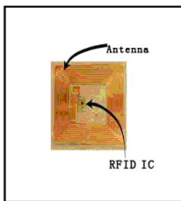
Figura 2.3 Tag Pasivo. 4
